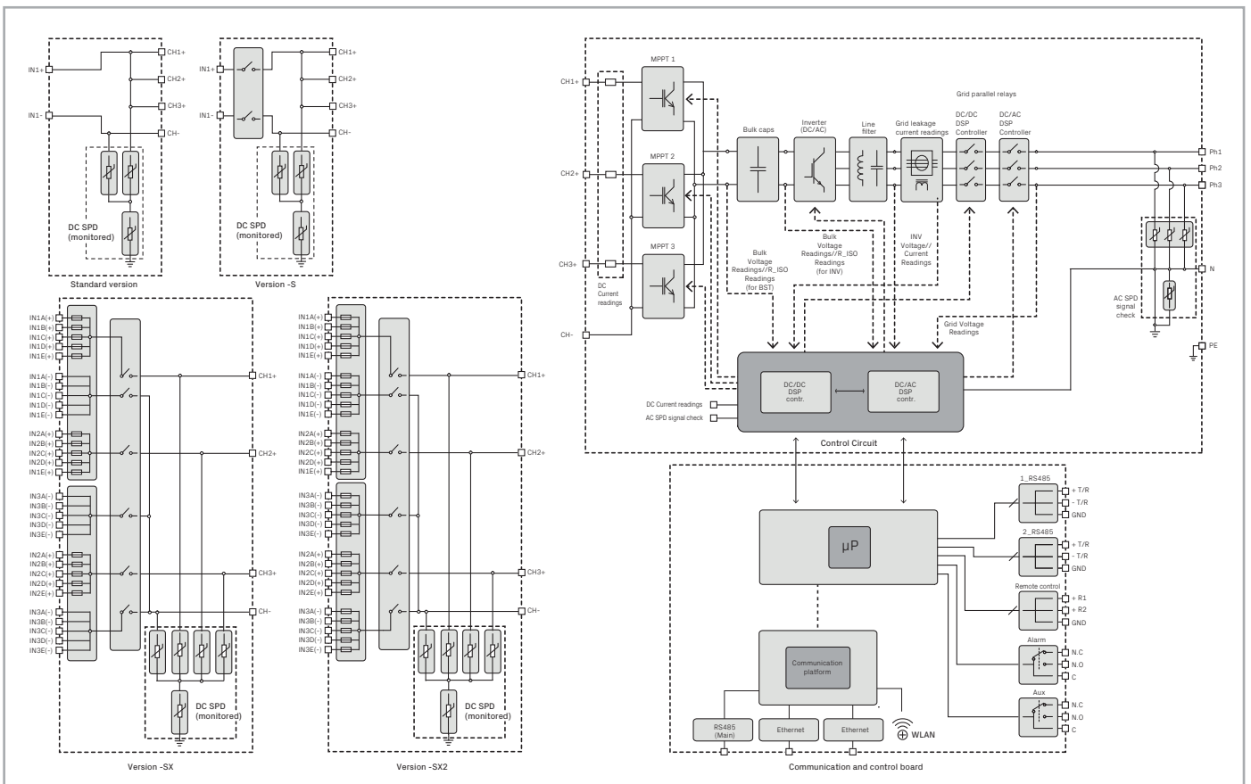
PVS-50/60-TL-String-Wechselrichter-Blockdiagramm
