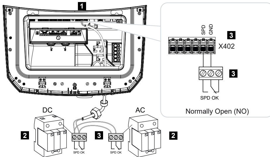
Abb. 2: Überspannungsschutz (SPD) als Schließer
