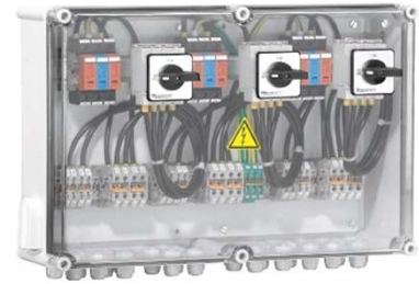
(Beispielbild, kann vom eigentlichen Produkt abweichen) (Example of Combiner Box. Picture may differ from product)
