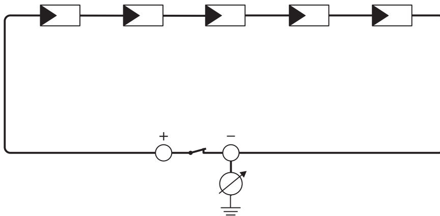
Figure 11 : Représentation schématique de la mesure
