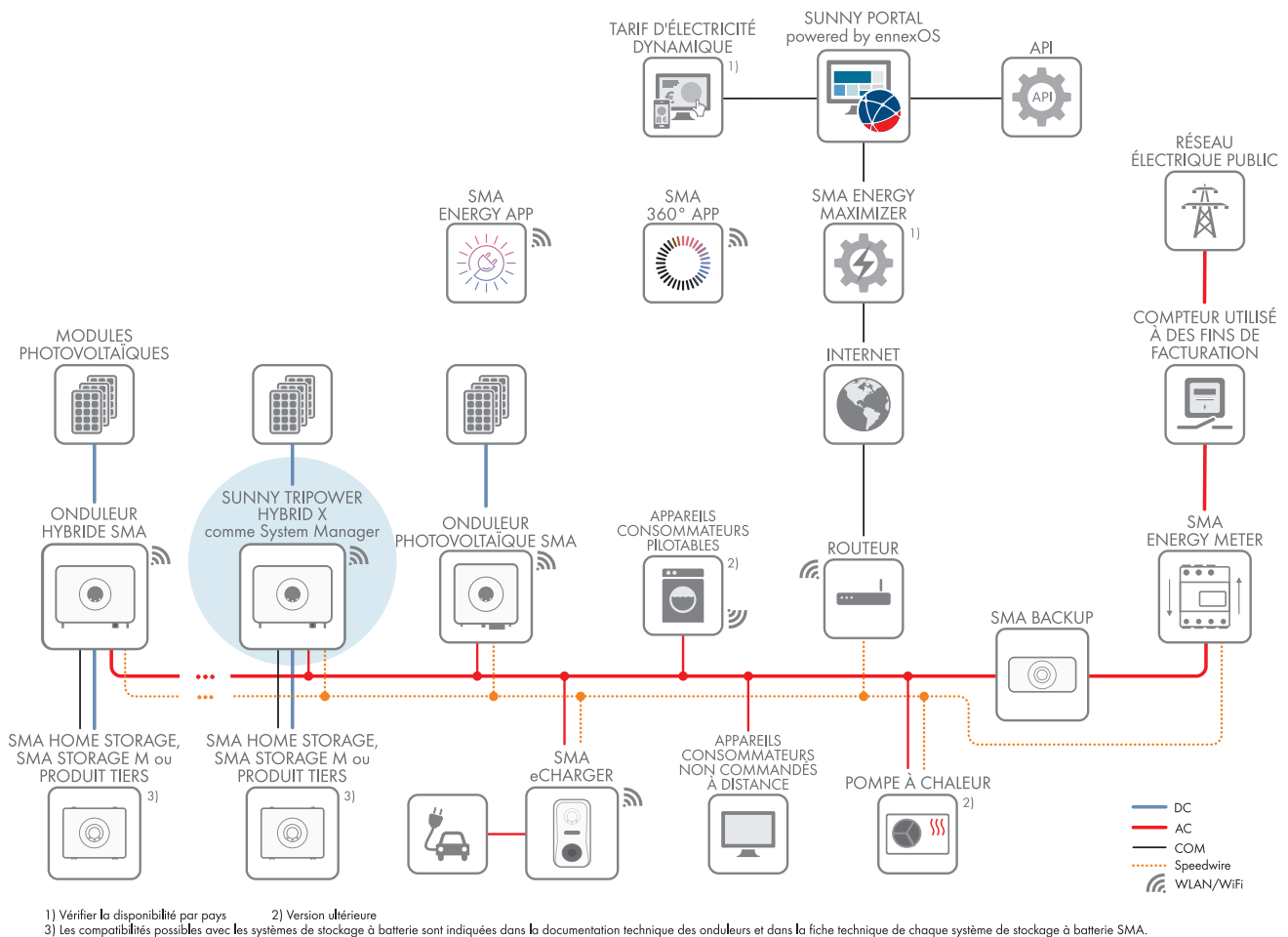
Figure 2 : Vue d'ensemble du système avec 1 Sunny Tripower Hybrid X (STPxx-70) comme System Manager.
