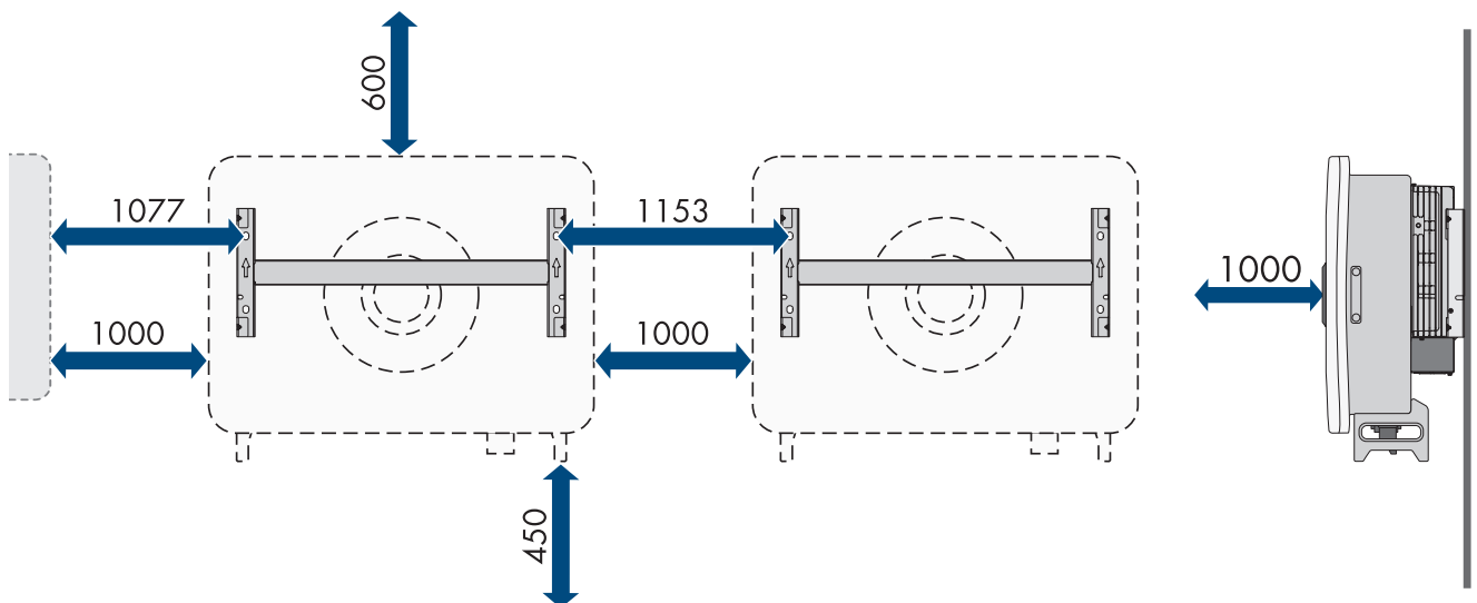
Figure 5 : Distances recommandées (dimensions en mm)
