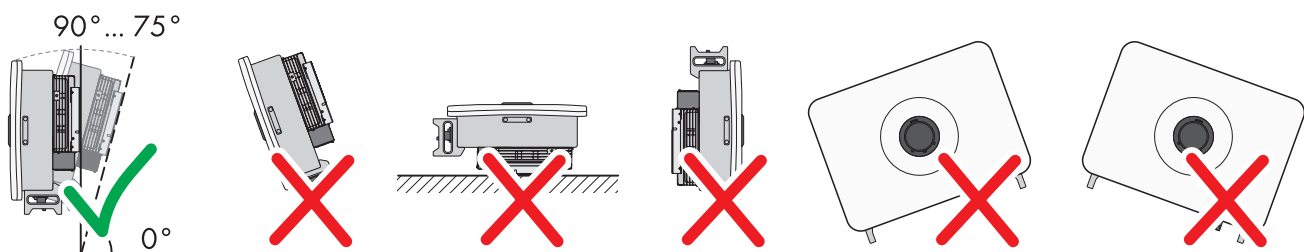
Figure 3 : Positions de montage autorisées et non autorisées
