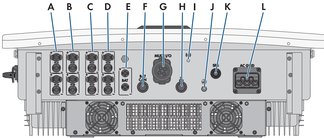
Figure 6 : Vue de dessous de l'onduleur
