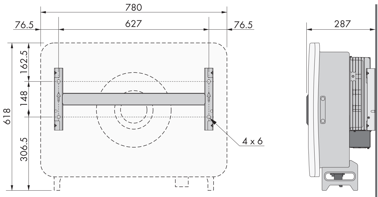
Figure 4 : Position des points de fixation (dimensions en mm)
