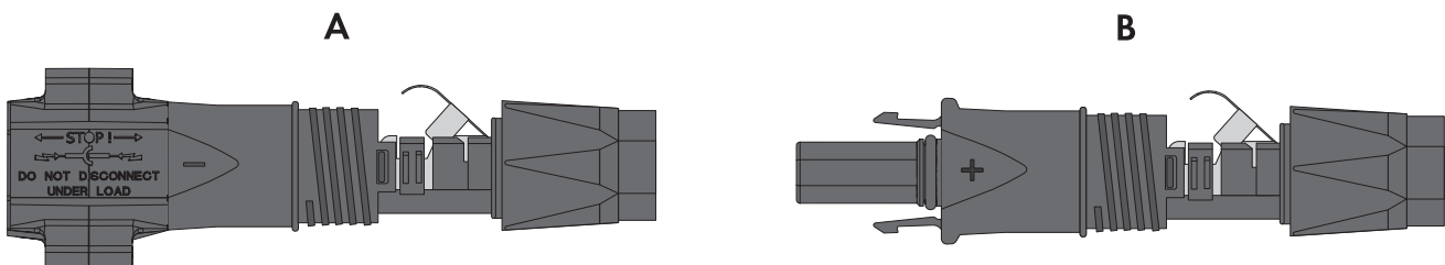
Figure 7 : Connecteur DC négatif (A) et positif (B)
