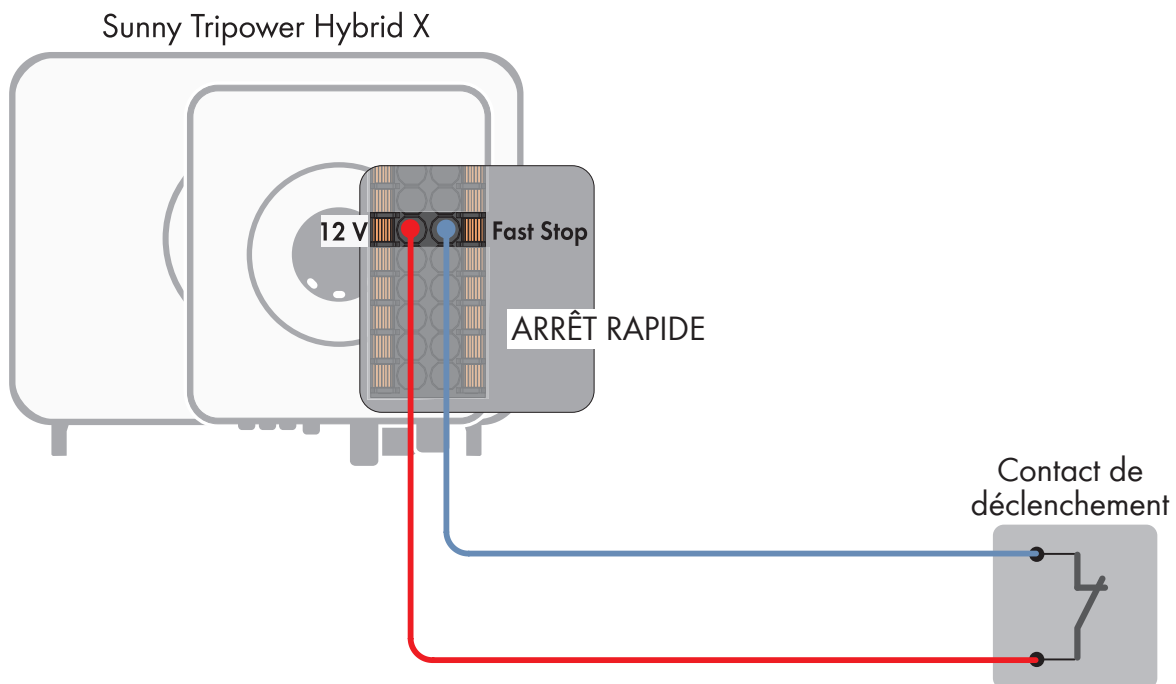
Figure 9 : Exemple de câblage pour le raccordement d'un contact de déclenchement pour l'arrêt rapide.
