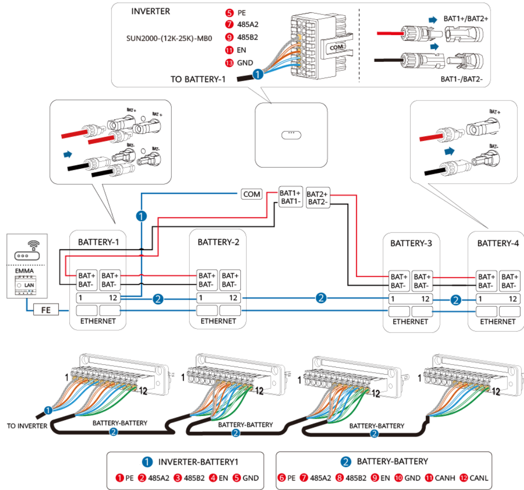
Figure 5-11 Onduleur connecté à quatre ESS
