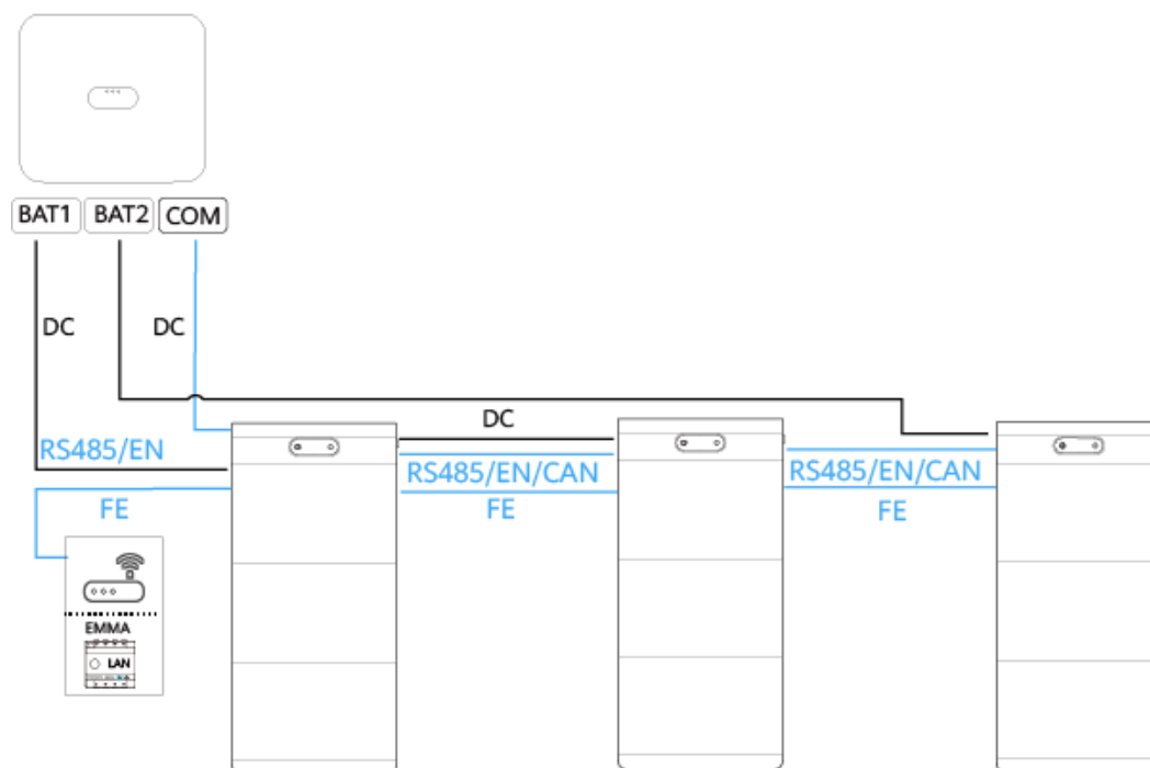
Figure 2-11 Connexion des ESS à l'onduleur (3)
