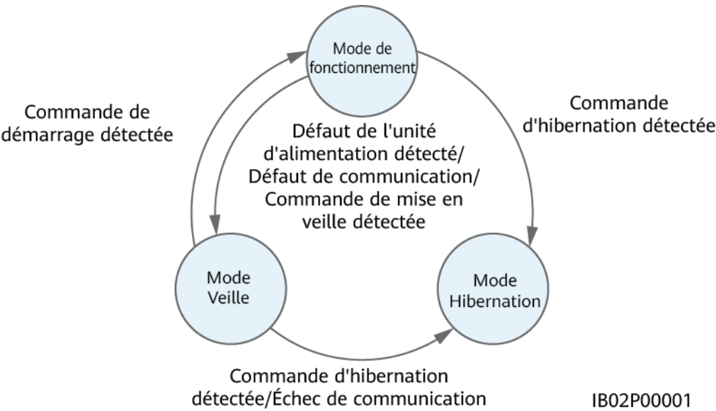
Figure 2-17 Changement de mode de fonctionnement
