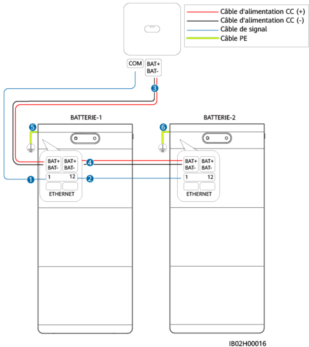
Figure 5-1 Connexion des câbles ESS
