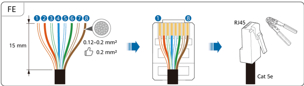
Figure 5-6 Préparation du câble réseau
