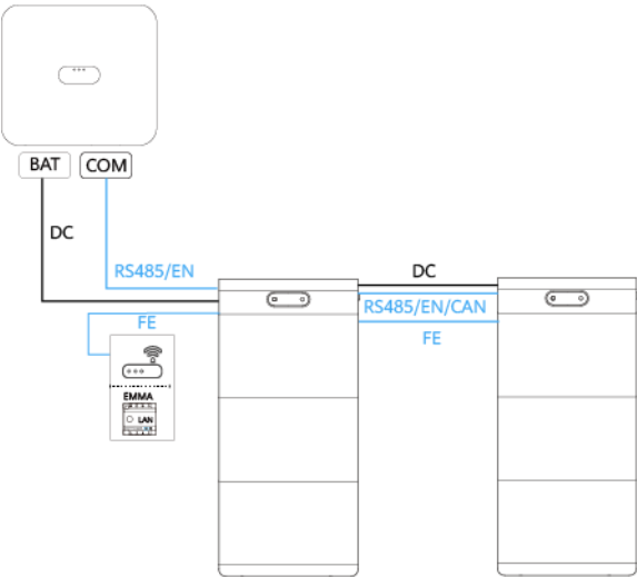
Figure 2-9 Connexion des ESS à l'onduleur (1)
