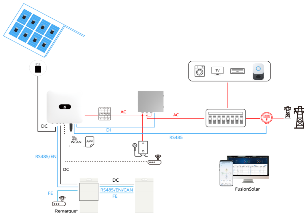
Figure 2-8 Scénario sur/hors réseau
