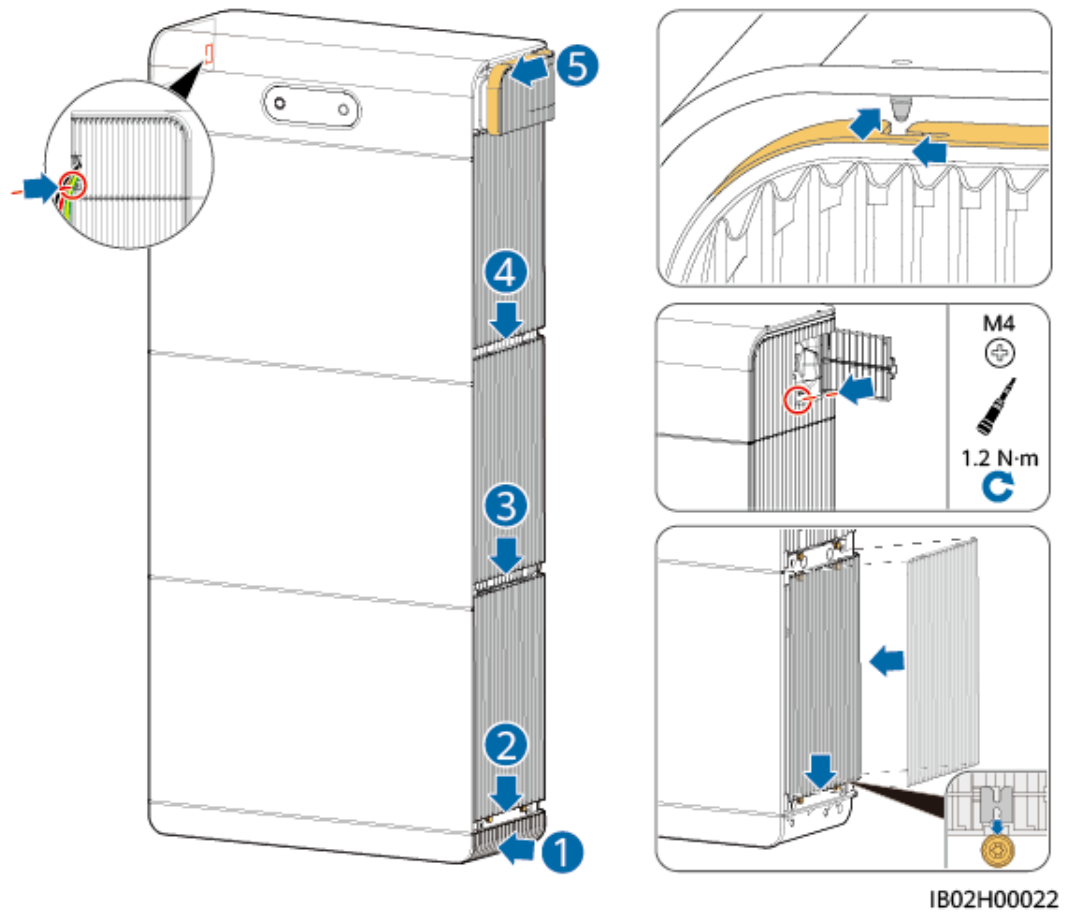
Figure 5-12 Installation des caches décoratifs
