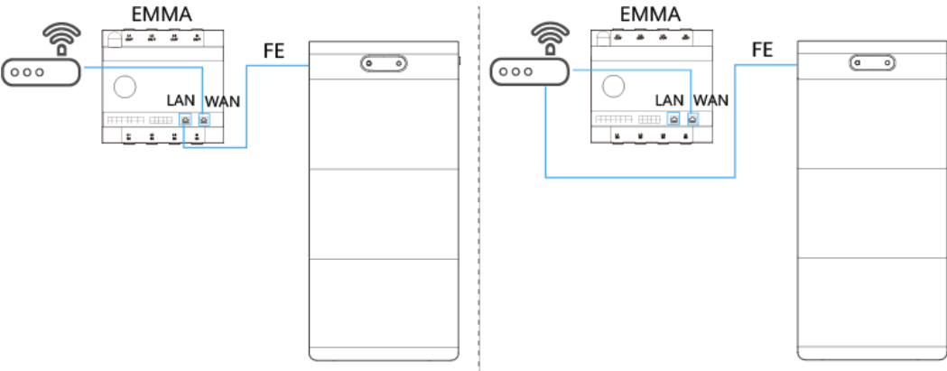
Figure 5-8 Port réseau connecté à l'EMMA ou au routeur
