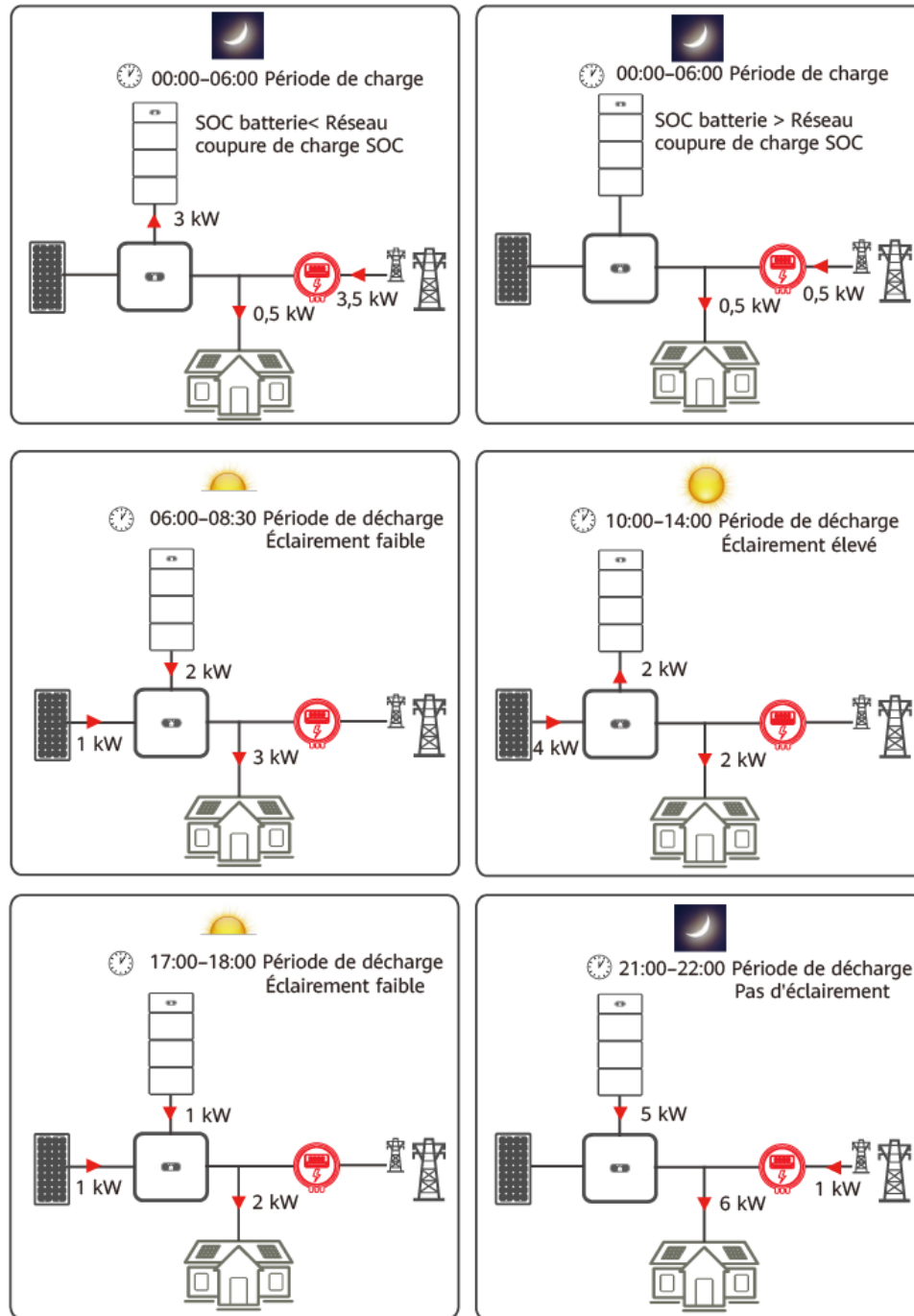
Figure 2-13 Exemple de TOU (00:00-06:00 pour la charge et 06:00-24:00 pour la décharge)
