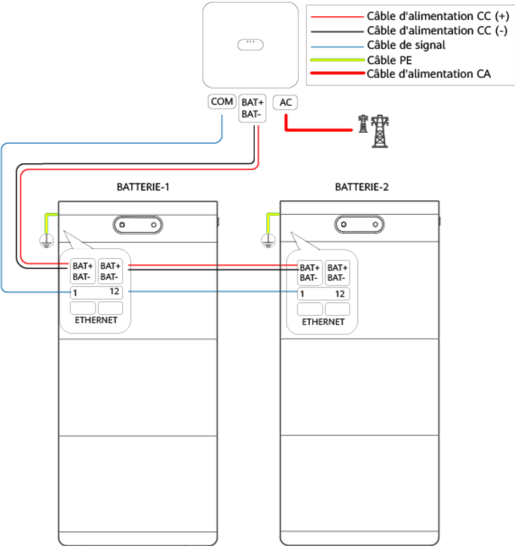
Figure 3-1 Schéma de raccordement des câbles
