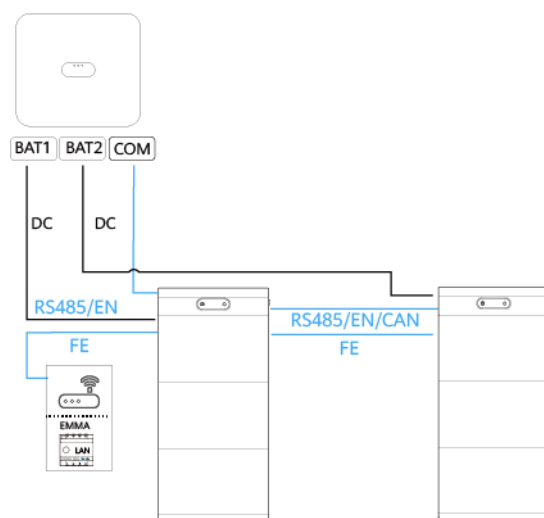
Figure 2-10 Connexion des ESS à l'onduleur (2)
