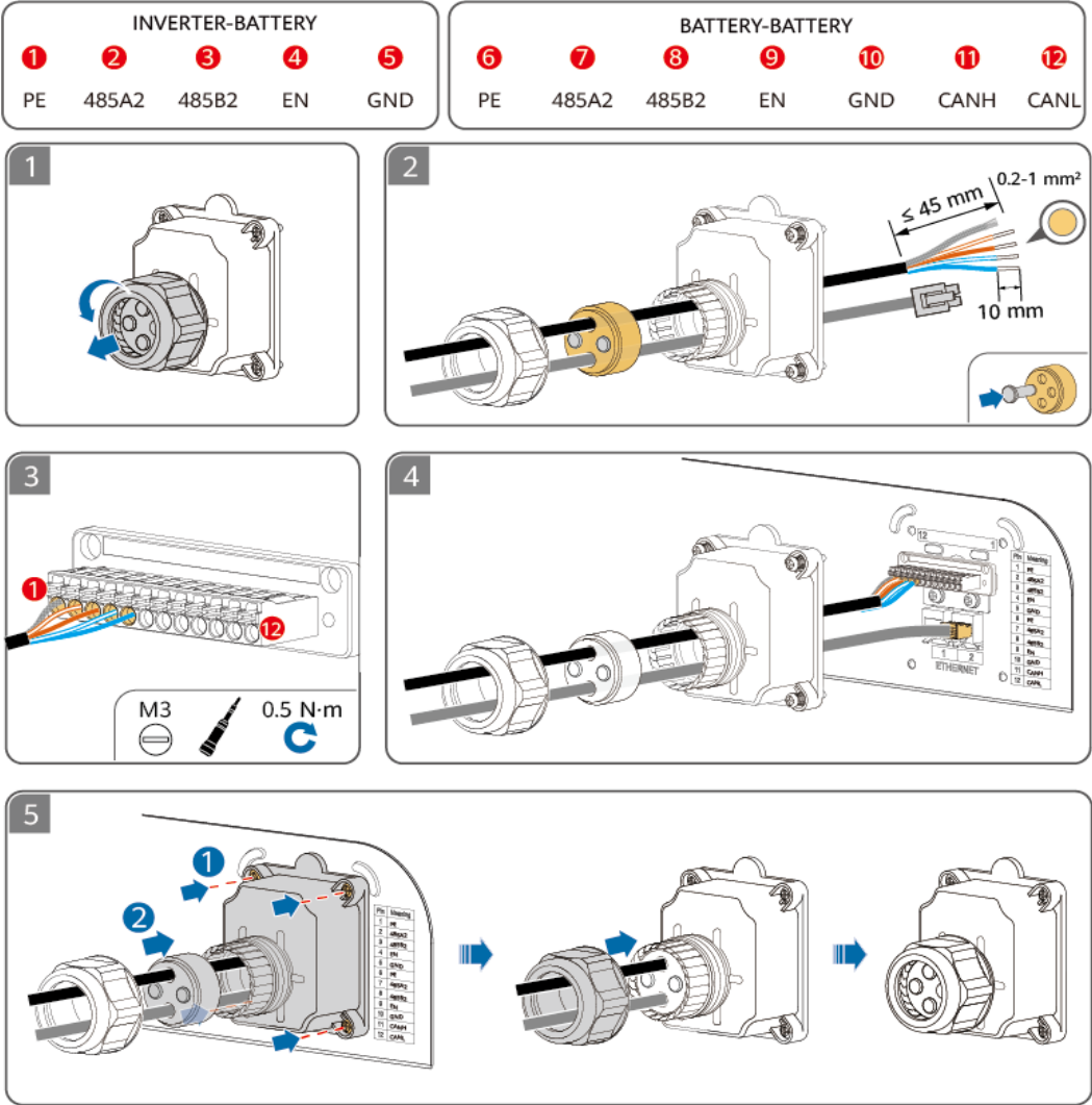
Figure 5-7 Connexions du port de signal
