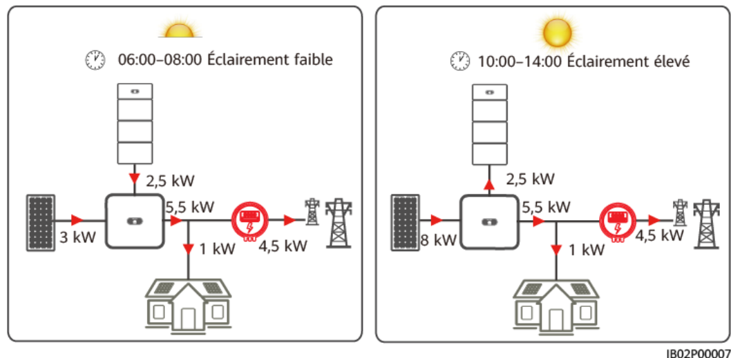
Figure 2-14 Entièrement alimenté au réseau
