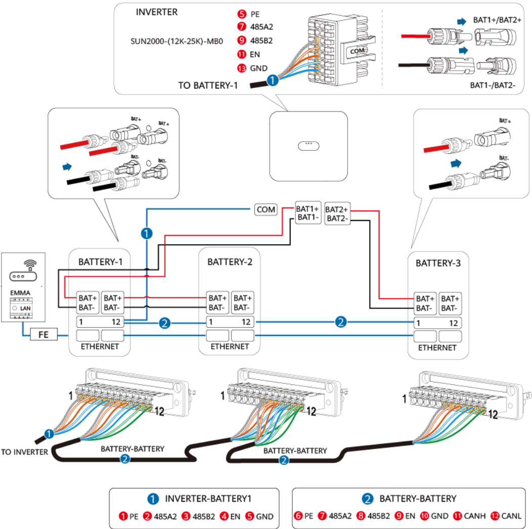
Figure 5-10 Onduleur connecté à trois ESS
