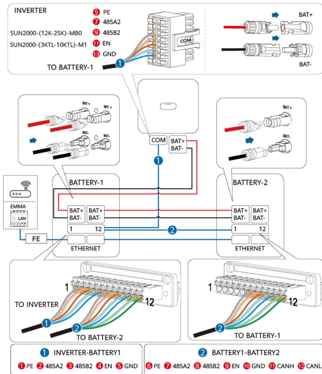
Figure 5-9 Onduleur connecté à deux ESS
