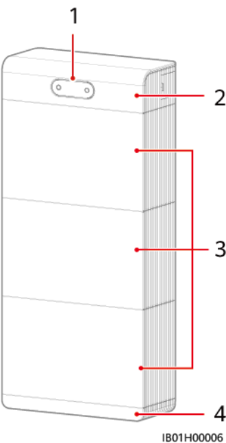
Figure 2-6 Aspect visuel de l'ESS
