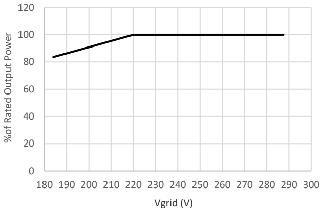
Rapport de puissance nominale par rapport à la tension du réseau
