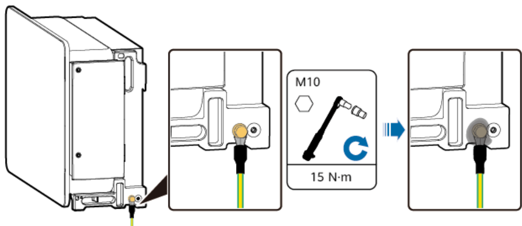
Figure 5-2 Connexion du câble PE au point PE (sur le boîtier)
