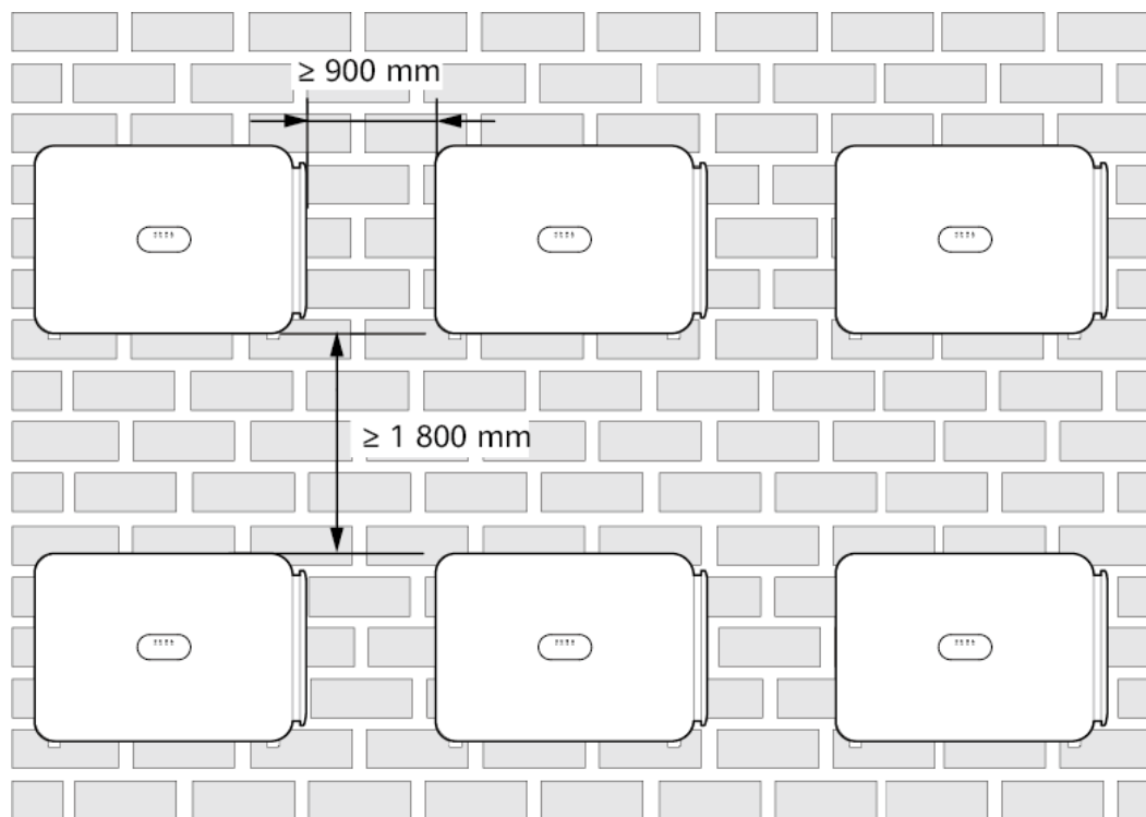
Figure 4-6 Mode d'installation empilé (non recommandé)
