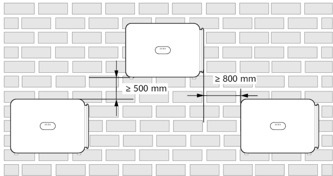
Figure 4-4 Mode d'installation en triangle (recommandé)
