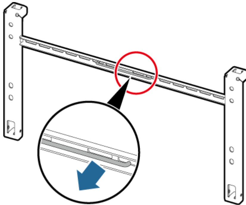
Figure 4-11 Retrait de la clé torx
