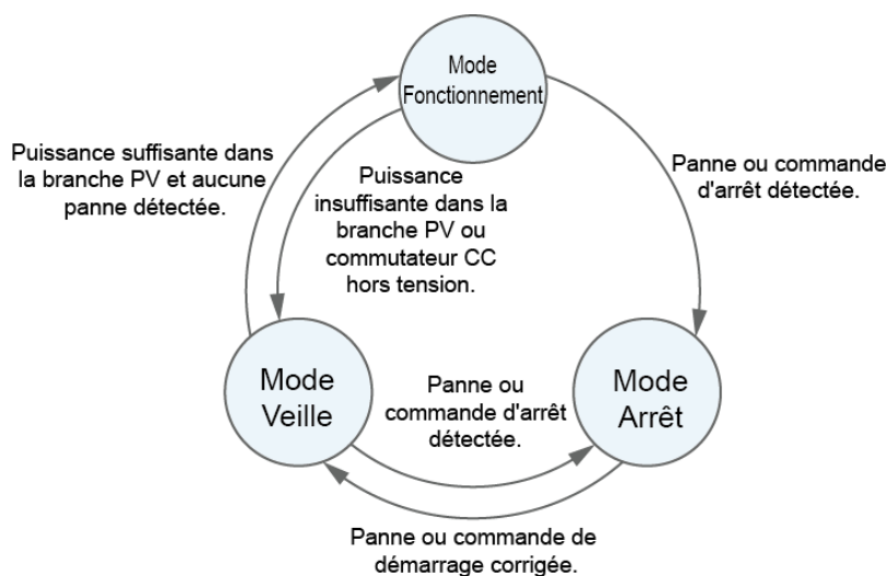
Figure 2-10 Modes de fonctionnement
