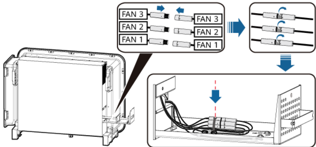
Figure 8-14 Liaison des câbles
