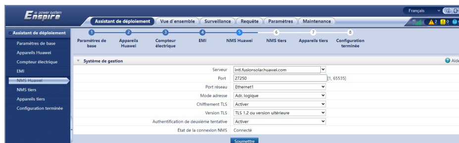
Figure 7-7 Connexion au NMS Huawei
