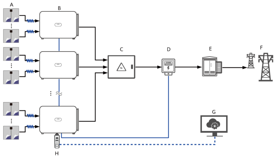
Figure 2-3 Application de mise en réseau RS485 (Dongle)
