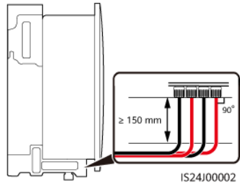
Figure 5-17 Connexion des câbles d'alimentation d'entrée CC(AVIC JONHON)
