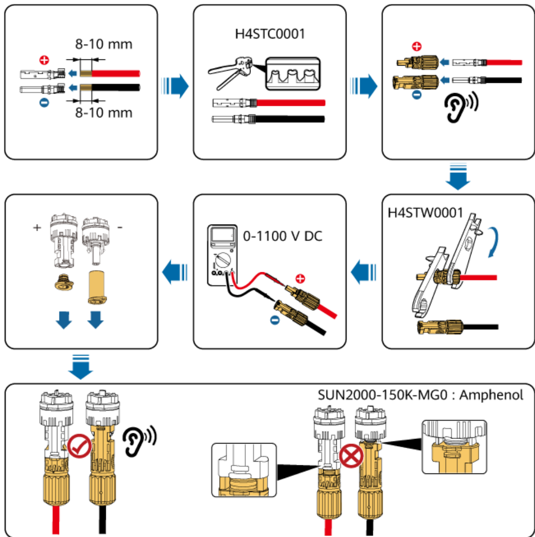
Figure 5-18 Connexion des câbles d'alimentation d'entrée CC (Amphenol)
