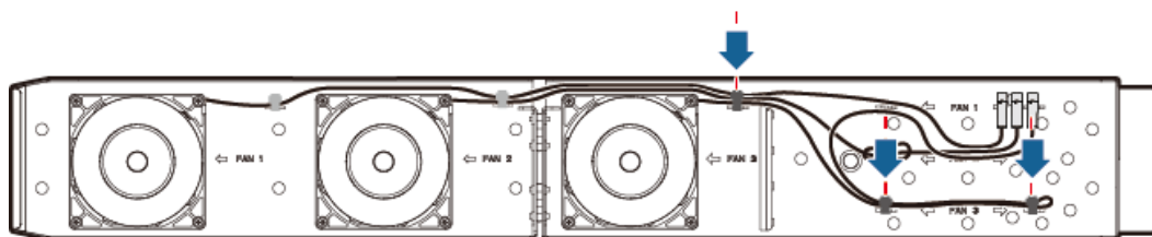
Figure 8-12 Liaison des câbles du FAN 3
