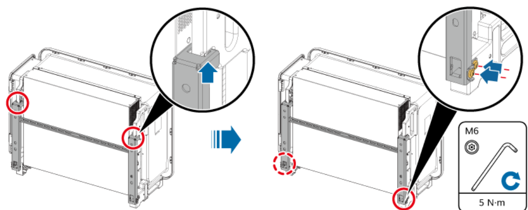
Figure 4-16 Fixation de l'onduleur
