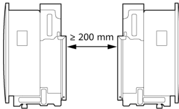
Figure 4-5 Installation dos à dos (recommandée)
