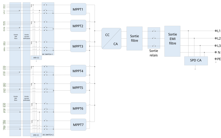
Figure 2-9 Schéma des circuits
