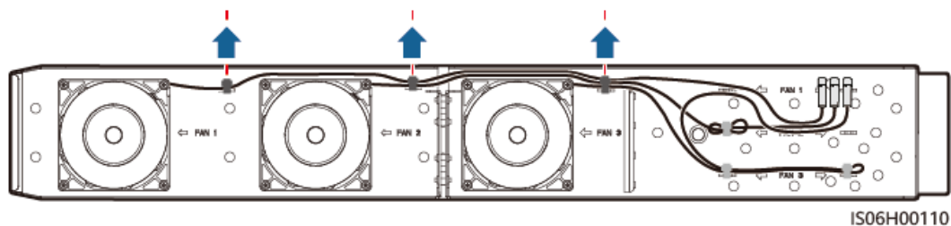
Figure 8-5 Retrait des attaches de câbles du FAN 1
