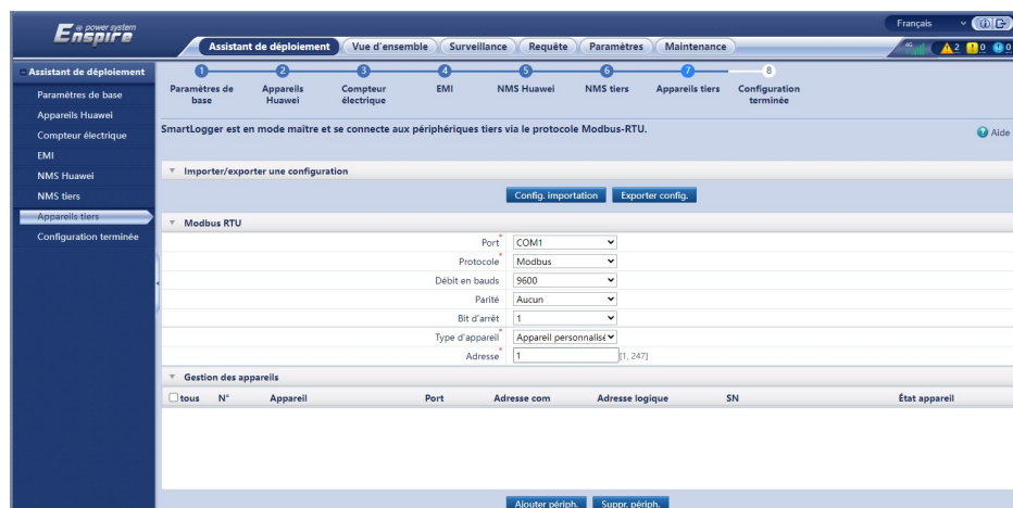
Figure 7-9 Connexion aux appareils tiers
