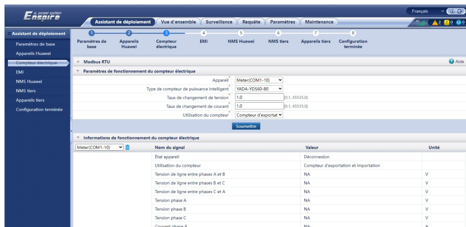
Figure 7-5 Connexion à des compteurs électriques
