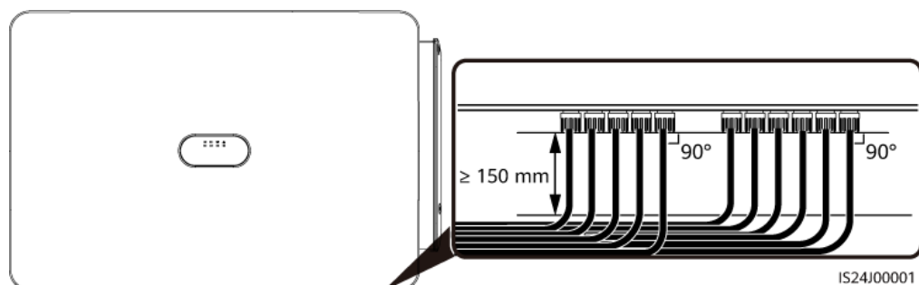
Figure 5-16 Exigences en matière de câblage d'alimentation d'entrée CC
