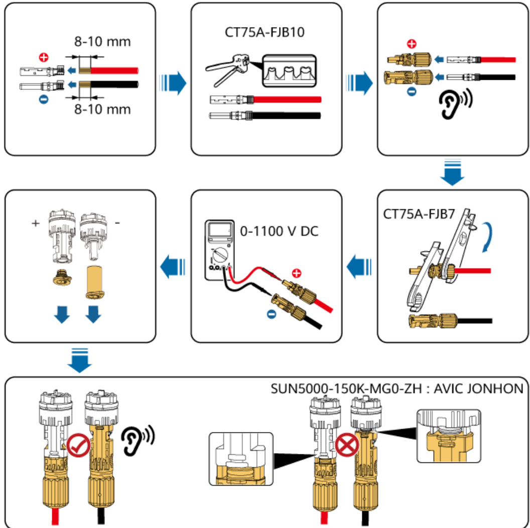
Figure 5-17 Connexion des câbles d'alimentation d'entrée CC(AVIC JONHON)
