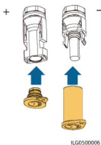
Figure 5-19 Bouchons d'étanchéité
