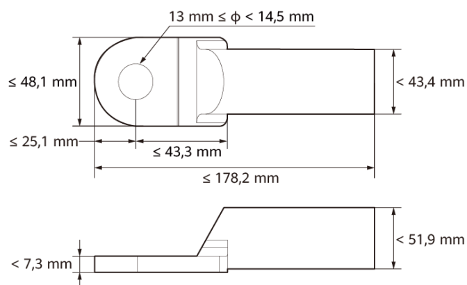
Figure 5-5 Caractéristiques de la borne OT/DT sertie
