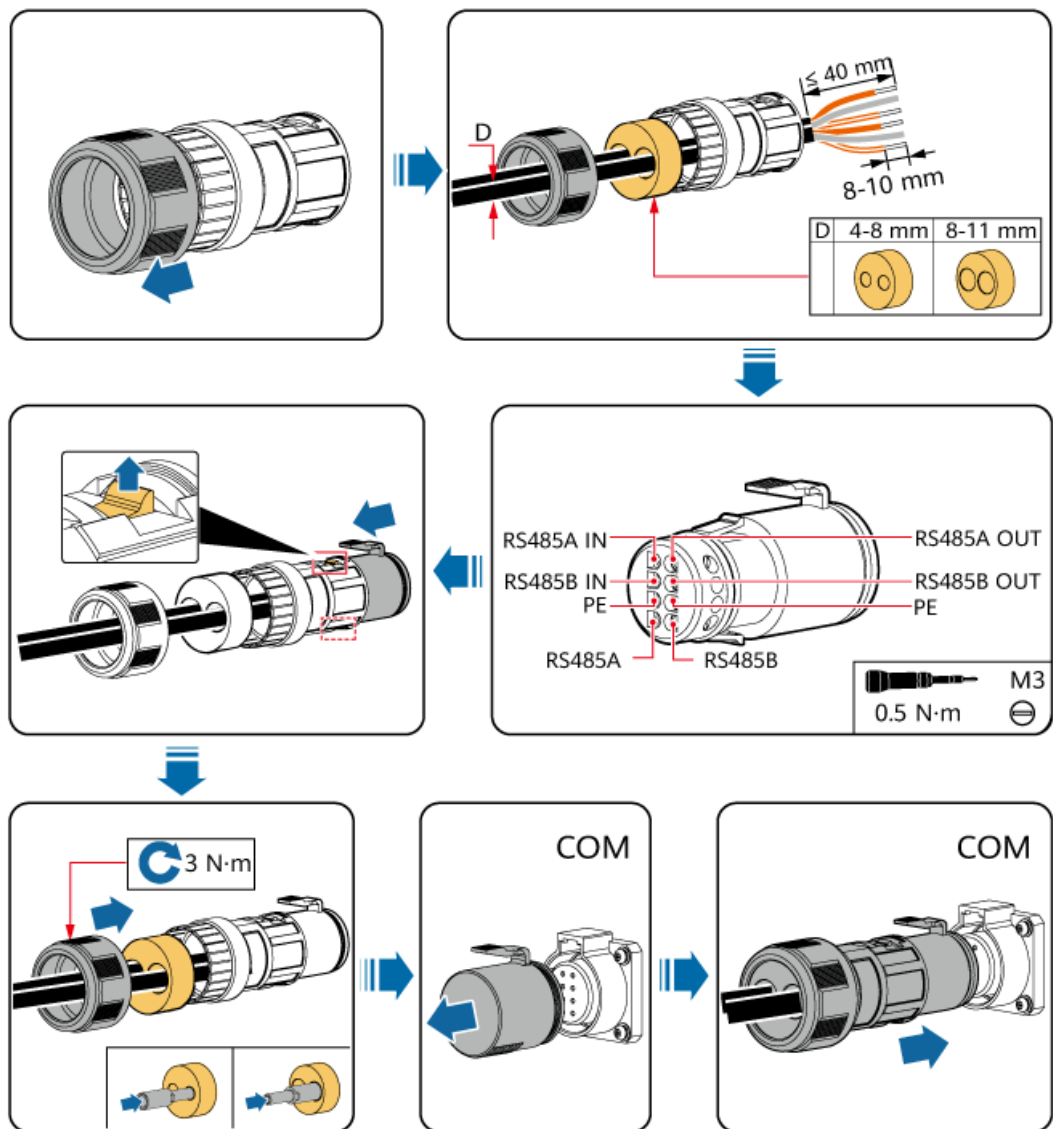
Figure 5-21 Connexion des câbles de communication
