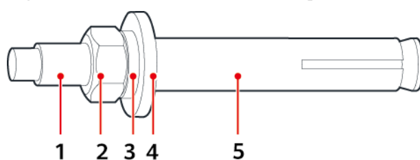
Figure 4-14 Structure d'un boulon à expansion
