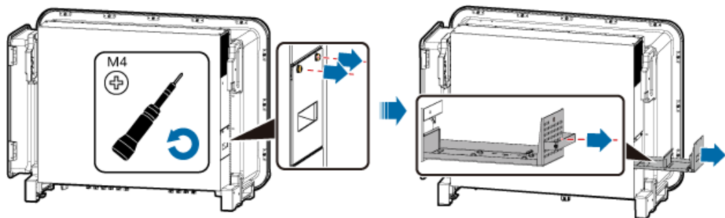
Figure 8-2 Retrait du plateau du ventilateur (1)
