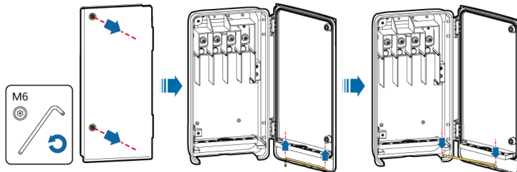
Figure 5-4 Ouverture d'une porte du compartiment de maintenance
