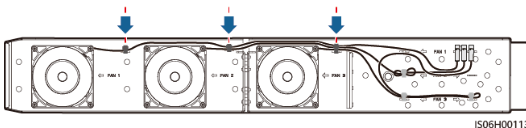
Figure 8-10 Liaison des câbles du FAN 1
