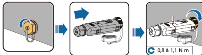
Figure 5-23 Installation du Smart Dongle WLAN-FE (SDongleA-05 pour le scénario de communication WLAN)
