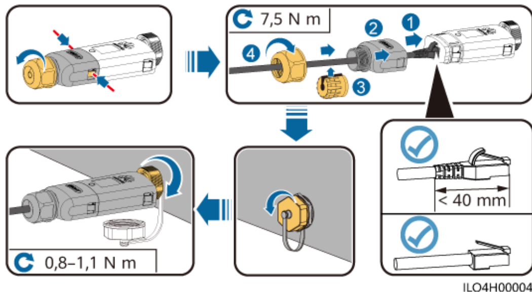
Figure 5-24 Installation du Smart Dongle WLAN-FE (SDongleA-05 pour le scénario de communication FE)
