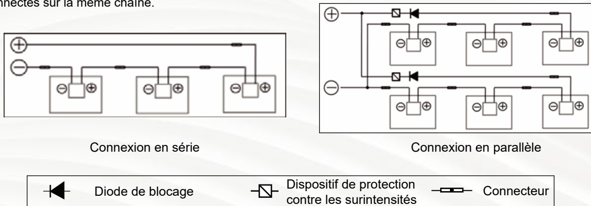
Figure 9 Schéma du circuit de connexion en série et en parallèle
