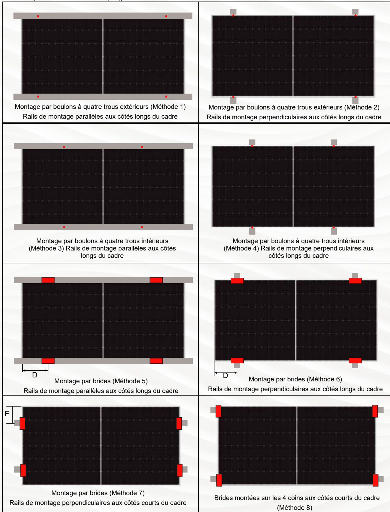
Figure 8 Position d'installation des modules bifaciaux
