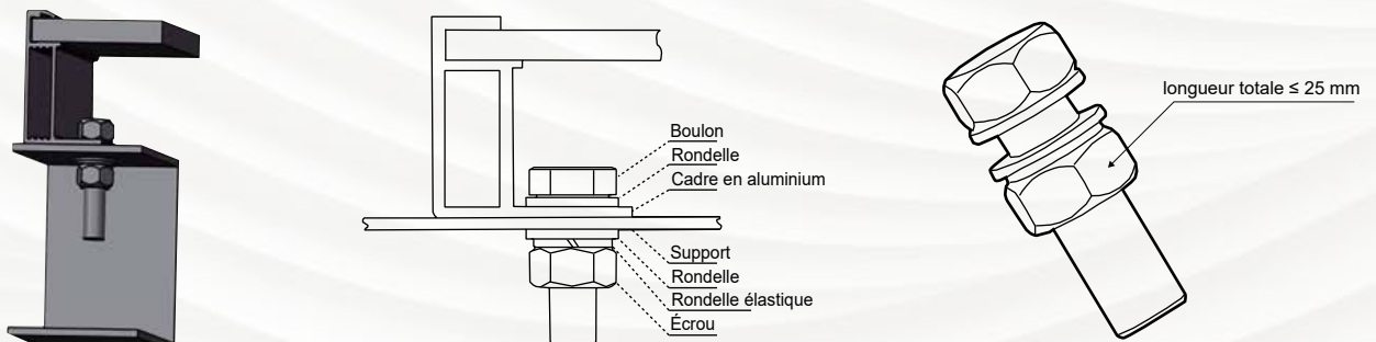
Figure 5 Installation de boulons des modules
