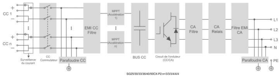
Figure 2-4 Schéma du circuit
