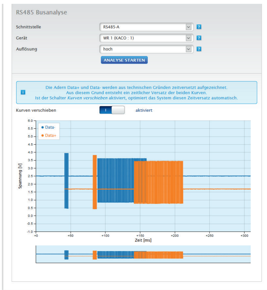
Abb.: Beispiel einer RS485-Busanalyse (bei aktiviertem Installationsmodus)
