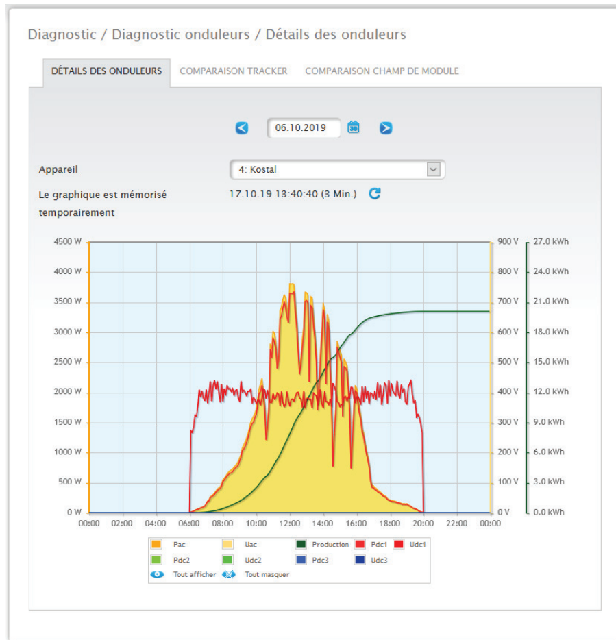
Fig. : Graphique Détails des onduleurs
