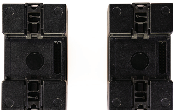
Fig. : Solar-Log™ Base et Solar-Log™ MOD 485 sans connecteur de bus.
