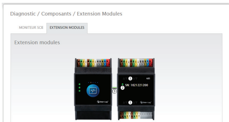
Fig. : Bus de communication/LED Solar-Log™ MOD 485 - Solar-Log™ Base
