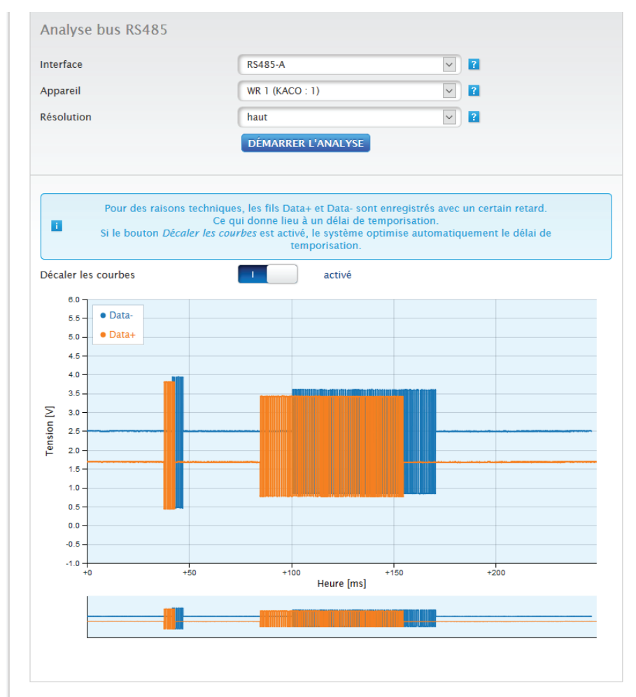
Fig. : Analyse bus RS485, exemple Janitza (mode d'installation activé)
