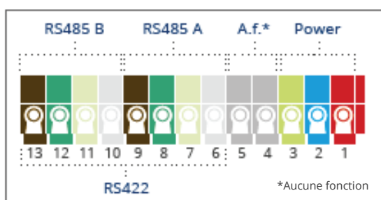
Fig. : Connexions Solar-Log™ Base - 2 x RS485 (A et B) ou 1 x RS422 - à droite, affectation des broches couleur sur l'appareil
