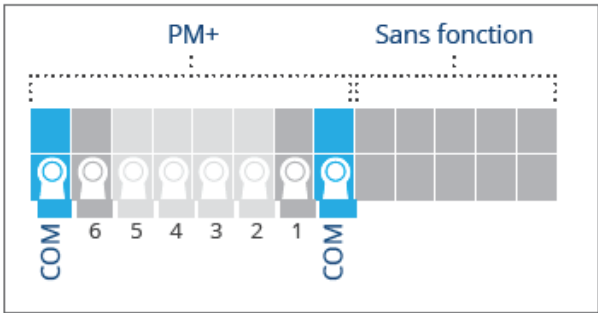
Fig. : Affectation du PIN sur la face inférieure
