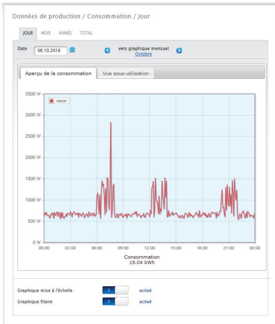
Fig. : Graphique consommation journalière avec compteurs raccordés et graphique filaire activé
