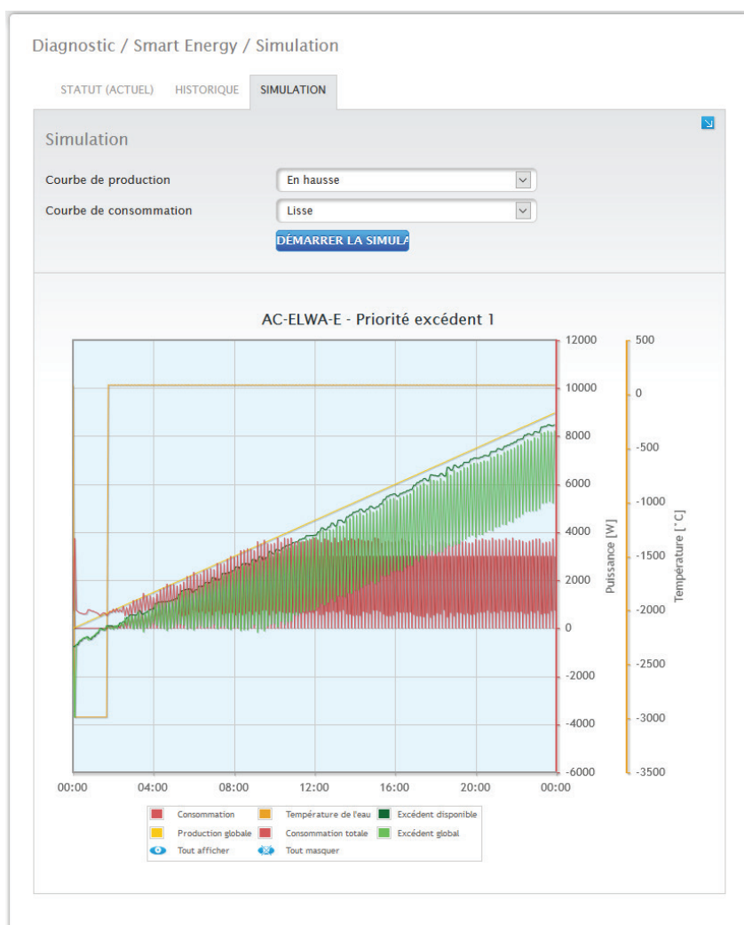
Fig. : Smart Energy – Simulation avec AC-ELWA-E – Priorité excédent 1
