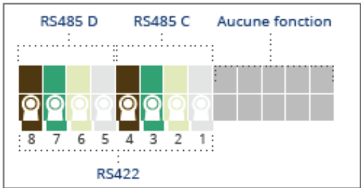
Fig. : Connexions Solar-Log™ MOD 485 – partie inférieure
