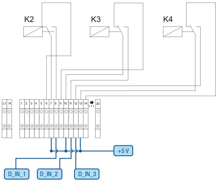
Fig. : Câblage récepteur centralisé avec 3 relais - 3ème exemple
