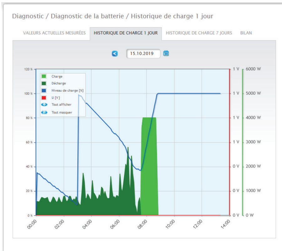
Fig. : Diagnostic de la batterie - Historique de charge 1 jour
