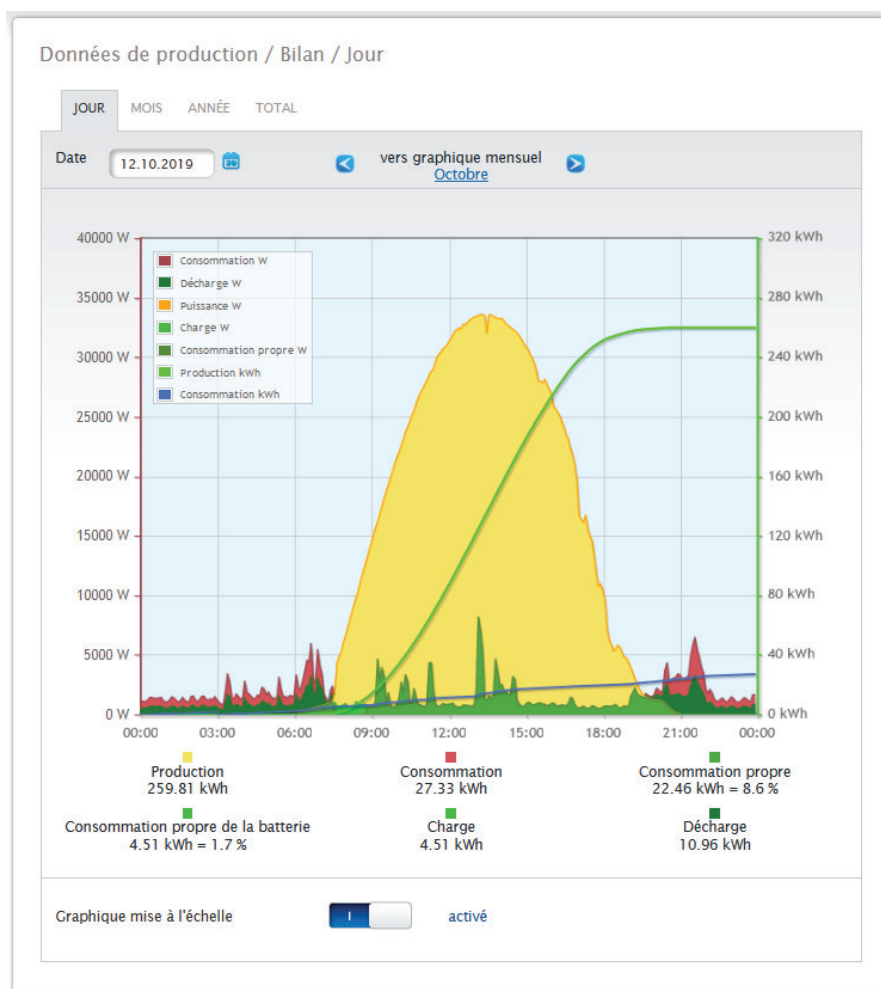
Fig. : Graphique Bilan Jour avec système batterie
