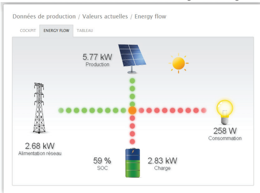
Fig. : Exemple d'installation avec le flux d'énergie
