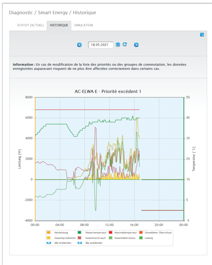
Fig. : Historique Smart Energy - Exemple Priorité 1
