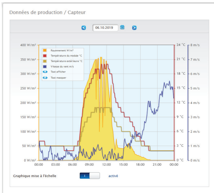
Fig. : Graphique Valeurs de la Sensorbox
