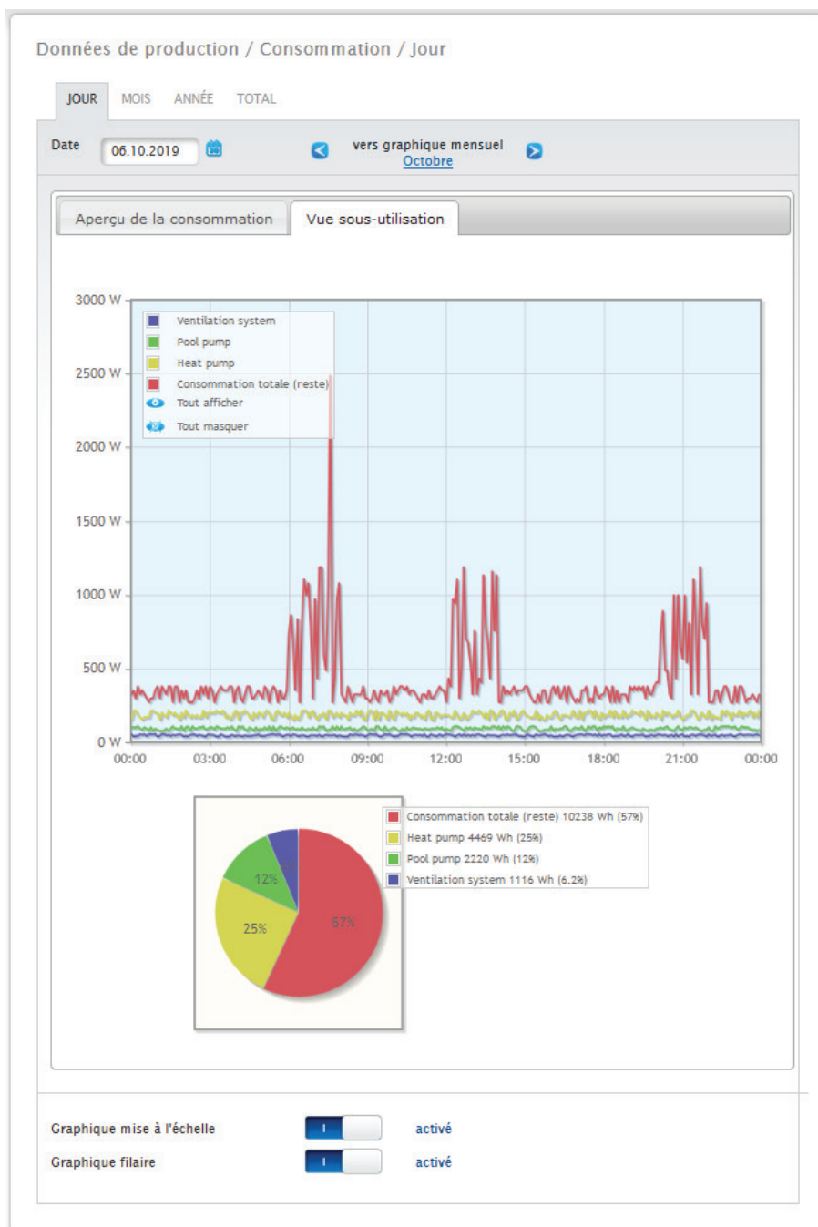
Fig. : Graphique consommation journalière avec consommateurs raccordés et graphique filaire activé dans la Vue sous-utilisation
