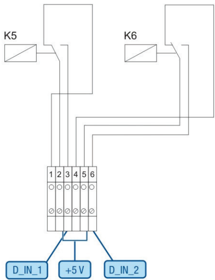
Fig. : Câblage du récepteur centralisé avec 2 relais - 2ème exemple
