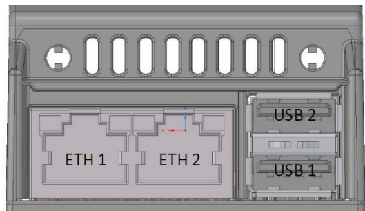
Fig. : Connexions Solar-Log™ Base – partie inférieure
