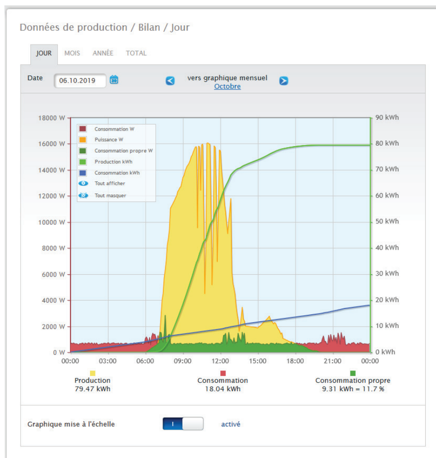
Fig. : Graphique Bilan Jour avec mise à l'échelle automatique activée
