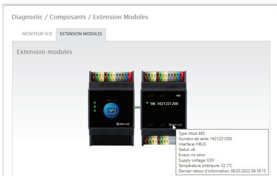
Fig. : Communication entre le Solar-Log™ MOD 485 et le Solar-Log™ Base
