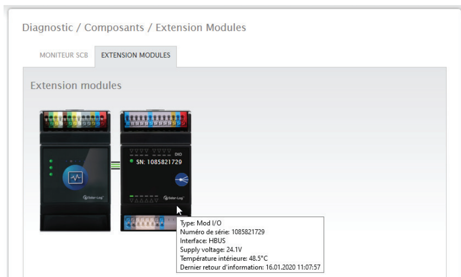
Fig. : Communication entre le Solar-Log™ MOD I/O et le Solar-Log™ Base
