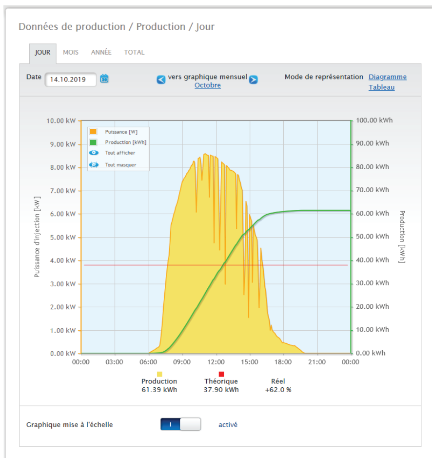
Fig. : Graphique Vue Production Jour avec mise à l'échelle automatique activée
