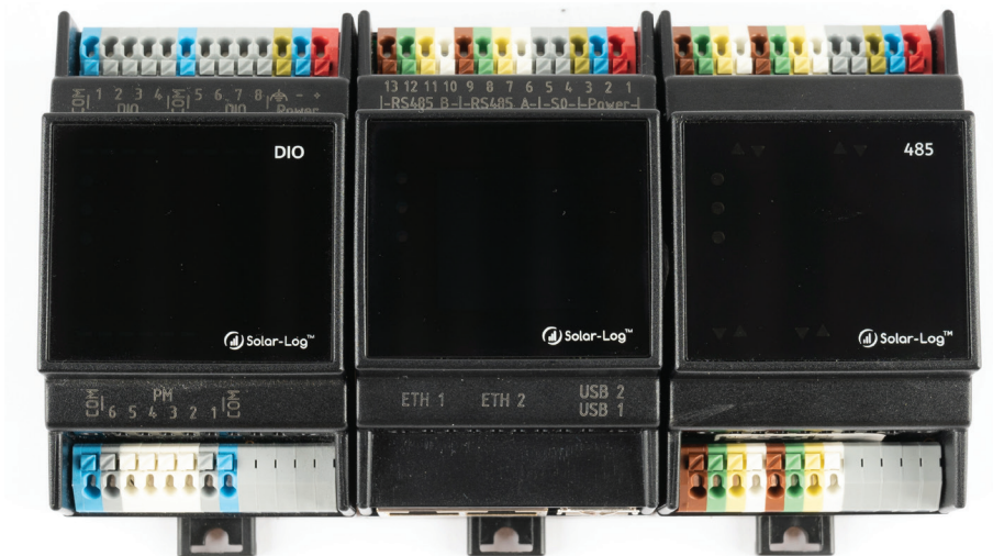
Fig. : Combinaison Solar-Log™ Base avec Solar-Log™ MOD I/O et Solar-Log™ MOD 485 (Connecté - face avant)
