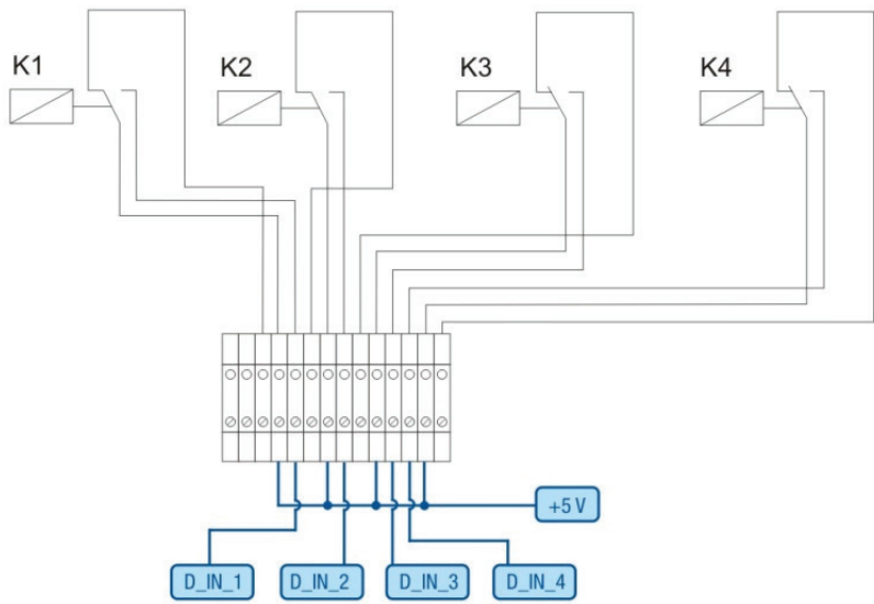
Fig. : Câblage du récepteur centralisé avec 4 relais - 1er exemple
