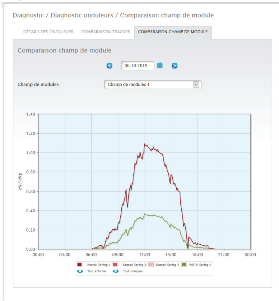
Fig. : Graphique Comparaison champ de module
