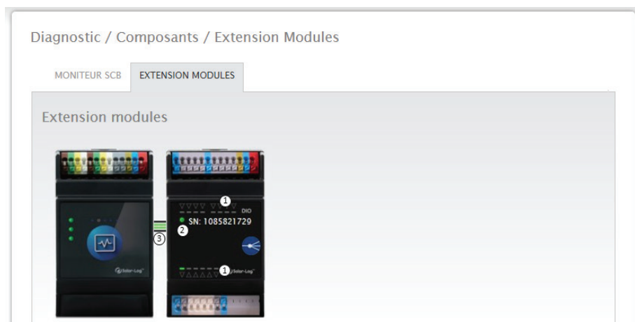
Fig. : Bus de communication/LED Solar-Log™ MOD I/O - Solar-Log™ Base
