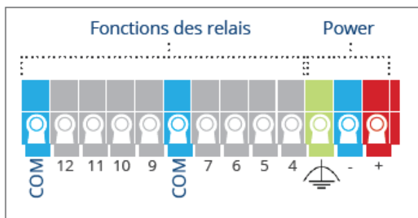
Fig. : Affectation du PIN sur la face supérieure
