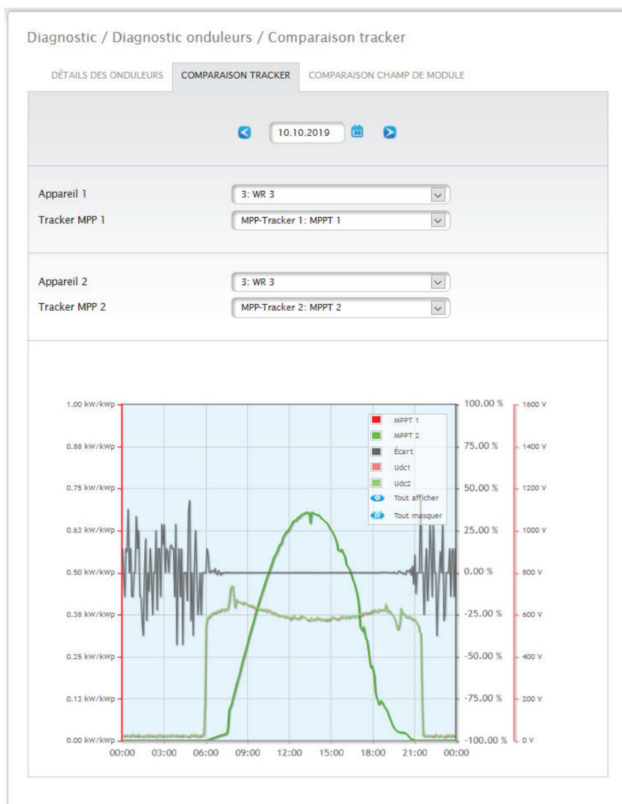
Fig. : Diagramme Comparaison tracker
