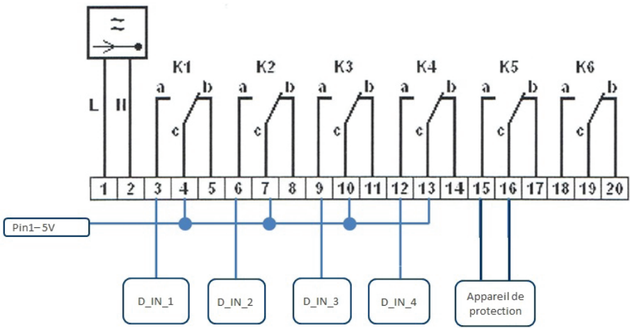
Fig. : Câblage récepteur centralisé avec 5 relais - 4ème exemple
