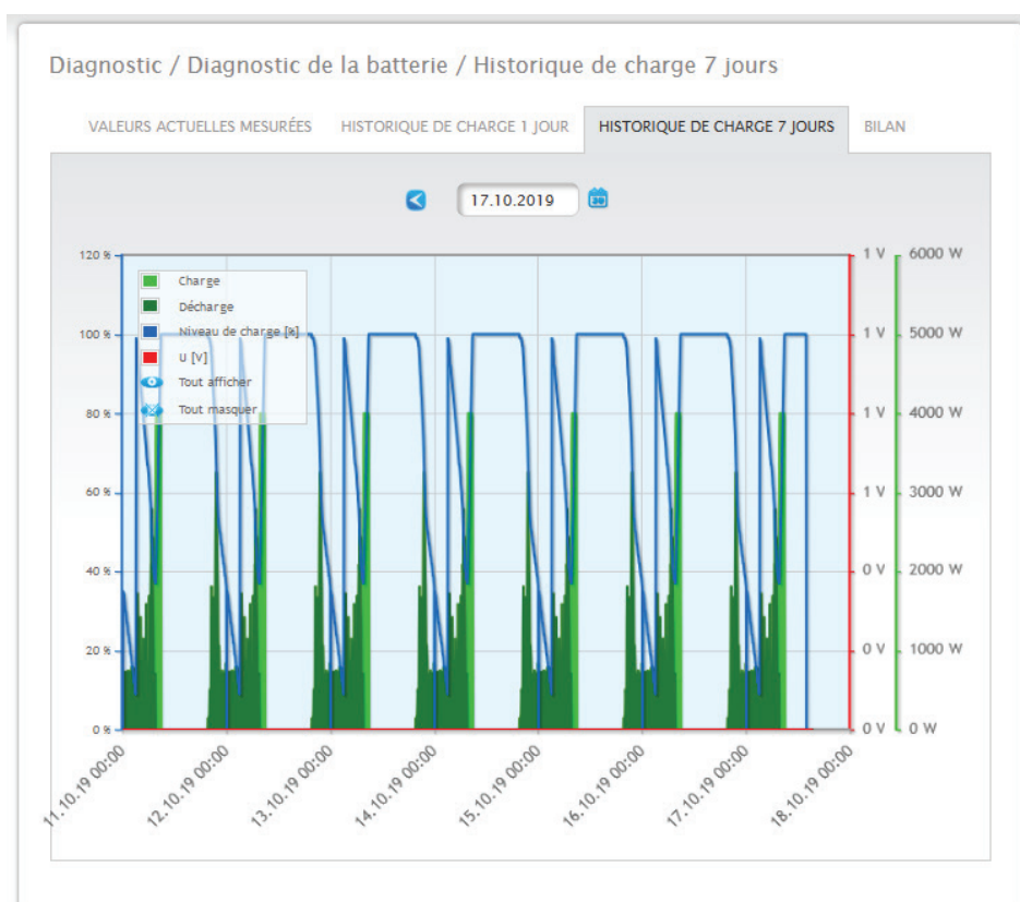
Fig. : Diagnostic de la batterie - Historique de charge 7 jours
