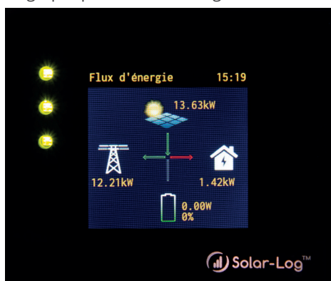
Fig. : Exemple d'installation avec le flux d'énergie
