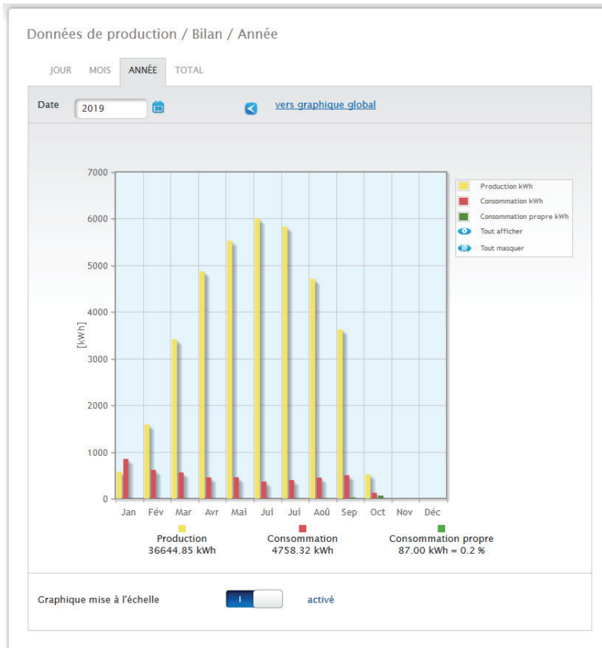
Fig. : Graphique Bilan Année
