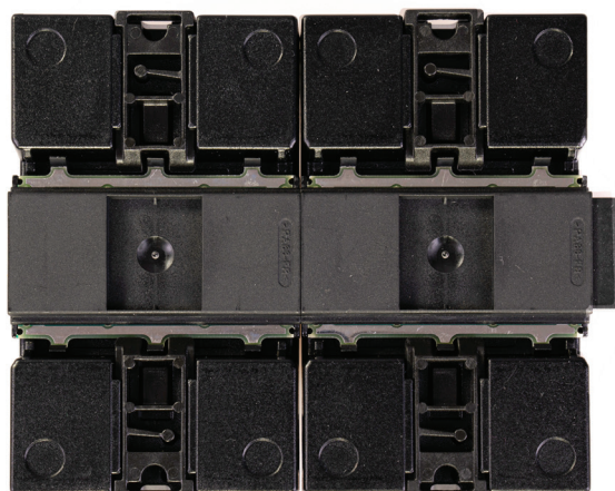
Fig. : Solar-Log™ Base et Solar-Log™ MOD I/O assemblés avec connecteur de bus
