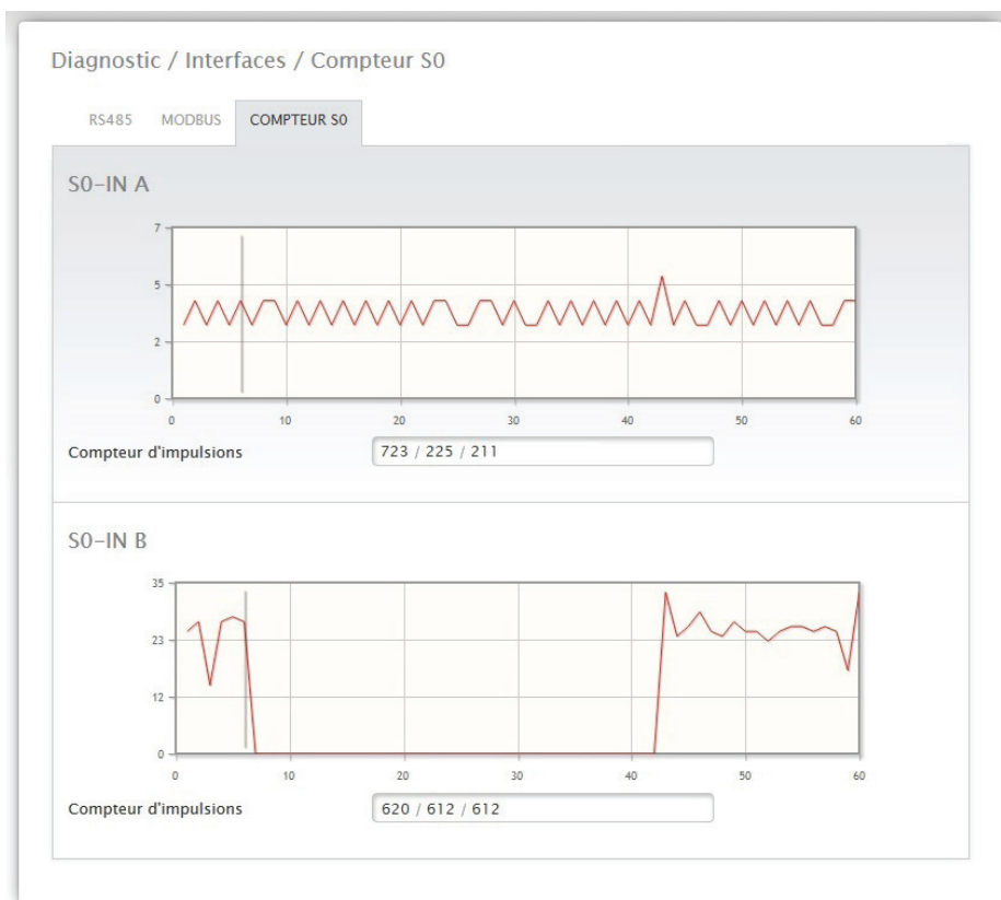
Fig. : Composants - compteur S0 sur interface A et B
