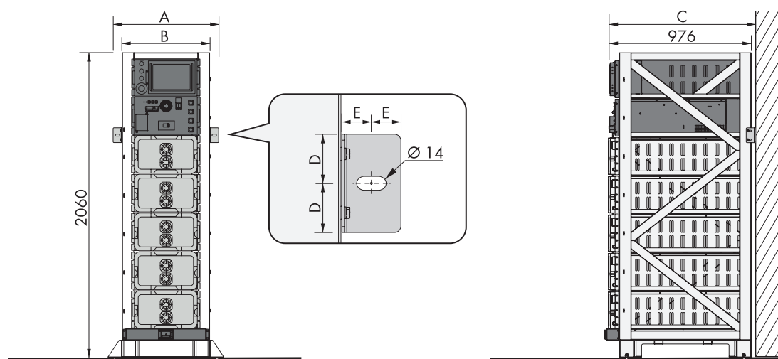
Figure 23 : Cotes de montage de la variante intérieure de l'armoire de batteries (dimensions en mm)
