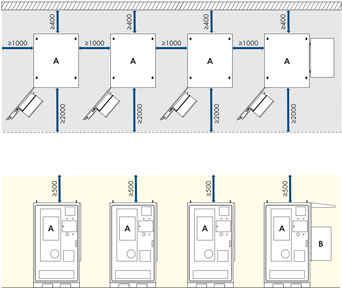
Figure 19 : Exemple d'implantation d'un système avec 4 armoires de batteries (dimensions en mm)
