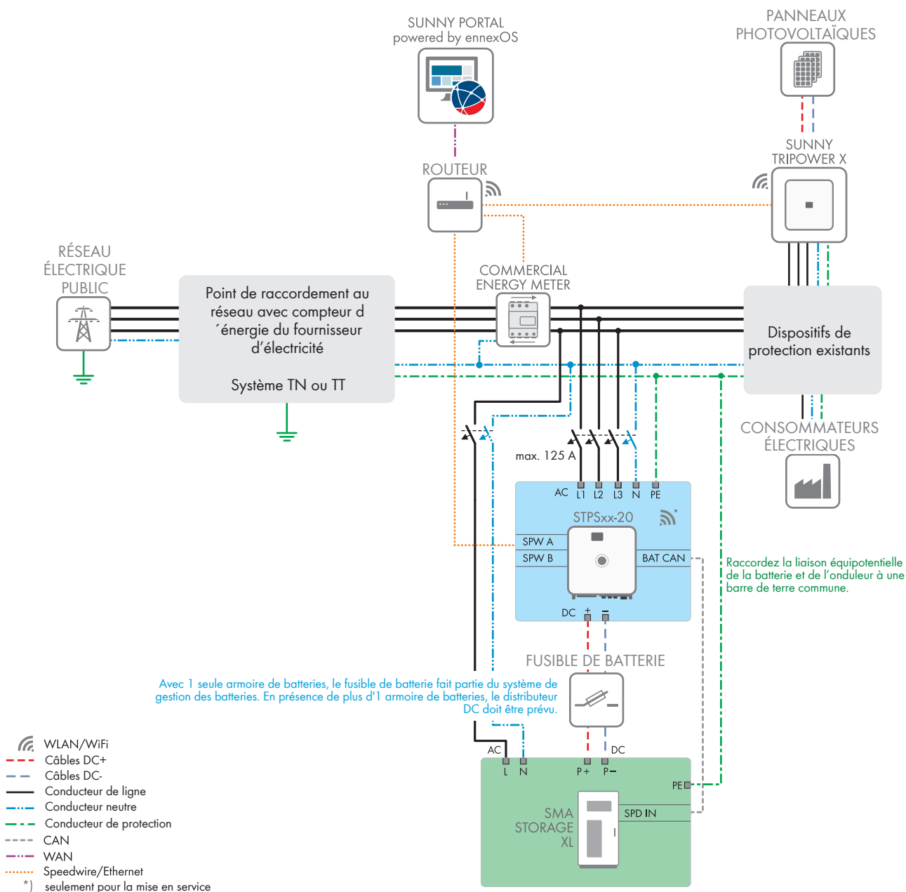
Figure 28 : SMA Storage XL Package avec 1 onduleur-chargeur et 1 armoire de batteries de la variante extérieure (exemple)
