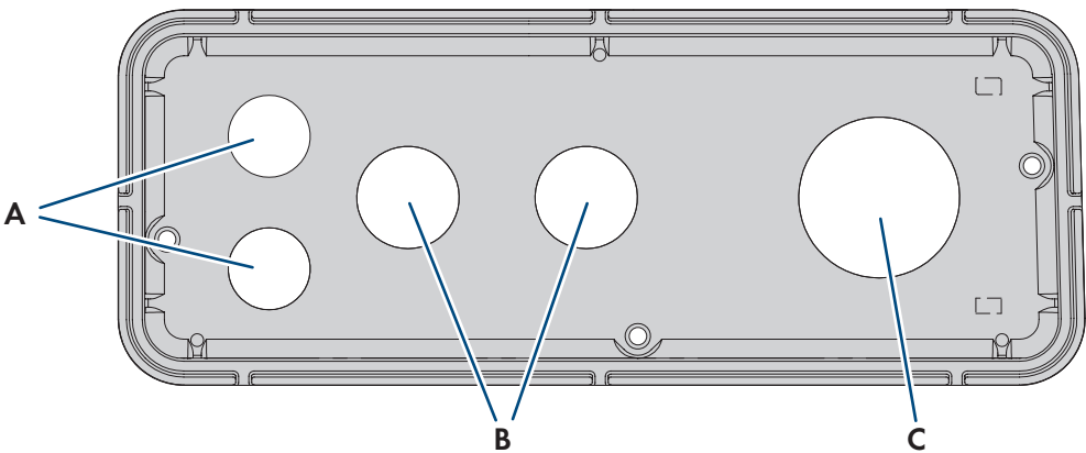
Figure 26 : Position des ouvertures de boîtier
