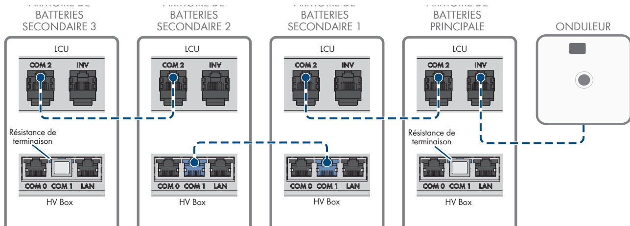
Figure 38 : Structure de la communication CAN de la variante intérieure à l'exemple d'un système avec 1 armoire de batteries primaire et 3 armoires de batteries secondaires
