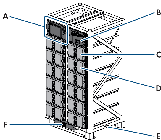
Figure 12 : Structure de l'armoire de batteries de la variante intérieure
