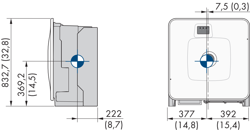
Figure 27 : Dimension du centre de gravité du produit (mesures en mm (in))
