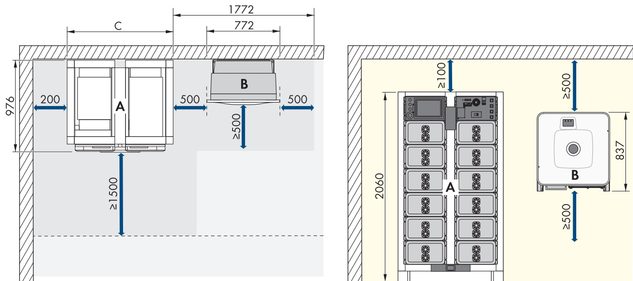
Figure 16 : Exemple d'implantation d'un système avec 1 armoire de batteries (dimensions en mm)
