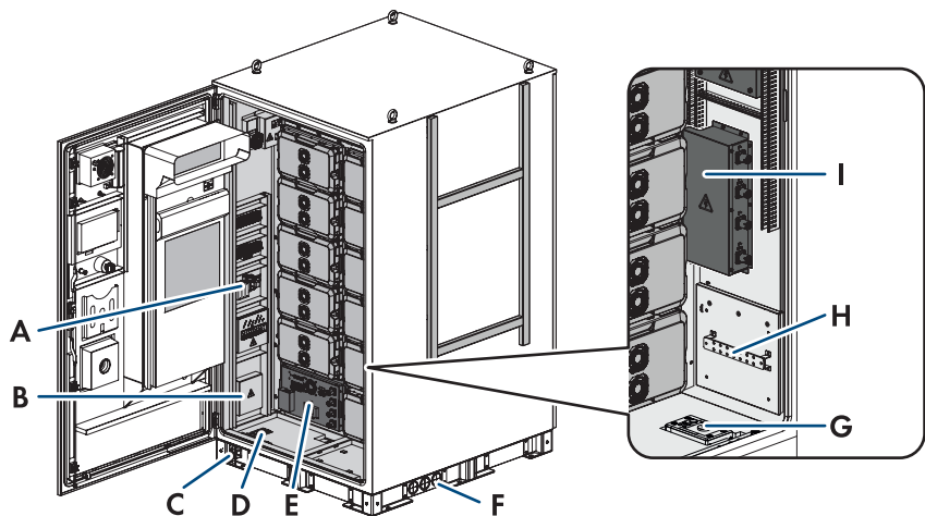
Figure 35 : Zone de raccordement de l'armoire de batteries
