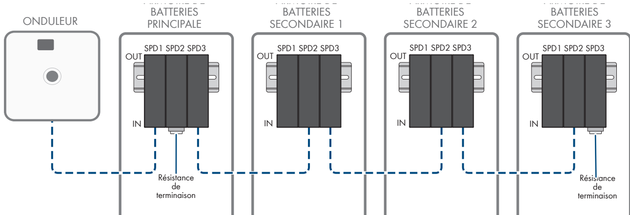
Figure 37 : Structure de la communication CAN de la variante extérieure à l'exemple d'un système avec 1 armoire de batteries primaire et 3 armoires de batteries secondaires
