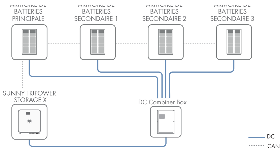
Figure 14 : Structure modulaire de la batterie pour la variante intérieure
