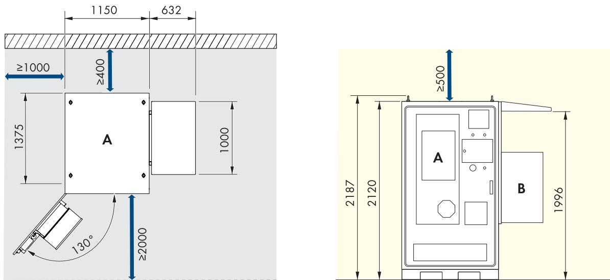
Figure 18 : Exemple d'implantation d'un système avec 1 armoire de batteries (dimensions en mm)
