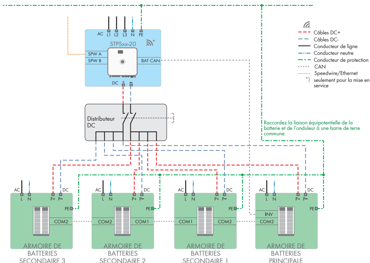
Figure 29 : Raccordement de la batterie à l'onduleur-chargeur via un distributeur DC avec 4 armoires de batteries de la variante intérieure (exemple)
