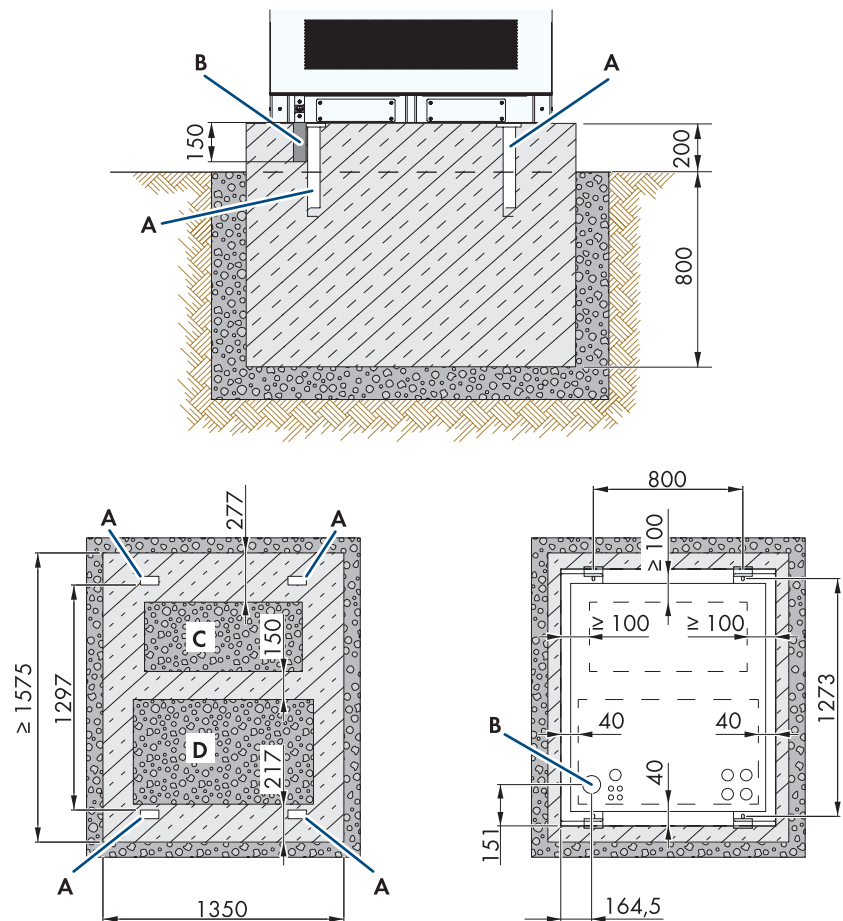
Figure 25 : Structure de la sous-fondation pour la version extérieure ; en haut, une coupe transversale vue de face ; en bas, une vue de dessus de la sous-fondation sans et avec armoire de batteries (dimensions en mm)
