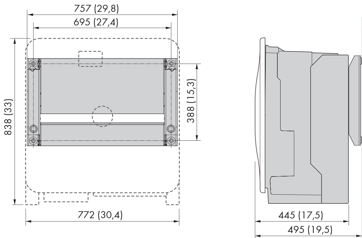
Figure 21 : Position des points de fixation (dimensions en mm (in))
