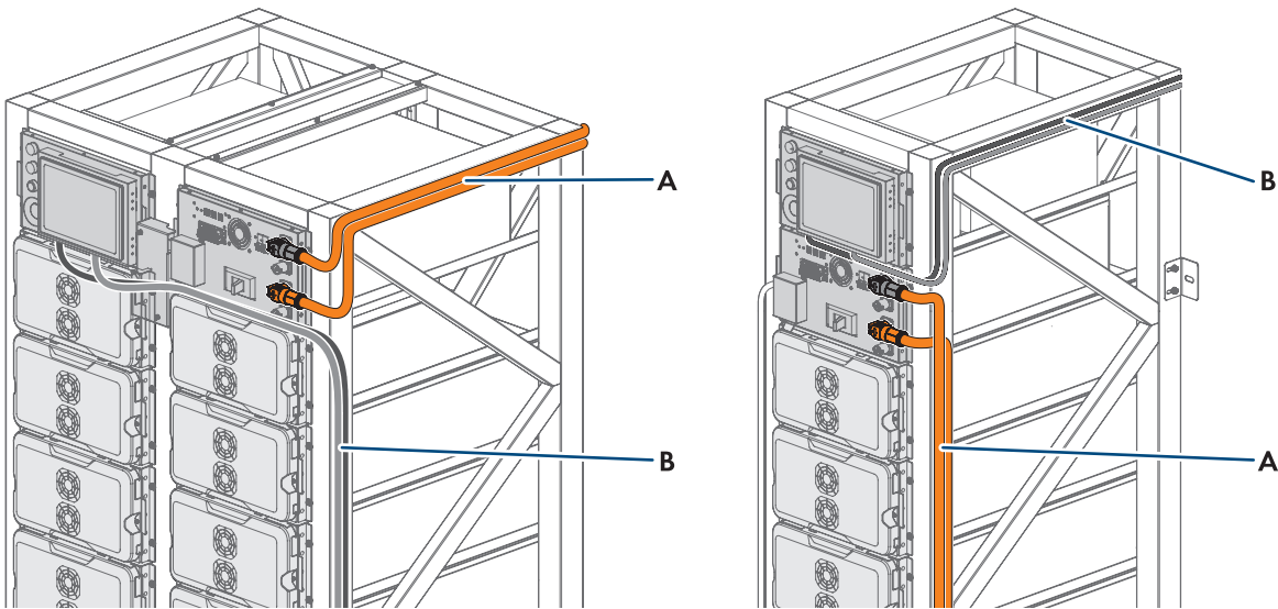
Figure 33 : Exemple de pose séparée des câbles avec la variante intérieure de l'armoire de batteries
