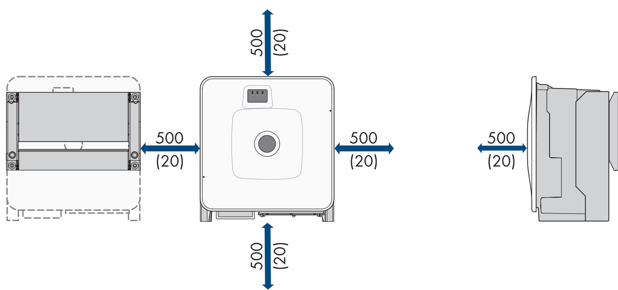
Figure 22 : Distances recommandées (dimensions en mm (in))
