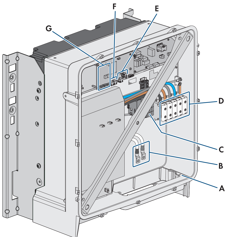
Figure 31 : Zones de raccordement situées à l'intérieur du produit
