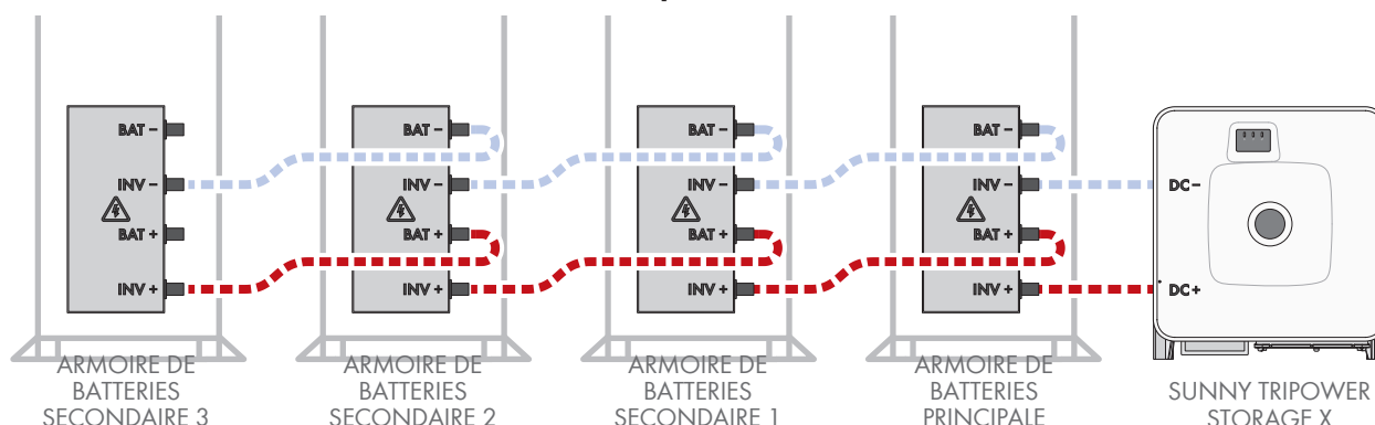
Figure 36 : Raccordement des câbles DC à l'exemple d'un système avec 1 armoire de batteries principale et 3 armoires de batteries secondaires
