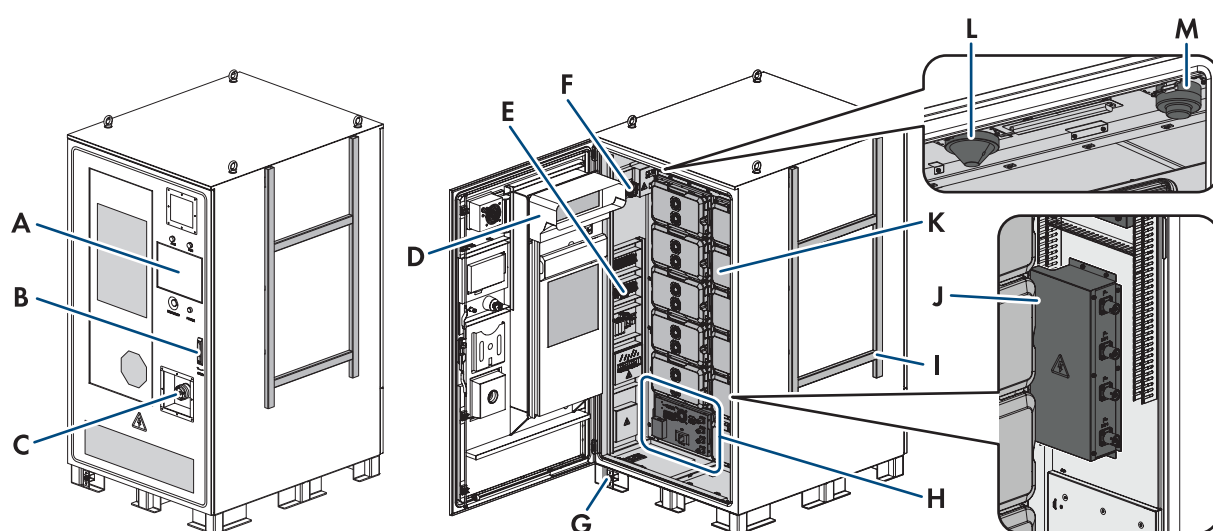
Figure 13 : Structure de l'armoire de batteries de la variante extérieure
