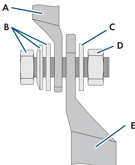
Figure 32 : Aperçu du raccordement DC
