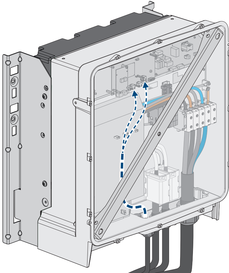
Figure 30 : Vue intérieure de l'onduleur avec plan de pose pour le câble réseau/câble de communication avec la batterie
