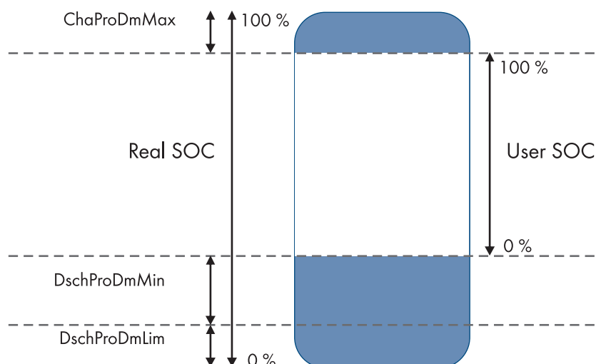
Figure 11 : Zones de l'état de charge de la batterie
