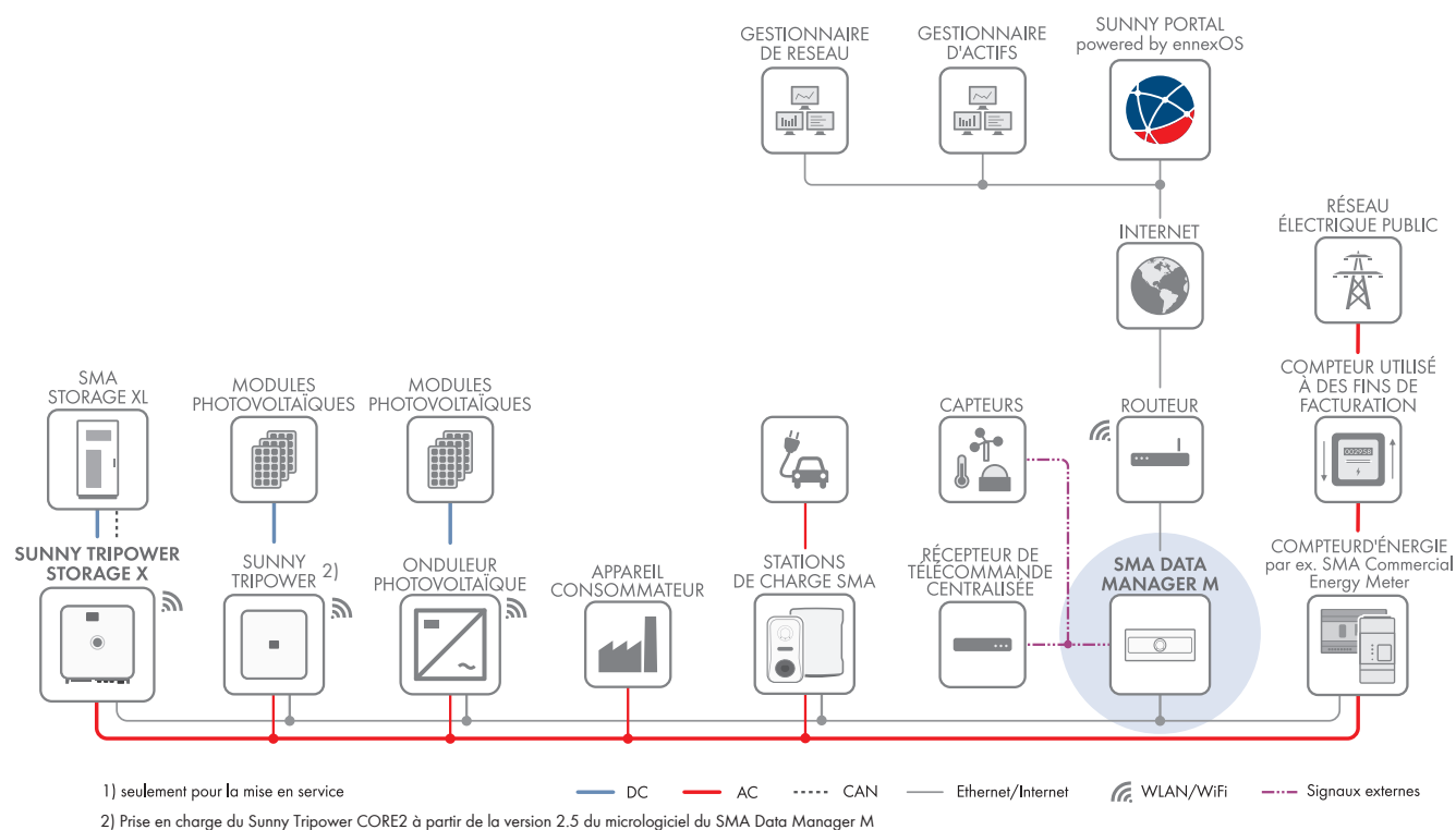
Figure 9 : Sunny Tripower Storage X avec SMA Data Manager M en tant que System Manager (exemple)
