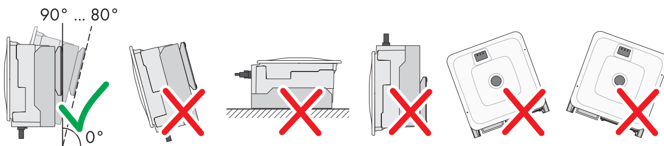
Figure 20 : Positions de montage autorisées et non autorisées
