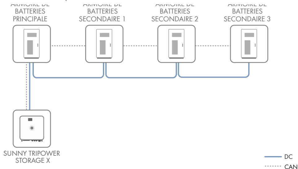
Figure 15 : Structure modulaire de la batterie pour la variante extérieure
