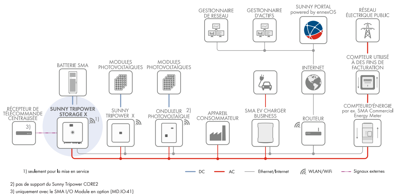
Figure 8 : Sunny Tripower Storage X en tant que System Manager (exemple avec raccordement du récepteur de télécommande centralisée à l'onduleur)
