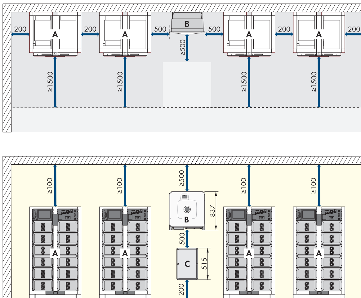
Figure 17 : Exemple d'implantation d'un système avec 4 armoires de batteries (dimensions en mm)
