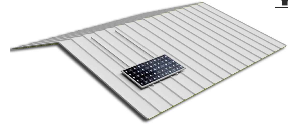
Perfiles perpendiculares a la cumbre
