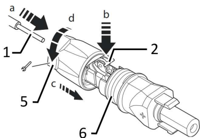
Abb. 18: Adern einfügen
