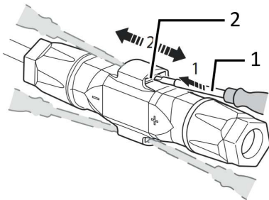
Abb. 35: Steckverbinder abstecken
