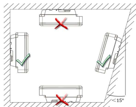
Abb. 4: Erlaubte Aufstelllage
