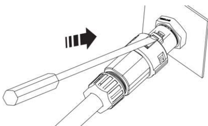
Abb. 32: AC-Anschlussstecker lösen
