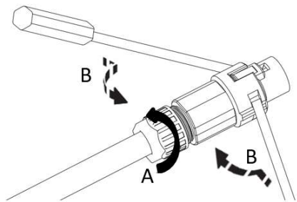
Abb. 34: Leitung lösen
