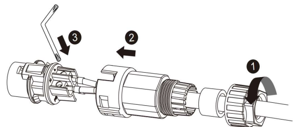
Abb. 16: Kabelverschraubung anziehen
