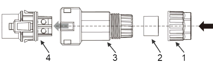
Abb. 13: AC-Anschlussstecker
