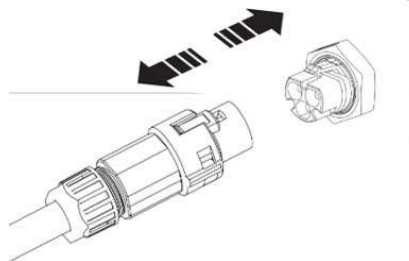
Abb. 33: AC-Anschlussstecker trennen
