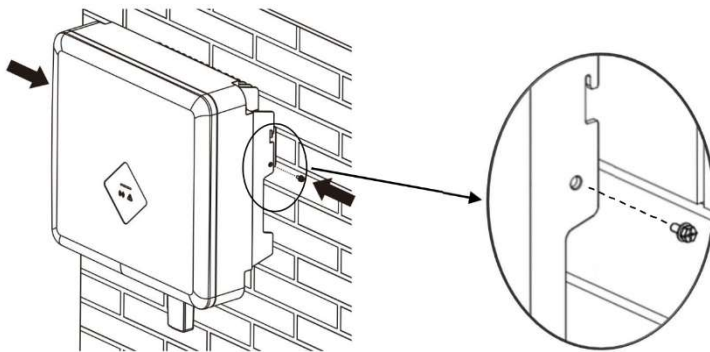
Abb. 11: Wechselrichter befestigen
