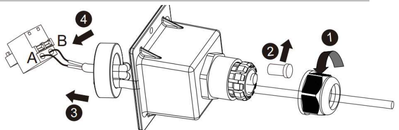
Abb. 27. Leitung durch Terminal führen
