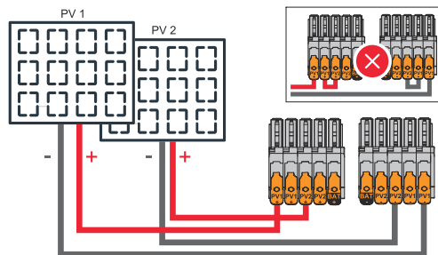
PV 1 kleiner/gleich 41,25 A ( I_{SC\ PV1} ) PV 2 kleiner/gleich 22 A ( I_{SC\ PV2} )
