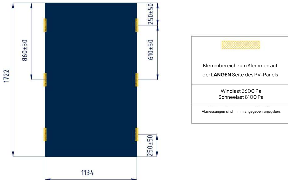
Abbildung 6: Befestigung von „BLACKSTAR B.108“ Modulen mit sechs Befestigungspunkten entlang der langen Seiten des Moduls
