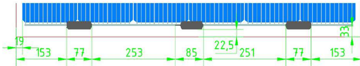
Abbildung 14: Position der Anschlussdose bei Modulen der „SOLID“ Serie
