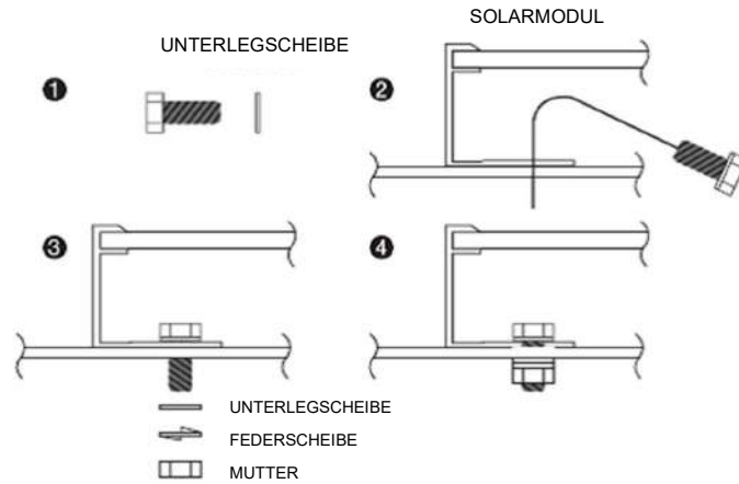
Abbildung 11: Befestigung mit Schrauben an den Querträgern.
