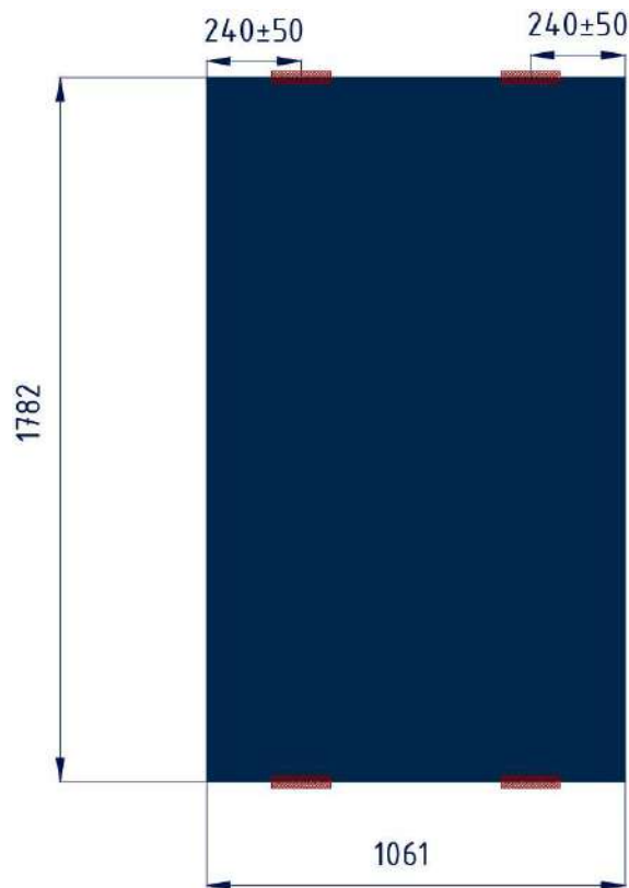
Abbildung 10: Montage von „BLACKSTAR B.60(40)“ Modulen mit vier Befestigungspunkten entlang der kurzen Seiten des Moduls
