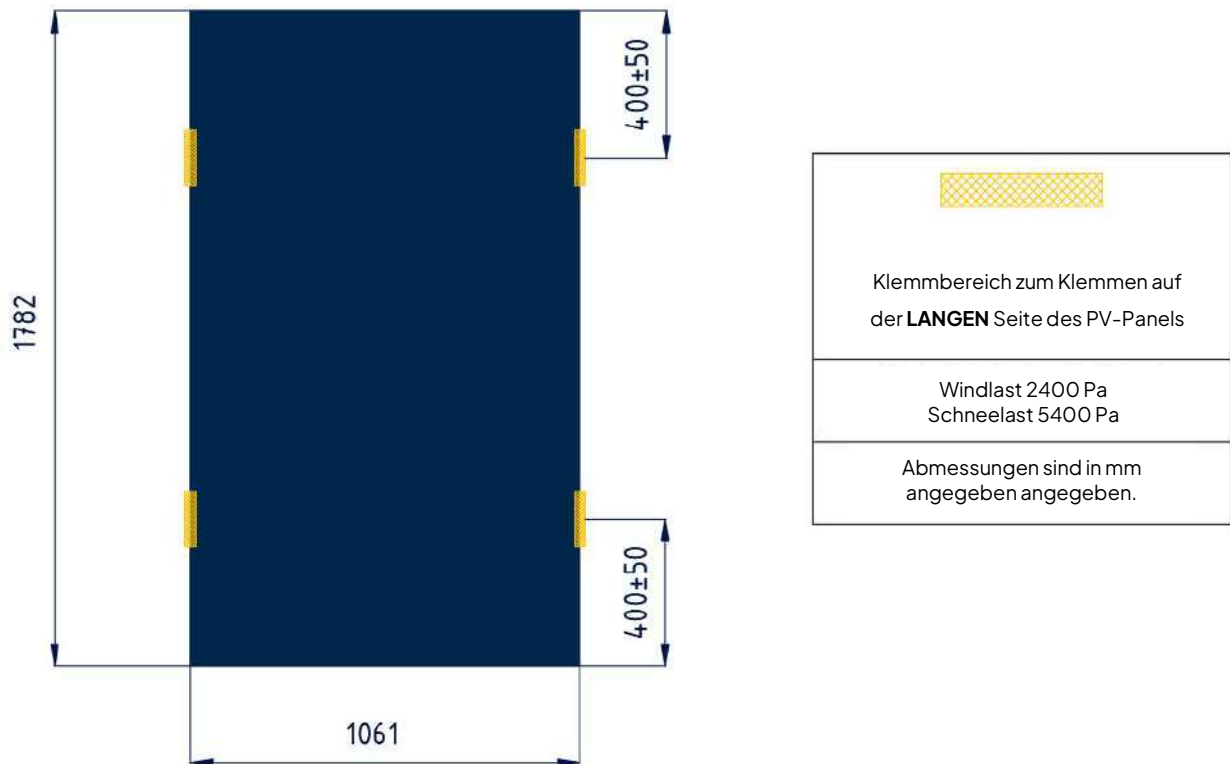
Abbildung 8: Montage von „Blackstar B.60(40)“ Modulen mit Klemmen an vier Befestigungspunkten entlang der langen Seiten des Moduls
