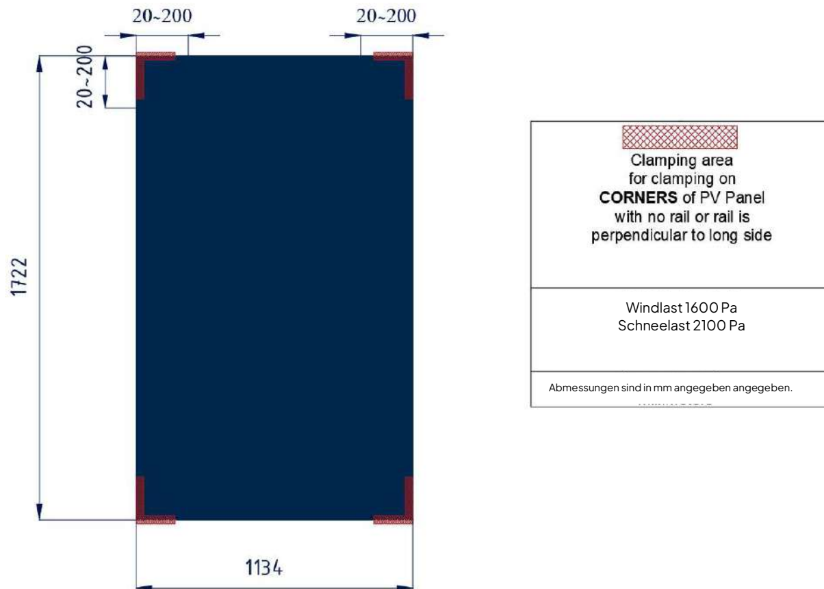
Abbildung 7. Blackstar B.108 Befestigung mit Klemmen, Verwendung von vier Befestigungspunkten an den Ecken des Moduls
