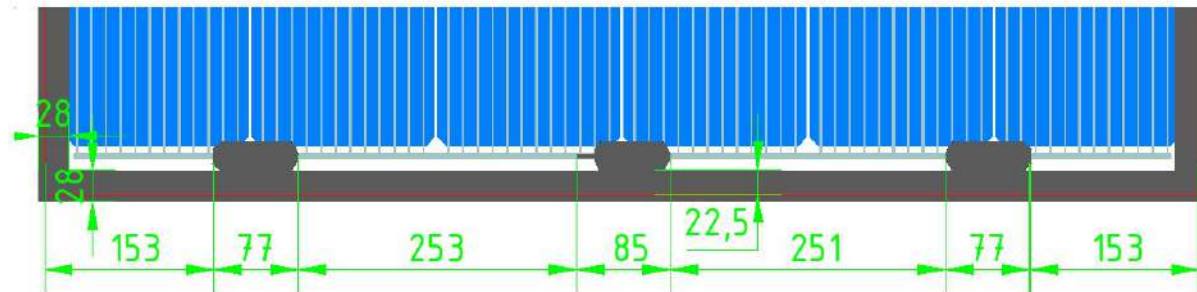
Abbildung 15: Position der Anschlussdose bei Modulen der „Blackstar B.60(40) (SOLID Framed)“ Serie
