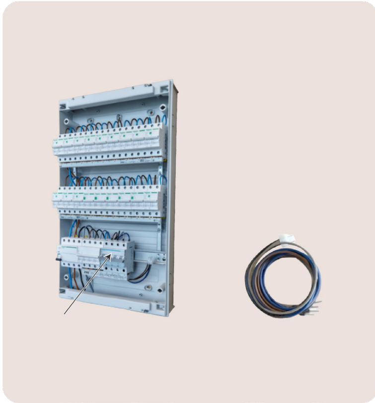
Abbildung 3: Blick auf eine Verteilertafel und das Stromversorgungskabel
