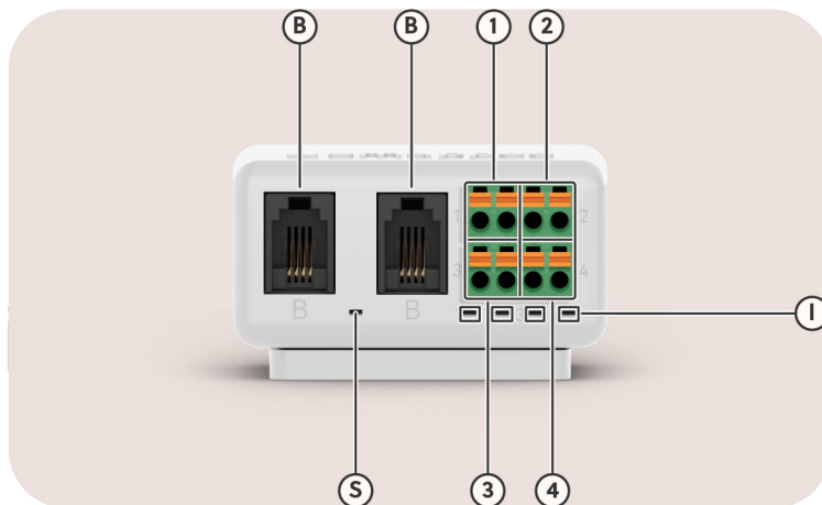
Abbildung 11: Ansicht auf ein Input Modul
