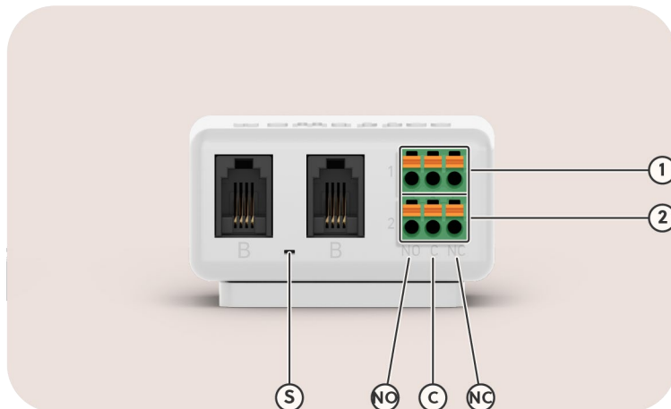
Abbildung13: Blick auf ein Output Modul
