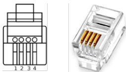
Abbildung 18: Stecker
