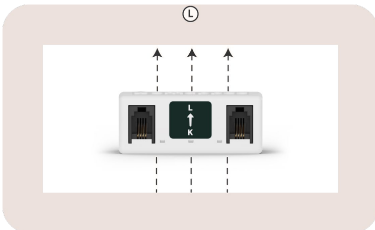
Abbildung 7: Ansicht auf den Pfeil auf einem Solid Core CT
