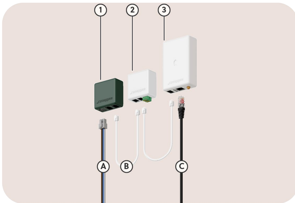
Abbildung 12: Schematische Darstellung des Smappee B-Bus-Stromkreises
