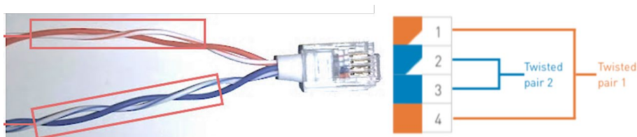
Abbildung 17: Verdrillte Paare
