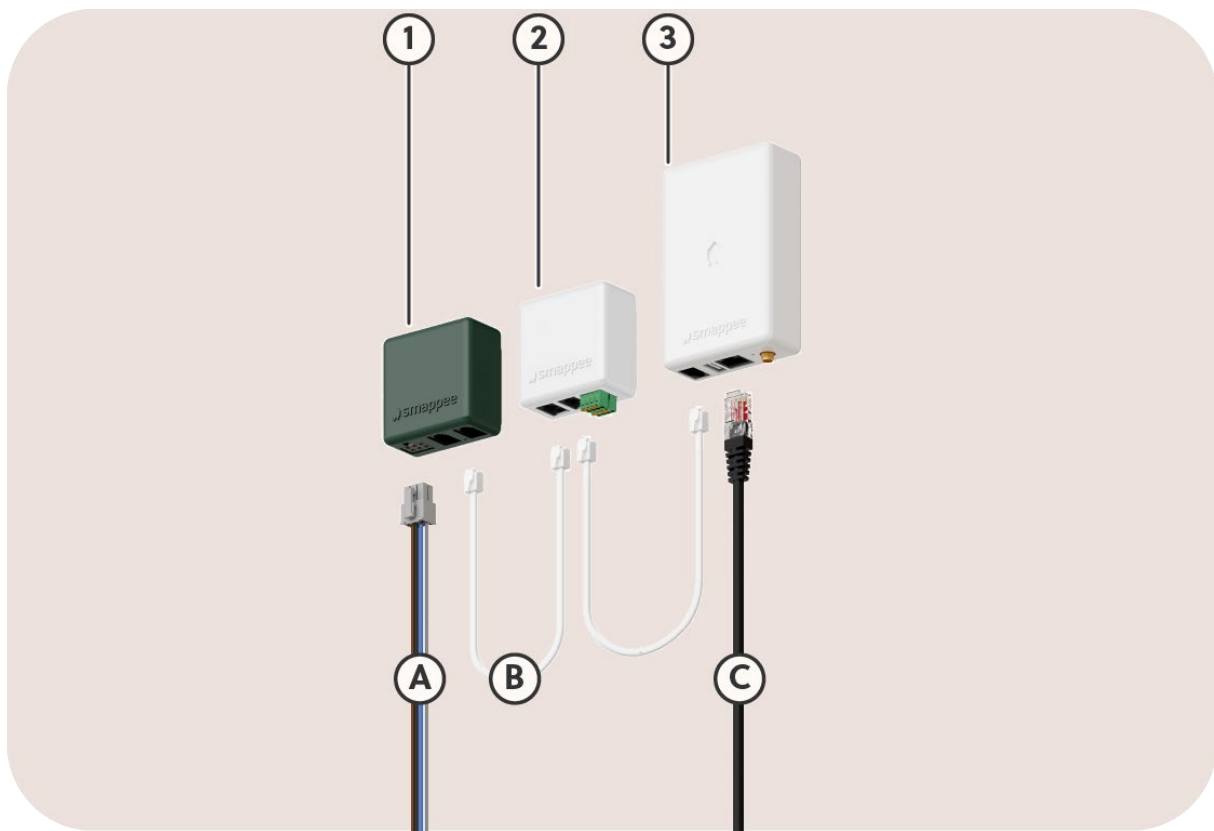
Abbildung 14: Schematische Darstellung des Smappee B-Busses.
