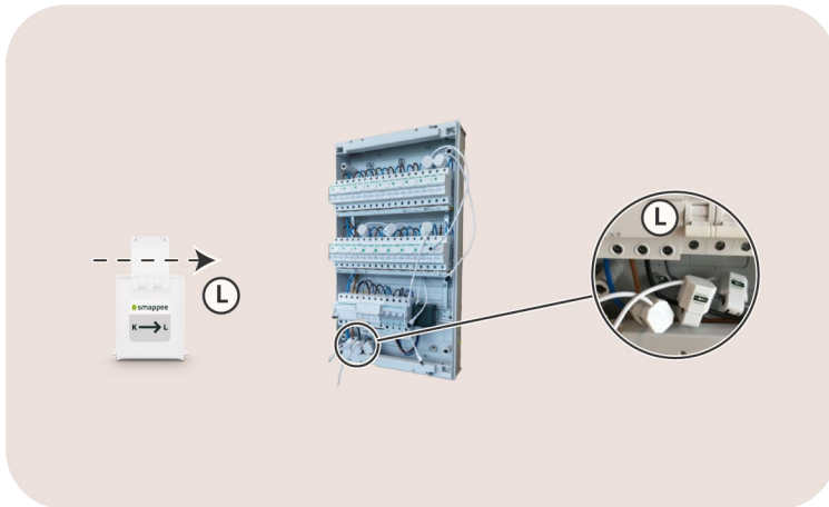
Abbildung 5: Ansicht des Pfeils auf einem Stromwandler und dessen Installation im Netzverteiler
