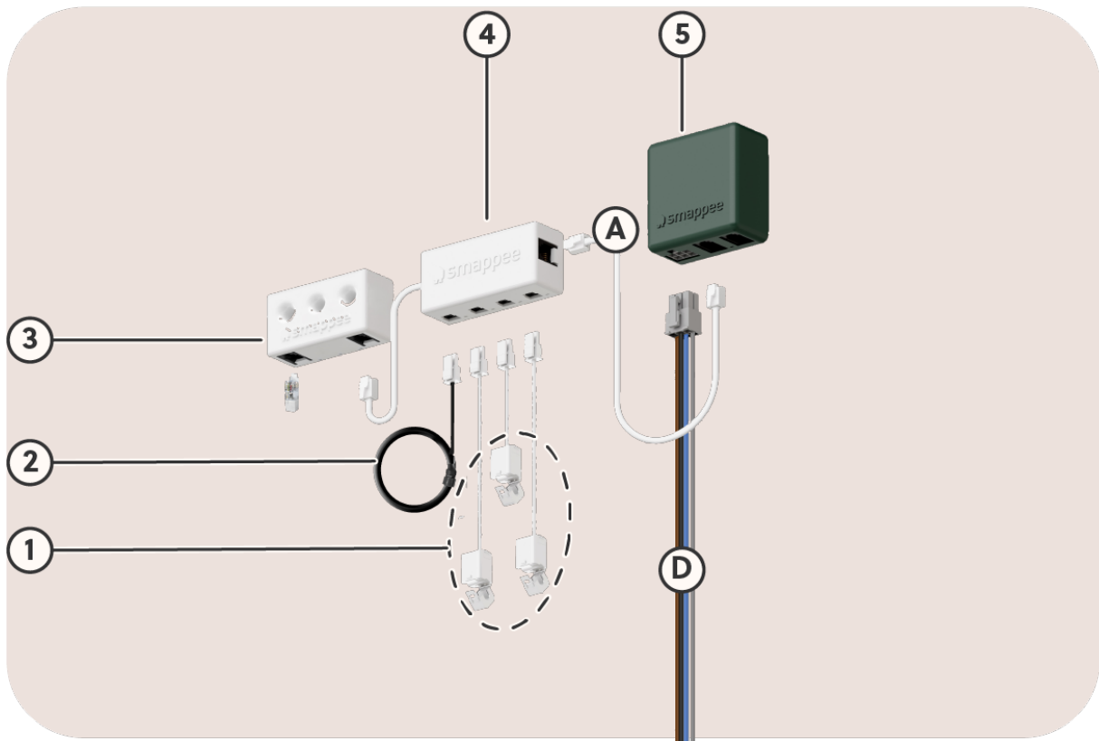
Abbildung 8: Schematische Darstellung des Smappee A-Bus-Stromkreises
