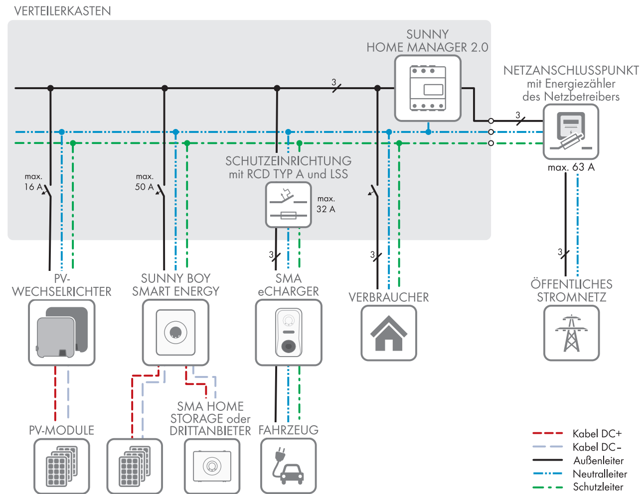
Abbildung 6: Verschaltungsübersicht (Beispiel mit 1 EVC22-3AC-20)
