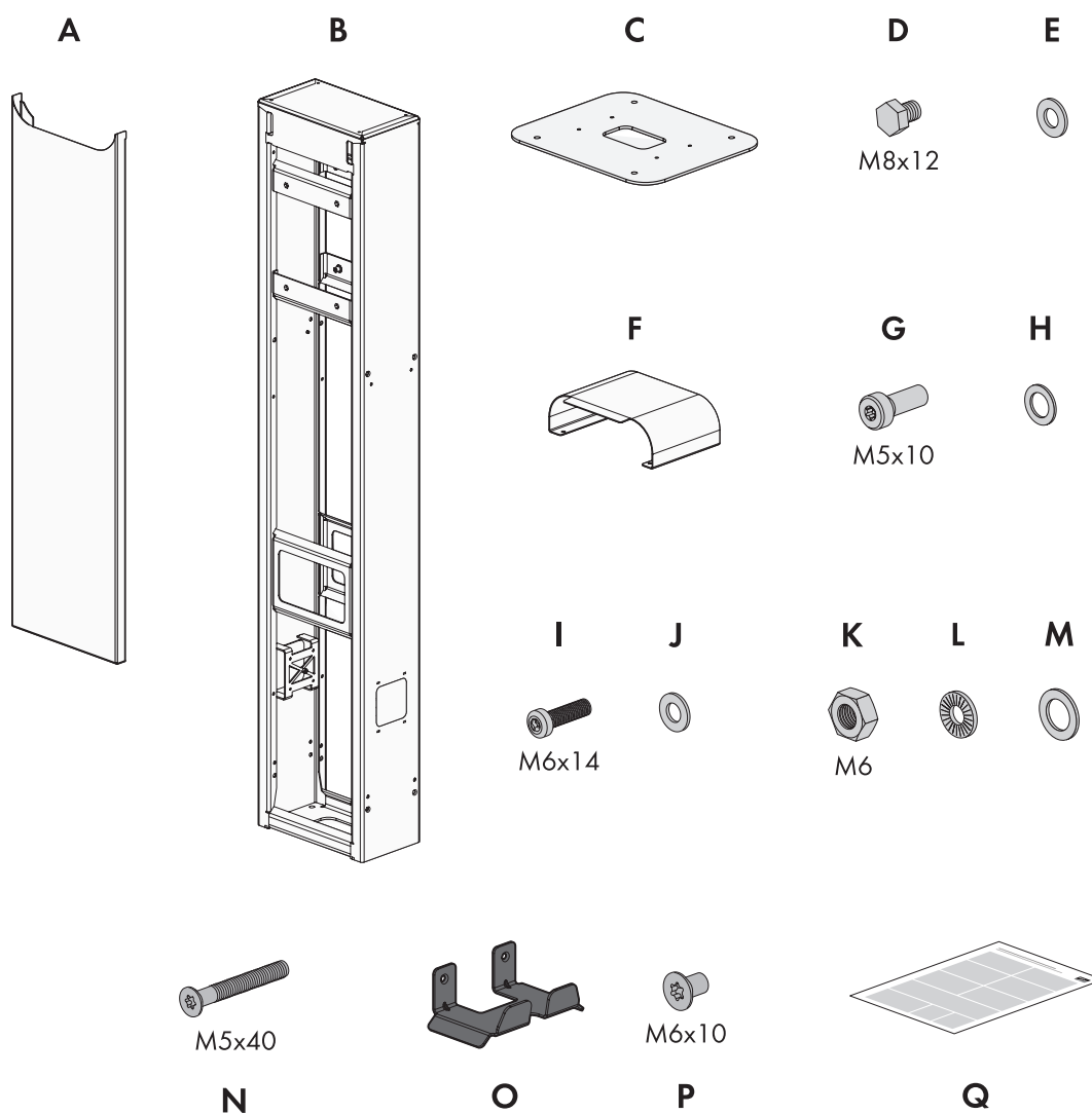
Abbildung 3: Bestandteile des Lieferumfangs
