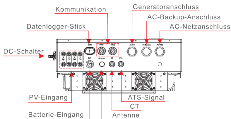
Abbildung 1.2 Seitenansicht von unten
