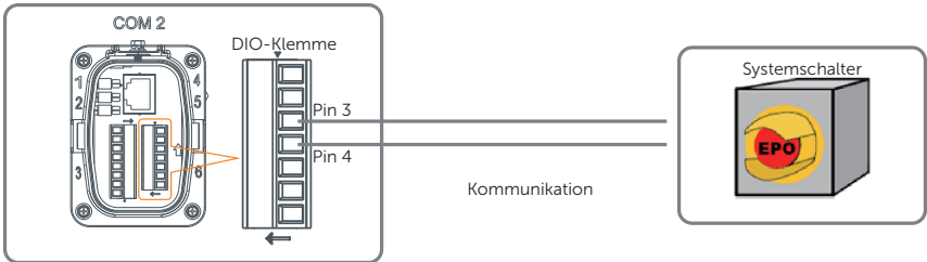
Abbildung 8-63 Anschlussplan für Systemschalter
