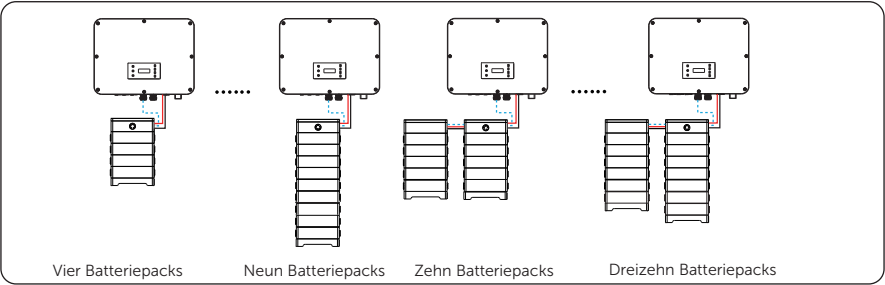
Abbildung 8-23 Batterie-Anschlussplan 1
