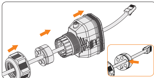
Abbildung 8-44 Kabel einfädeln
