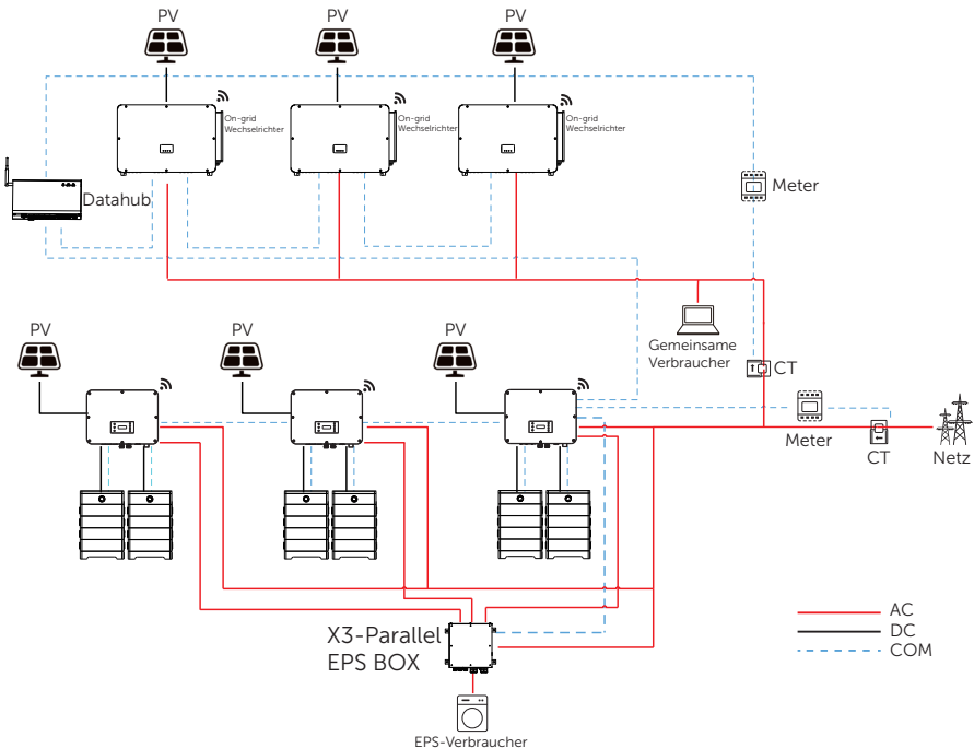
Abbildung 15-10 Schaltplan von DataHub
