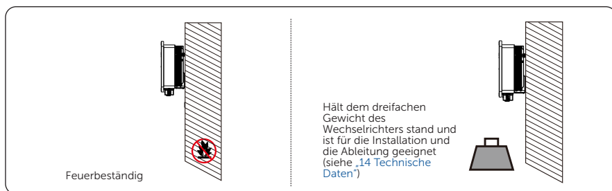
Abbildung 5-3 Anforderung an den Installationsträger
