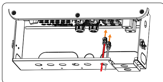
Abbildung 15-32 Batteriestromkabel anschließen
