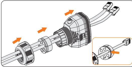
Abbildung 8-37 Kabel einfädeln
