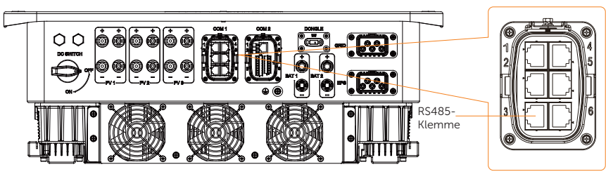
Abbildung 15-5 Anschlussklemme für Adapter Box
