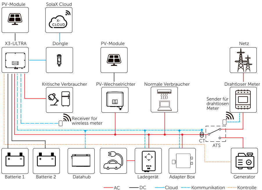
Abbildung 3-17 System-Übersichtsdiagramm
