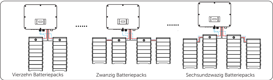
Abbildung 8-25 Batterie-Anschlussplan 2
