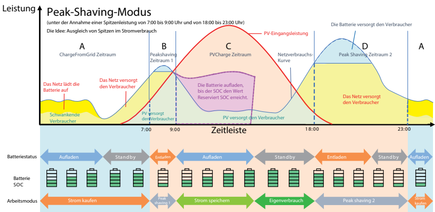
Abbildung 2-13 Peak-Shaving-Modus
