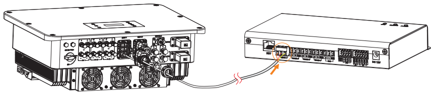
Abbildung 15-12 An Datahub anschließen
