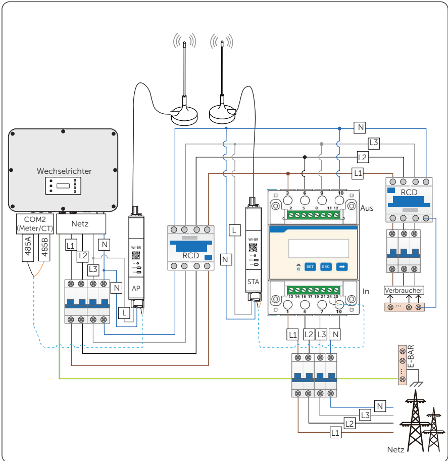
Abbildung 8-50 Anschlussplan für drahtloses Meter
