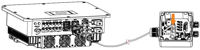
Abbildung 15-6 An die Adapterbox anschließen
