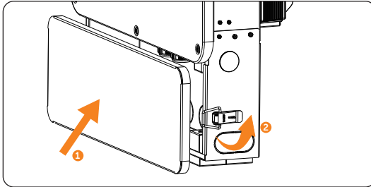
Abbildung 15-38 Frontplatte installieren
