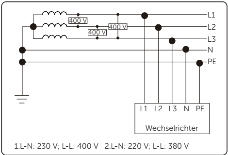
Abbildung 2-3 Unterstütztes Stromnetz-TN-S
