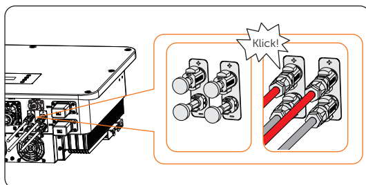
Abbildung 8-34 Batterie-Steckverbinder anschließen
