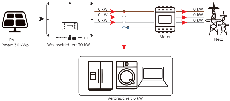
Abbildung 2-16 Null-Exportkontrolle bei aktivierter Phasenunsymmetrie
