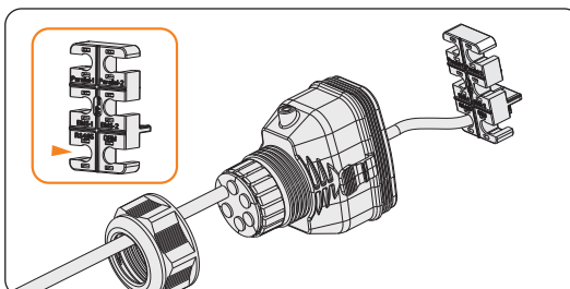
Abbildung 8-45 RJ45-Klemme an dem Kabelhalter anbringen
