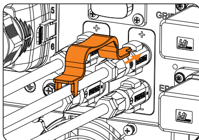
Abbildung 13-4 Batterie-Steckverbinder entfernen
