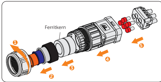
Abbildung 8-9 AC-Steckverbinder demontieren
