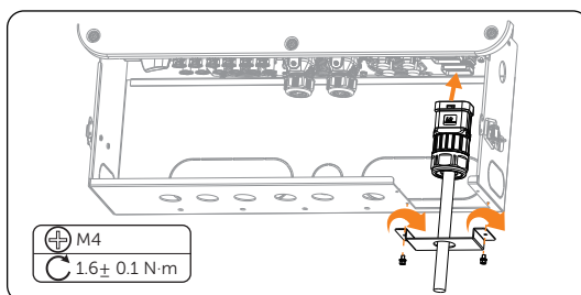
Abbildung 15-30 AC-Steckverbinder installieren
