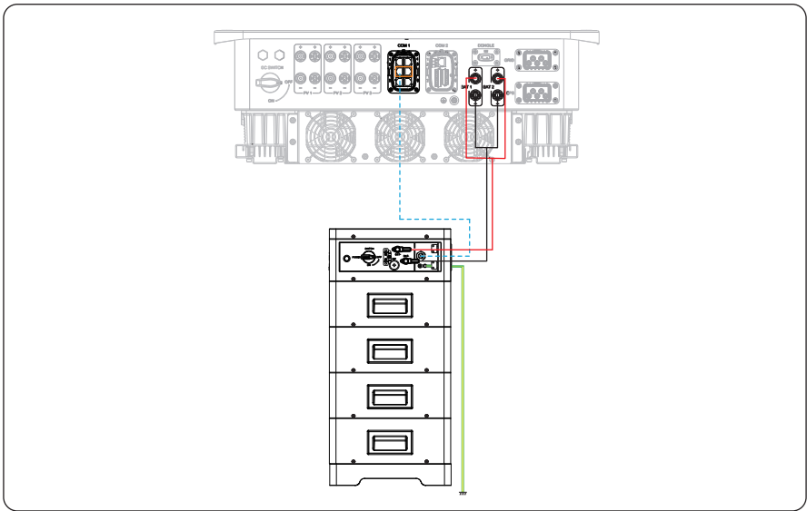
Abbildung 8-28 Detaillierter Anschlussplan 3
