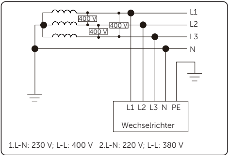
Abbildung 2-2 Unterstütztes Stromnetz-TT
