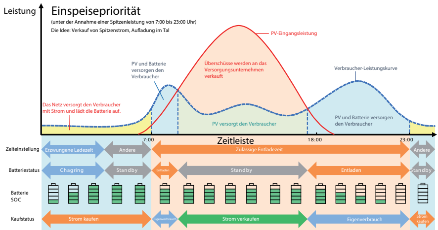
Abbildung 2-11 Einspeisepriorität
