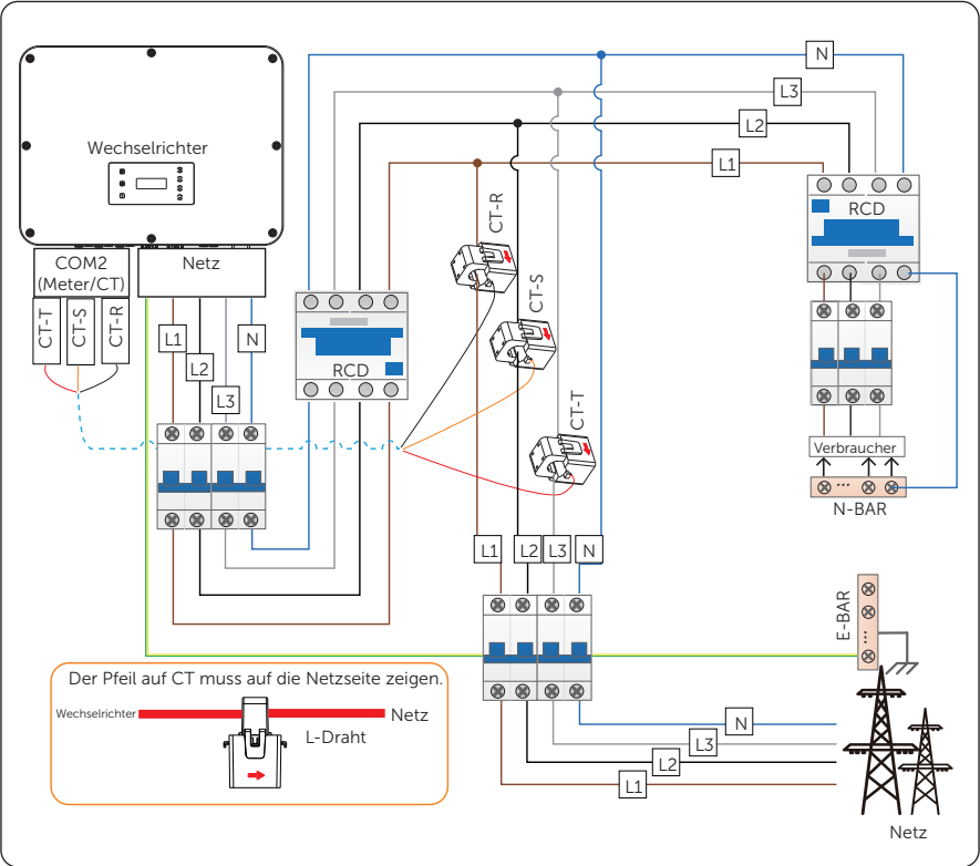
Abbildung 8-51 CT-Anschlussplan
