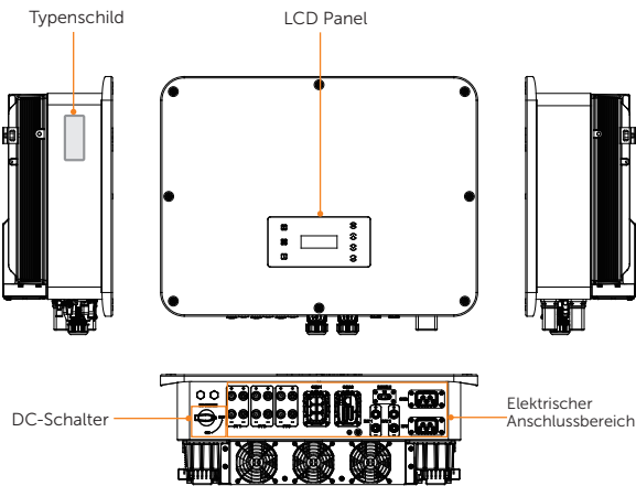
Abbildung 2-1 Erscheinungsbild
