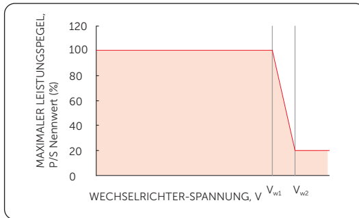
Abbildung 10-77 Kurve für P(u)
