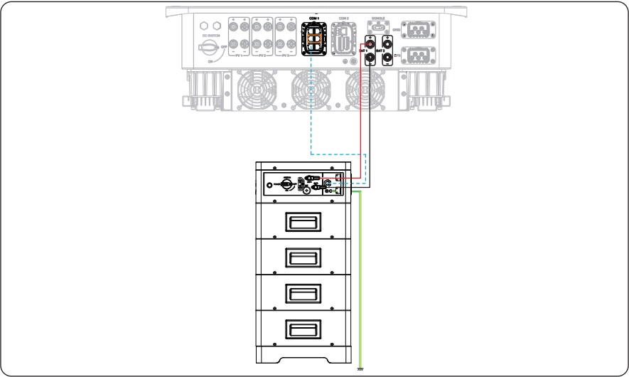
Abbildung 8-24 Detaillierter Anschlussplan 1
