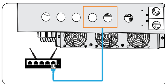
Abbildung 15-37 Dongle installieren
