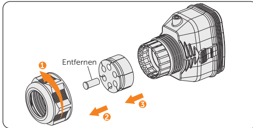
Abbildung 8-43 Den Steckverbinder demontieren
