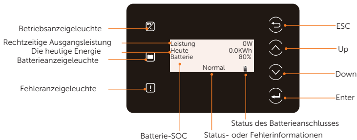
Abbildung 10-72 Bedienfeld
