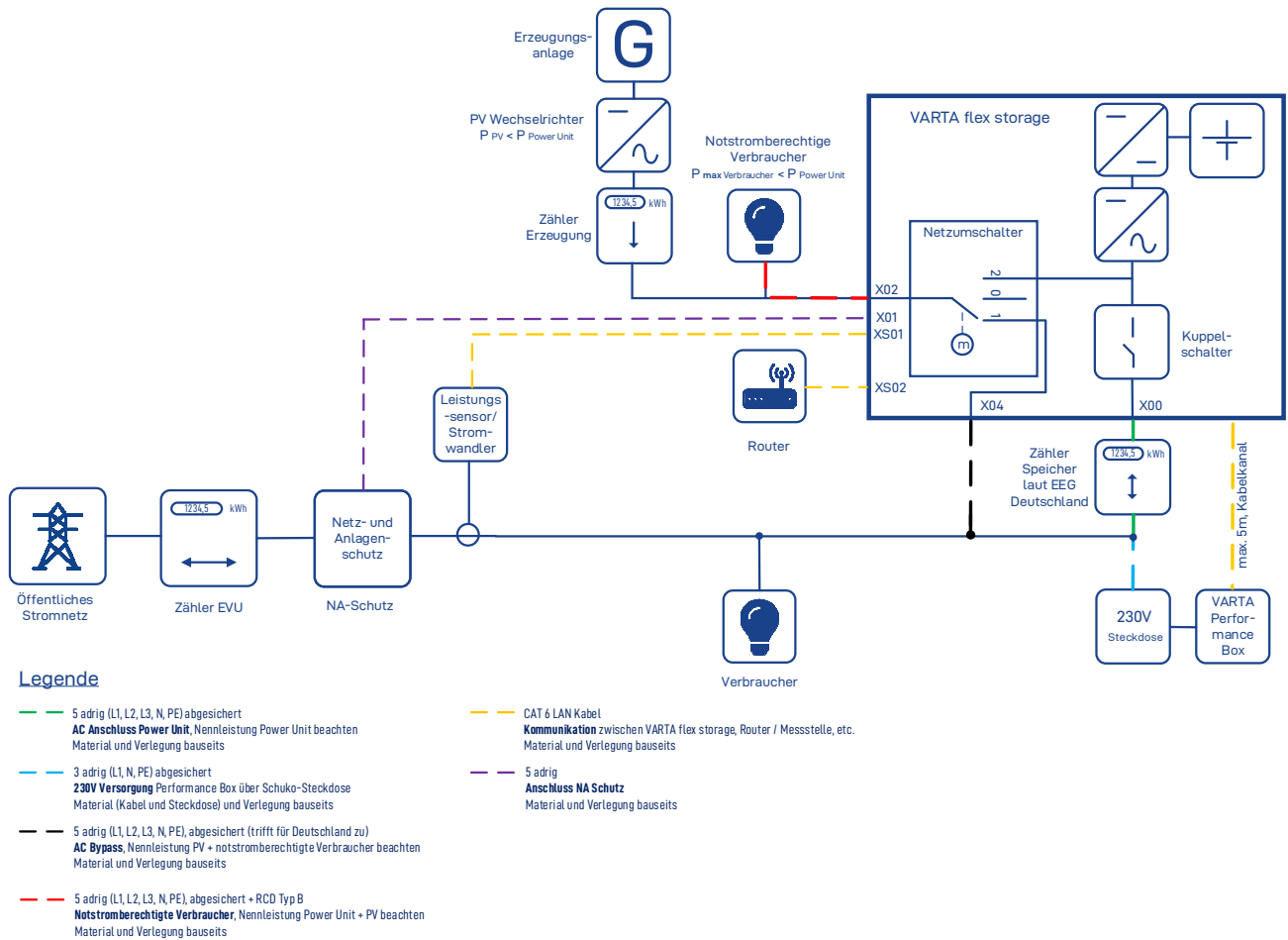
Abbildung 2: Schnittstellen - PV Eigenverbrauch mit Notstromfunktion
