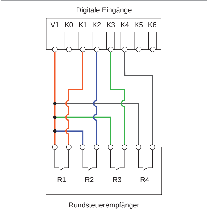
Anschlussschema für einen Rundsteuerempfänger
