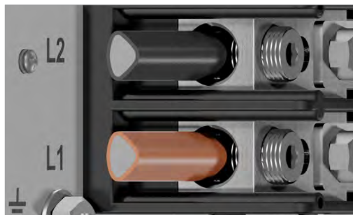
Korrekte Lage von sektorförmigen Aluminiumkabeln (2)
