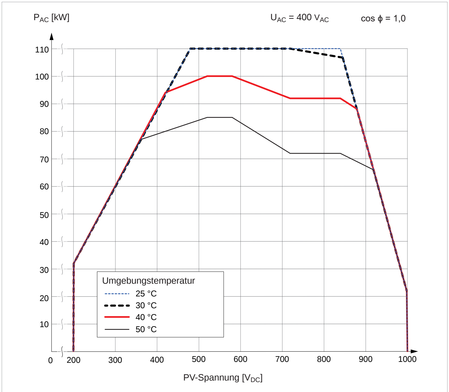
Kennlinie „Wirkleistungsregelung in Abhängigkeit von der PV-Spannung; cos \phi = 1,0; AC-Spannung = 400 V AC “
