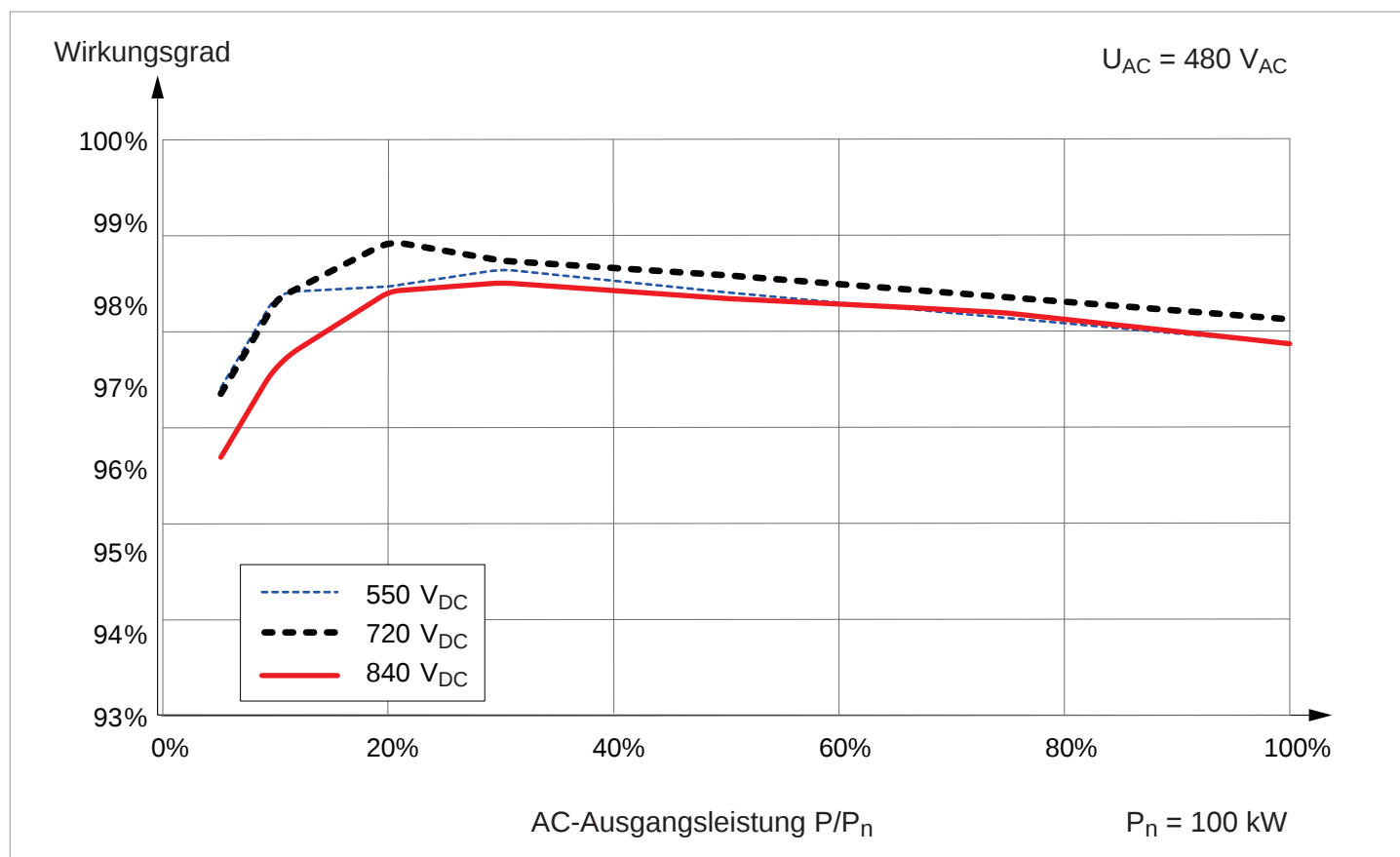
Wirkungsgrad-Kennlinie; AC-Spannung = 480 V_{AC}
