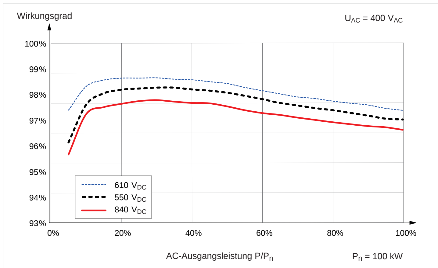
Wirkungsgrad-Kennlinie; AC-Spannung = 400 V_{AC}
