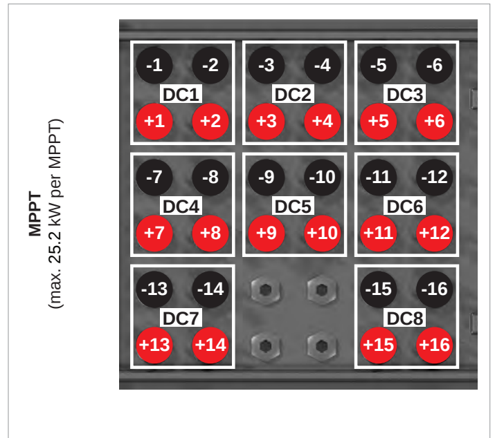
Anordnung der DC-Eingänge am DC-Anschlussfeld
