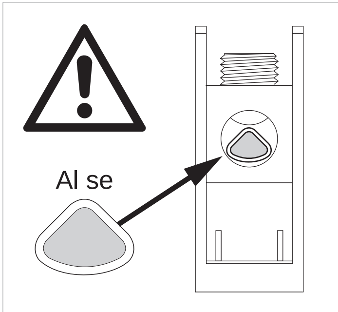
Abb. 8.11: Korrekte Lage von sektorförmigen Aluminiumkabeln (1)
