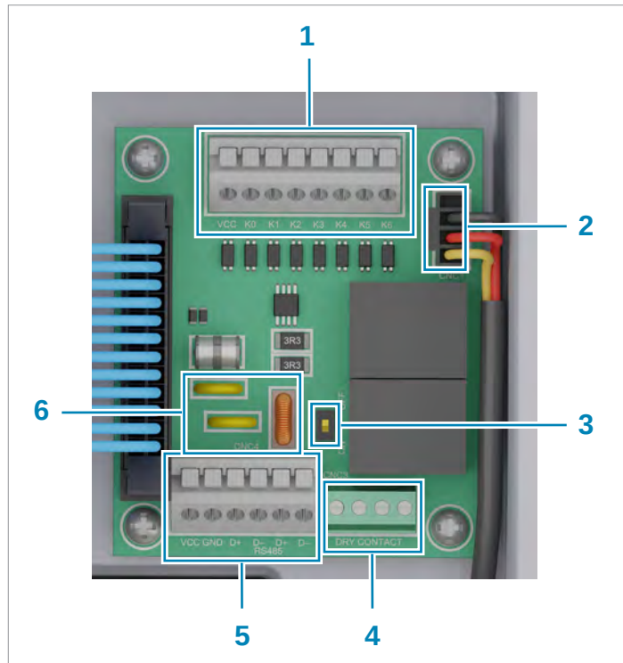
Abb. 5.25: Komponenten der Kommunikationskarte
