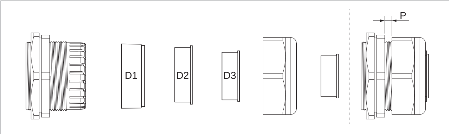
Abb. 8.15: Verwendung der Teile der AC-Kabelverschraubung in Abhängigkeit vom Kabeldurchmesser
