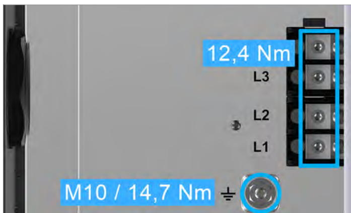
Abb. 8.9: Drehmomente für AC-Klemmenblock
