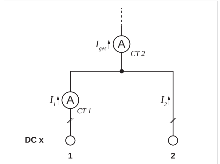
Abb. 6.23: Anordnung der Stromsensoren eines DC-Eingangs
