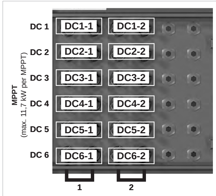
Abb. 6.22: Anordnung der DC-Eingänge am DC-Anschlussfeld
