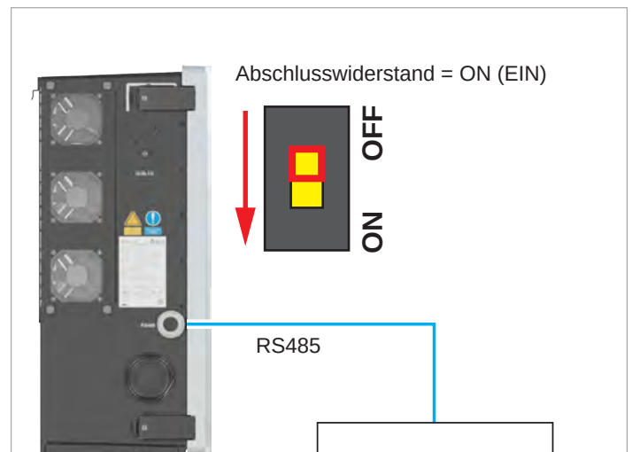
Abb. 8.2: RS485-Anschlusschema für einen einzelnen Wechselrichter
