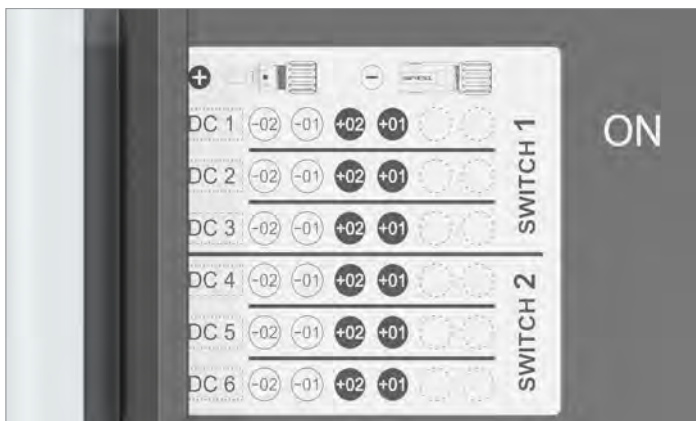
Abb. 4.8: Etikett mit der Zuordnung der einzelnen DC-Steckverbinder
