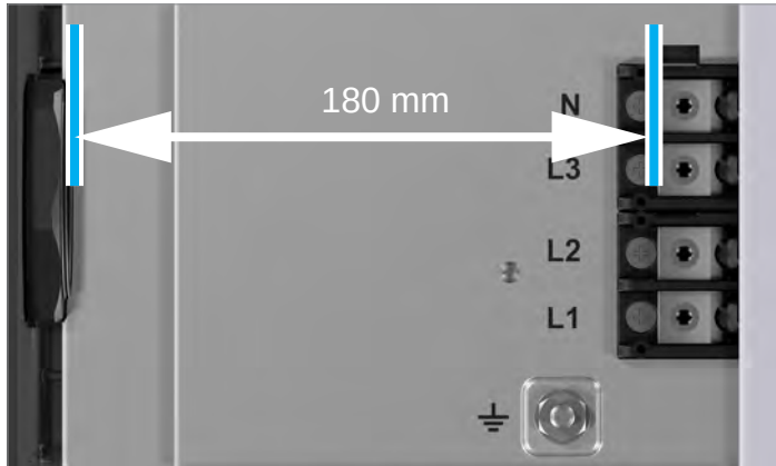
Abb. 8.8: Freiraum für Verdrahtung am AC-Klemmenblock
