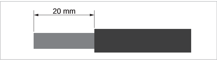
Abb. 6.17: Abisolierlänge bei AC-Kabeln
