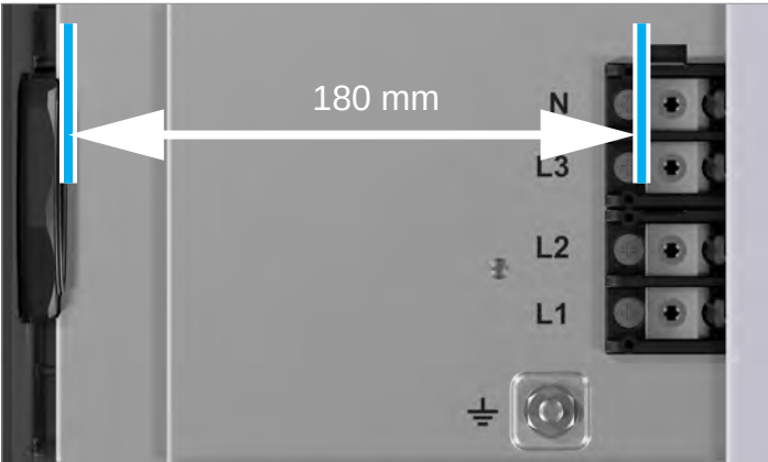
Abb. 6.16: Freiraum für Verdrahtung am AC-Klemmenblock
