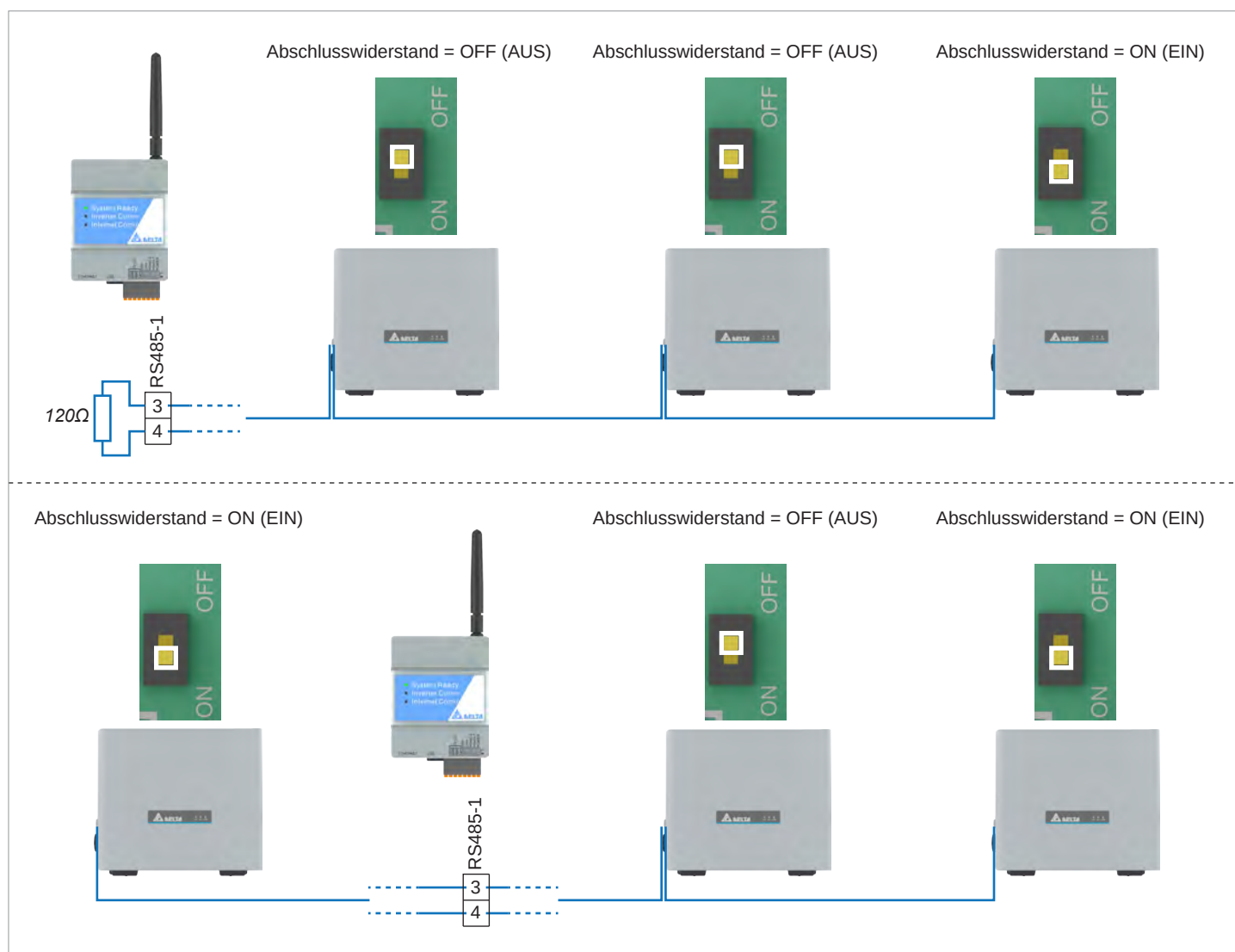
Abb. 5.26: RS485-Anschlussschema für einen DC1 Datenkollektor mit mehreren Wechselrichtern
