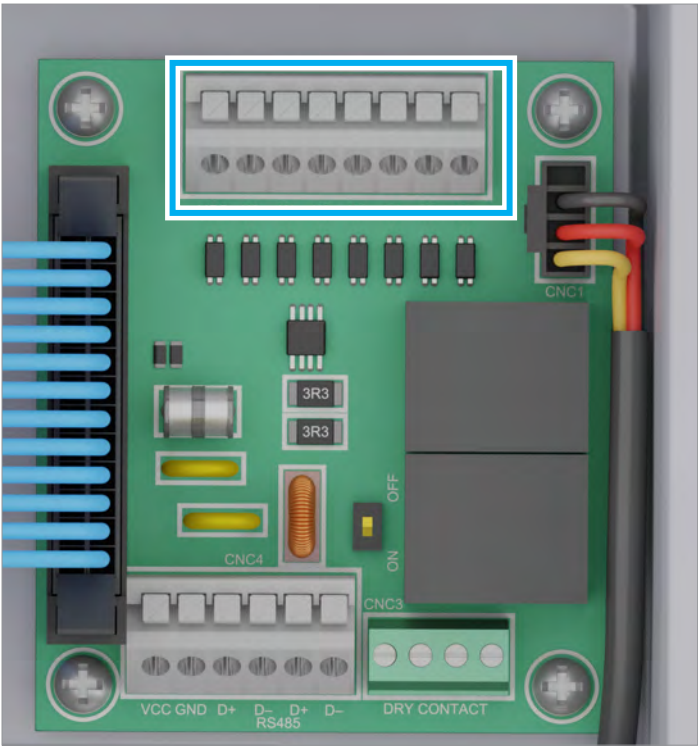
Abb. 5.27: Klemmenblock mit digitalen Eingängen
