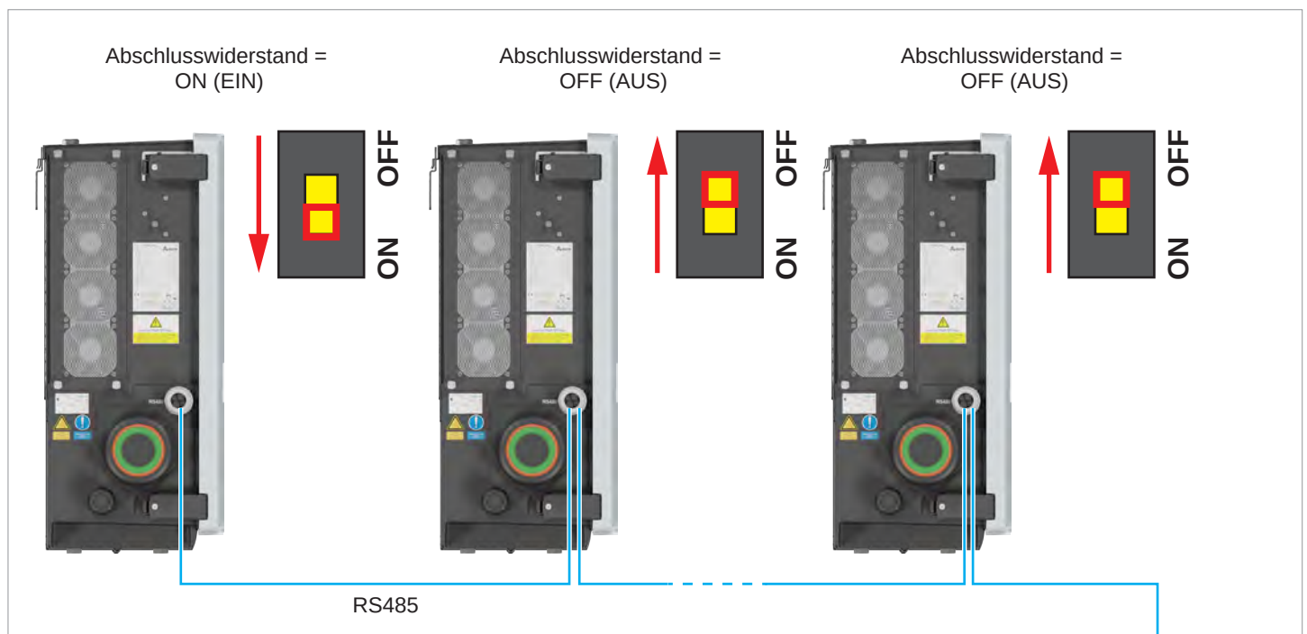
Abb. 8.3: RS485-Anschlussschema für mehrere Wechselrichter
