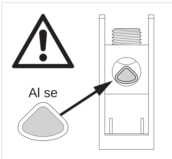
Abb. 6.18: Korrekte Lage von sektorförmigen Aluminiumkabeln (1)
