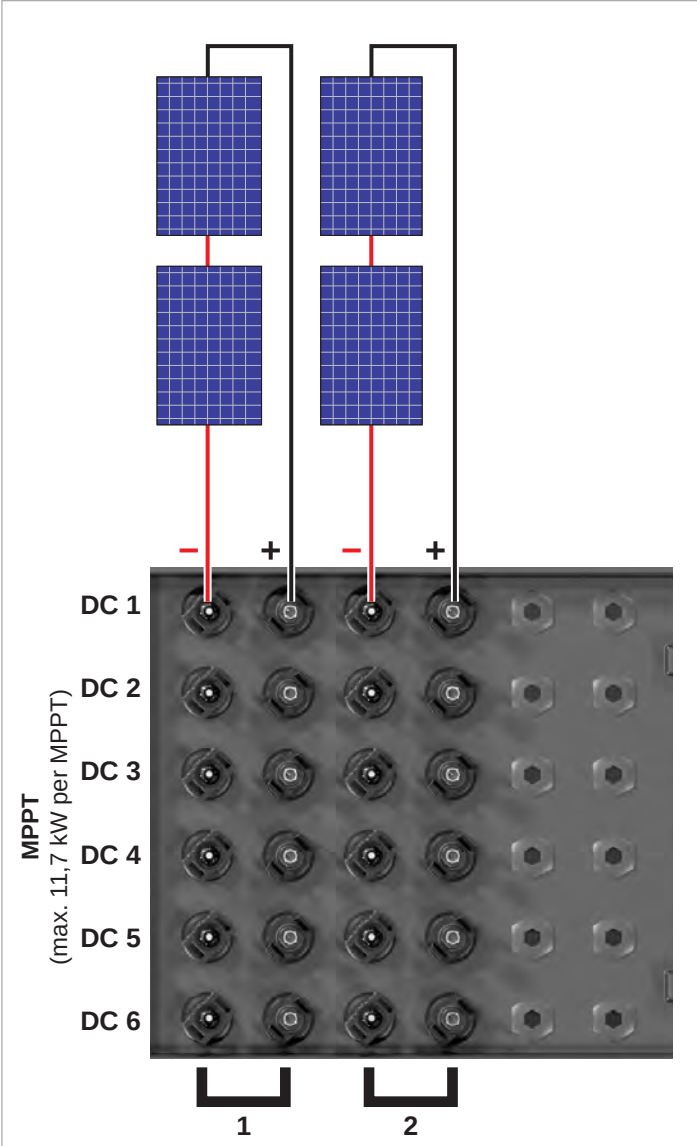
Abb. 6.24: Anschluss von 1 oder 2 Modulsträngen pro DC-Eingang (= MPP-Tracker): keine Strangsicherungen notwendig
