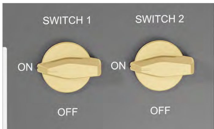
Abb. 4.11: Beide DC-Trennschalter in der Position ON (EIN) = die Verbindung zu den Solarmodulen ist geschlossen
