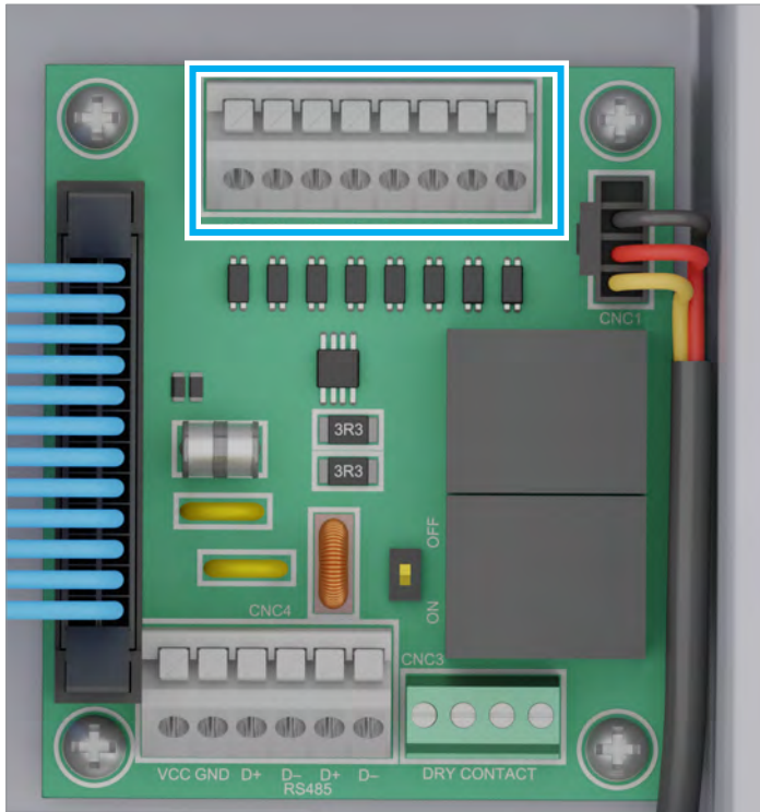
Abb. 5.28: Klemmenblock mit digitalen Eingängen
