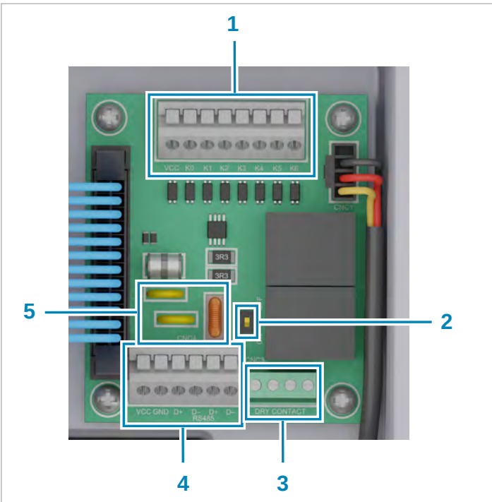
Abb. 4.14: Komponenten der Kommunikationskarte
