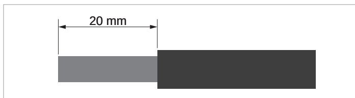
Abb. 8.10: Abisolierlänge bei AC-Kabeln
