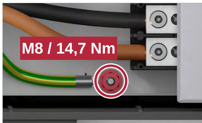
Drehmomente am PE-Anschluss
