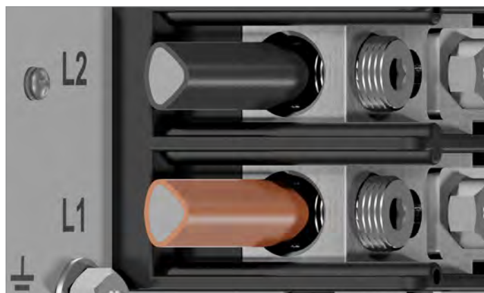
Korrekte Lage von sektorförmigen Aluminiumkabeln (2)
