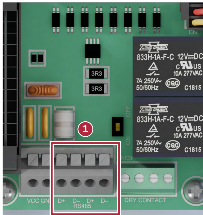
RS485 für den Anschluss eines Datenloggers
