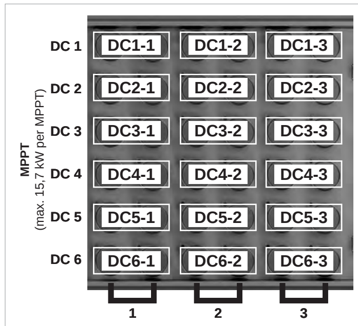
Anordnung der DC-Eingänge am DC-Anschlussfeld
