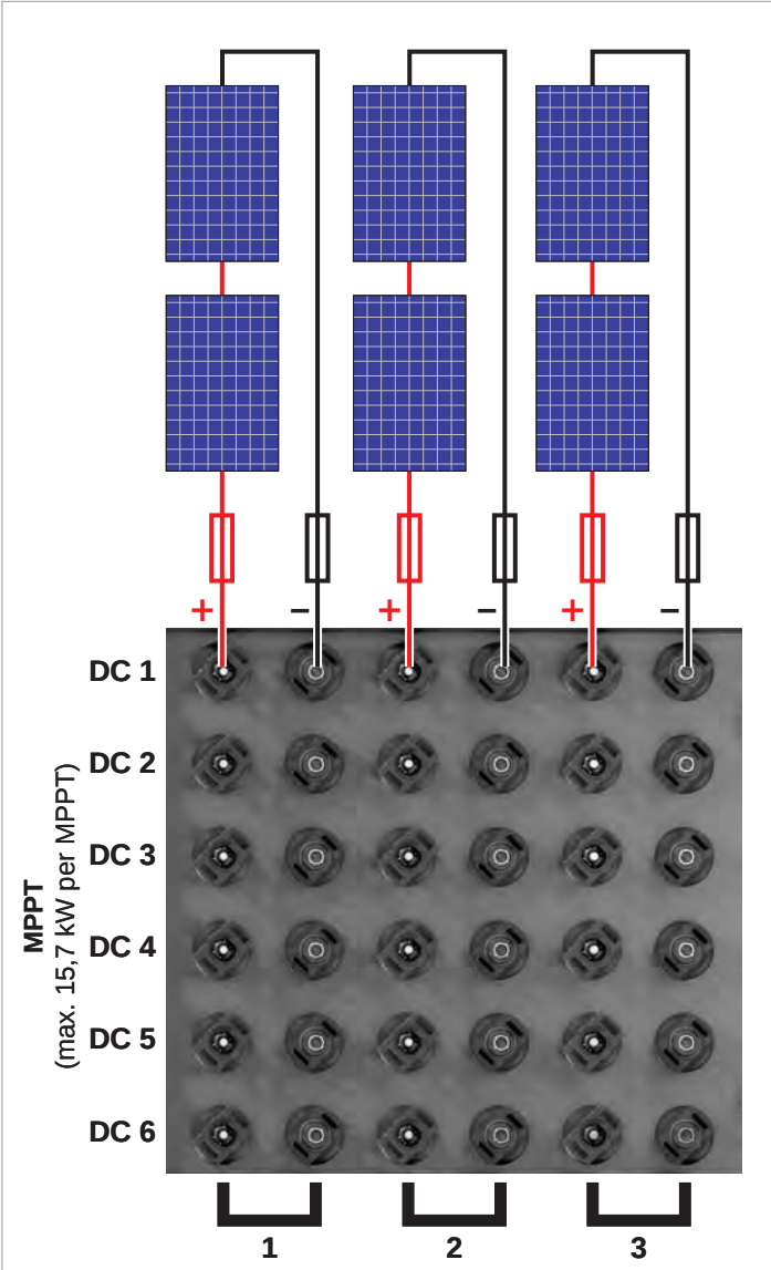
Anschluss von 3 Modulsträngen pro DC-Eingang (= MPP-Tracker): Strangsicherungen empfohlen
