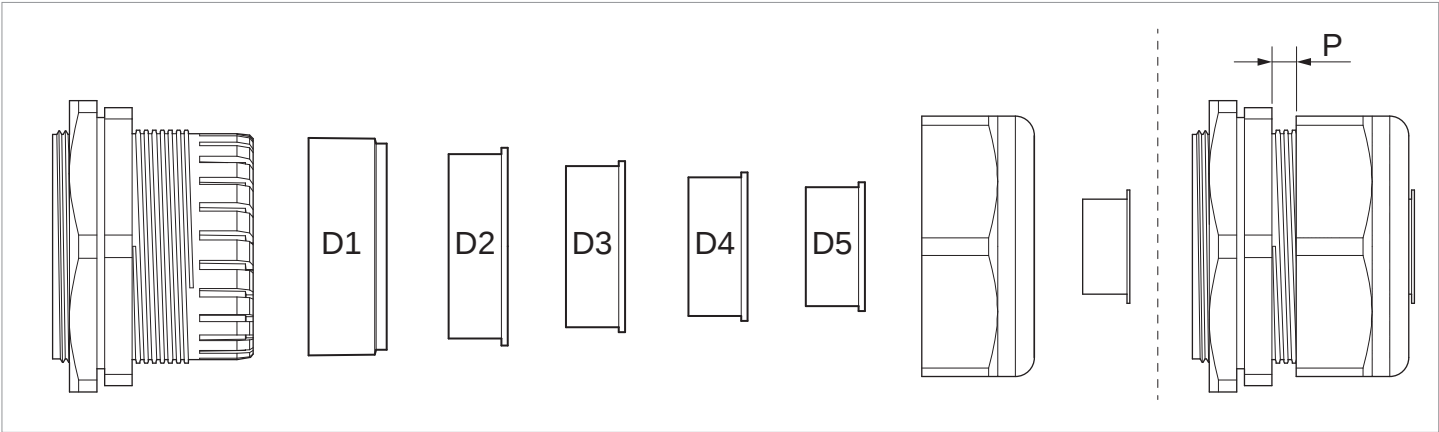
Verwendung der Teile der AC-Kabelverschraubung in Abhängigkeit vom Kabeldurchmesser
