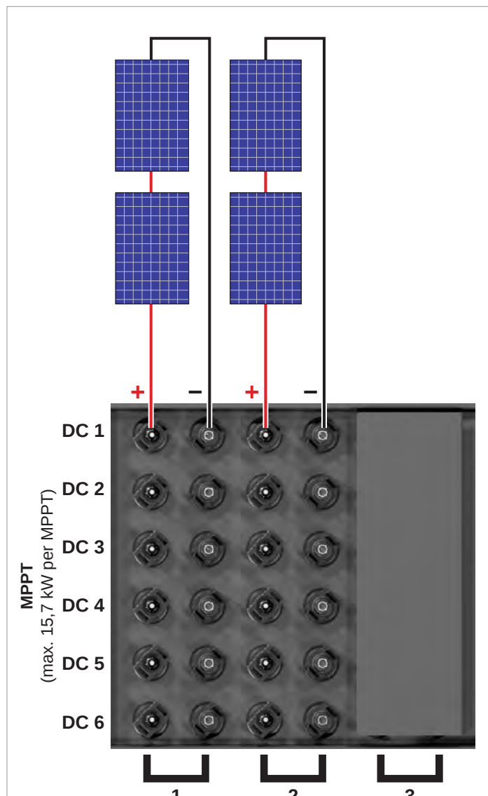
Beim Anschluss von 1 oder 2 Modulsträngen pro DC-Eingang (= MPP-Tracker) sind keine Strangsicherungen notwendig
