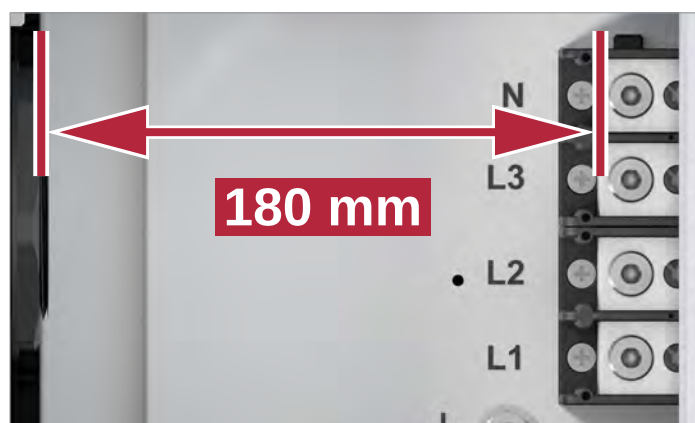
Freiraum für Verdrahtung am AC-Klemmenblock
