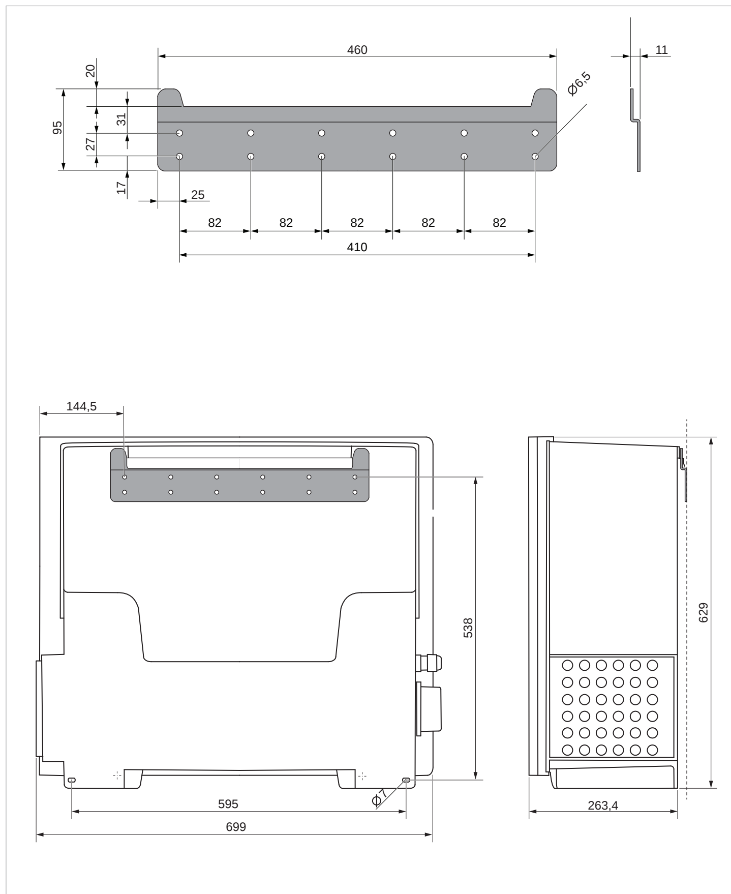
Abmessungen für die Wandmontage (Angaben in mm)
