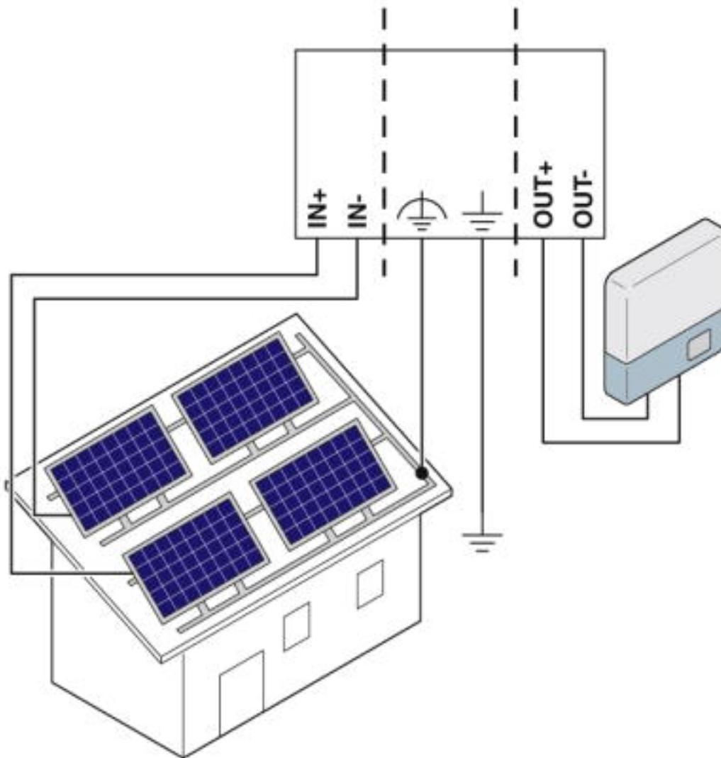
Schematische Applikationszeichnung
