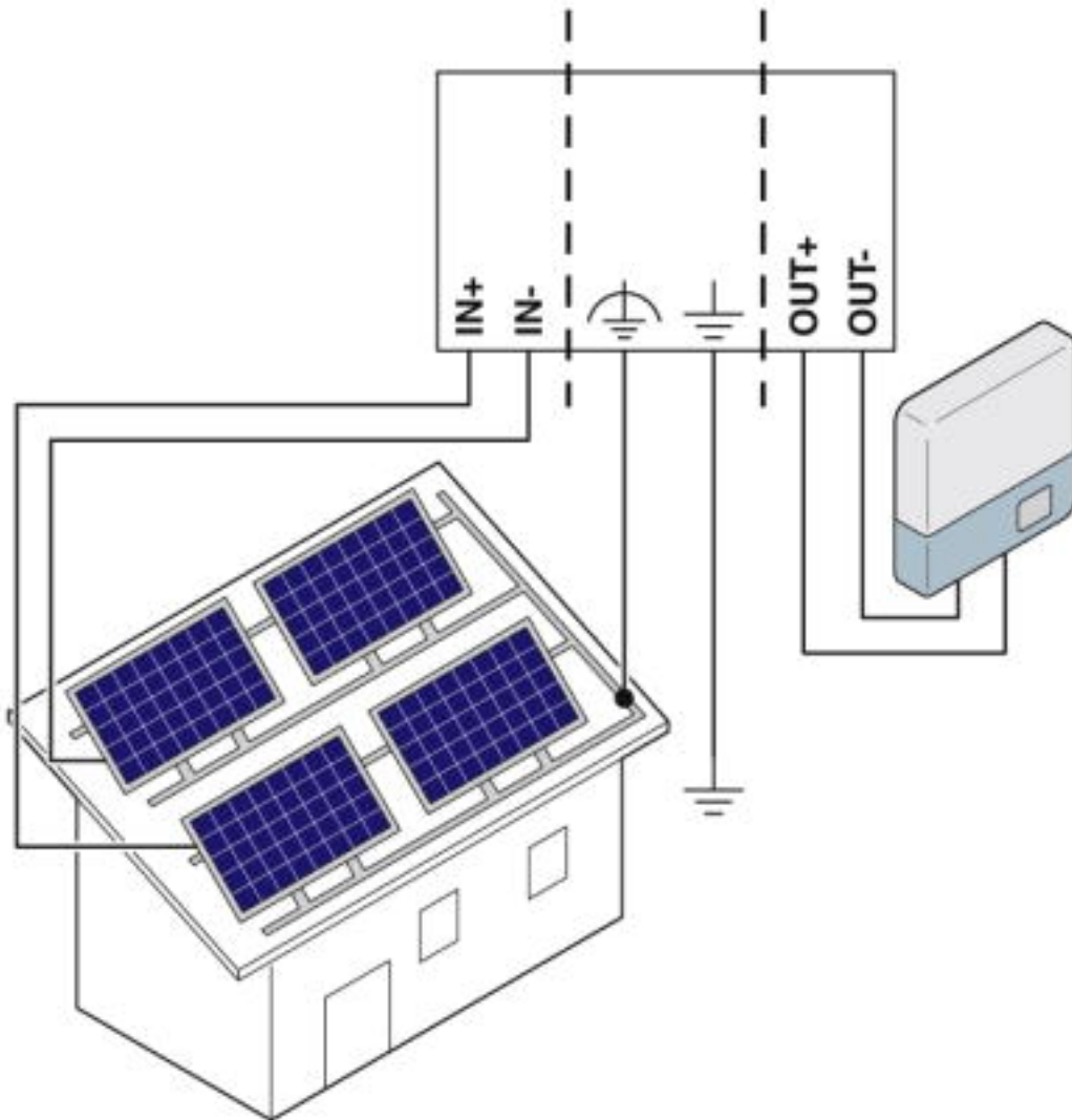
Schematische Applikationszeichnung
