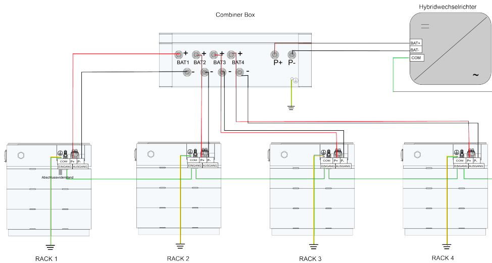
Abbildung 5-2 Diagramm Batteriekaskadierung
