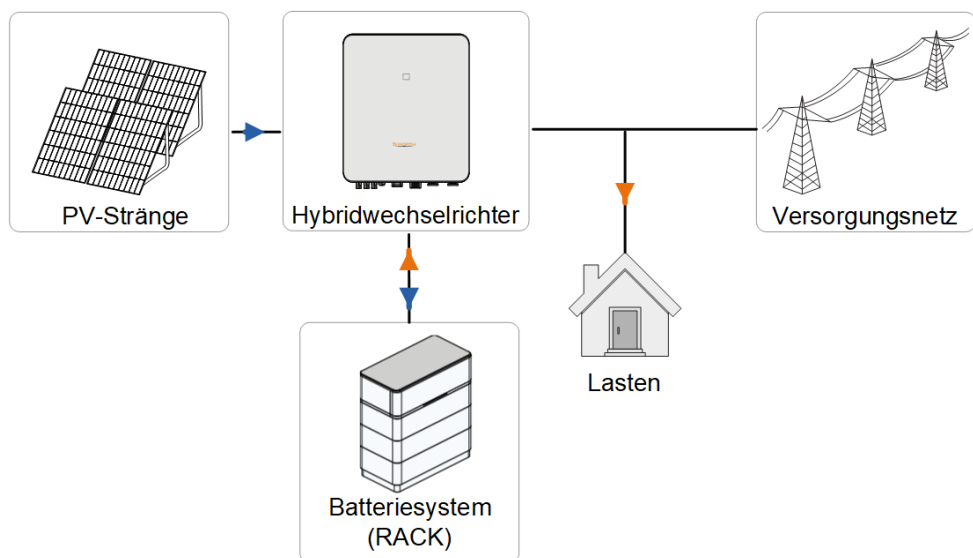
Abbildung 2-1 Systemschaltplan
