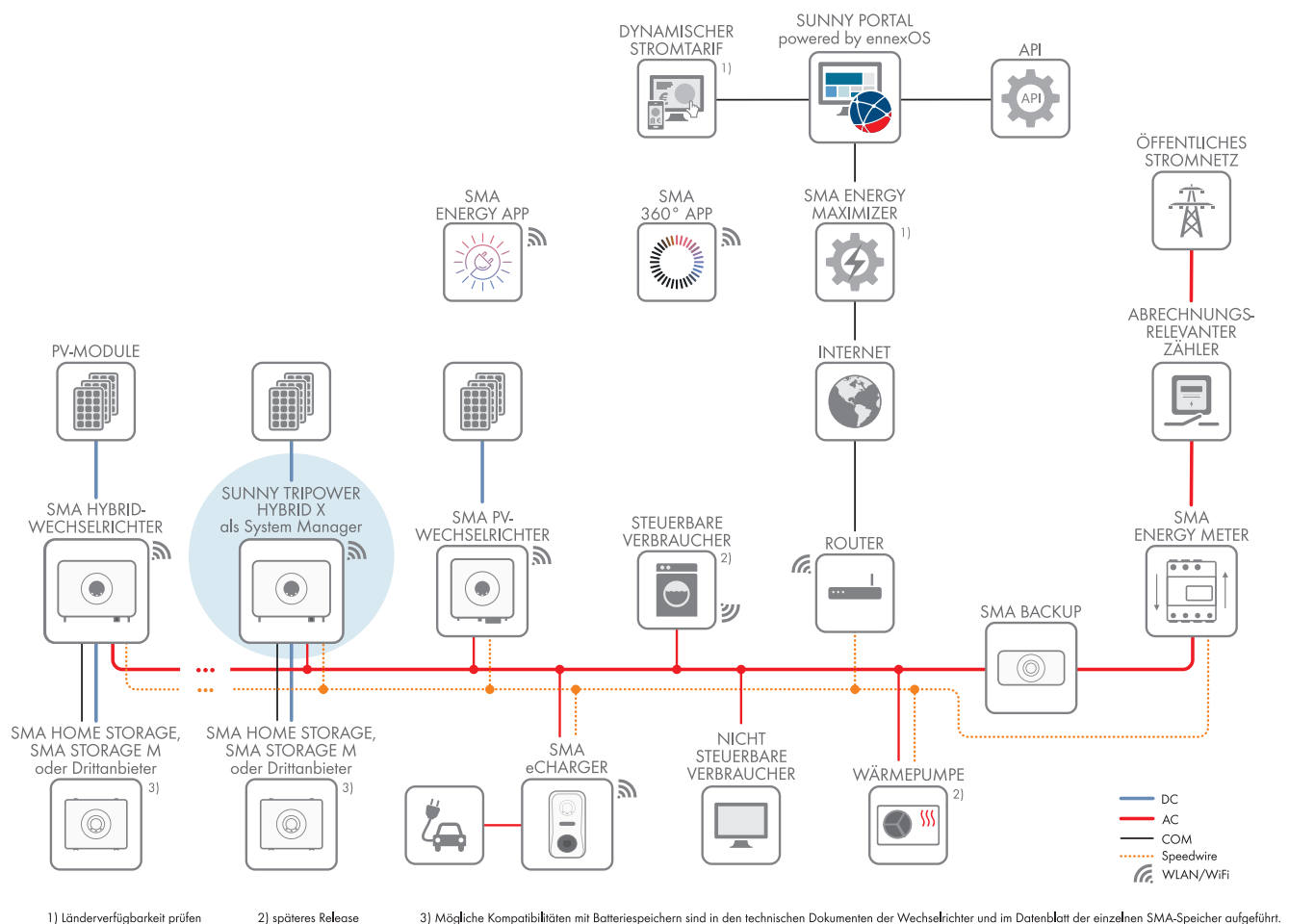
Abbildung 2: Systemübersicht mit Sunny Tripower Hybrid X (STPxx-70) als System Manager.
