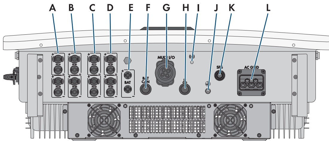
Abbildung 6: Unteransicht des Wechselrichters
