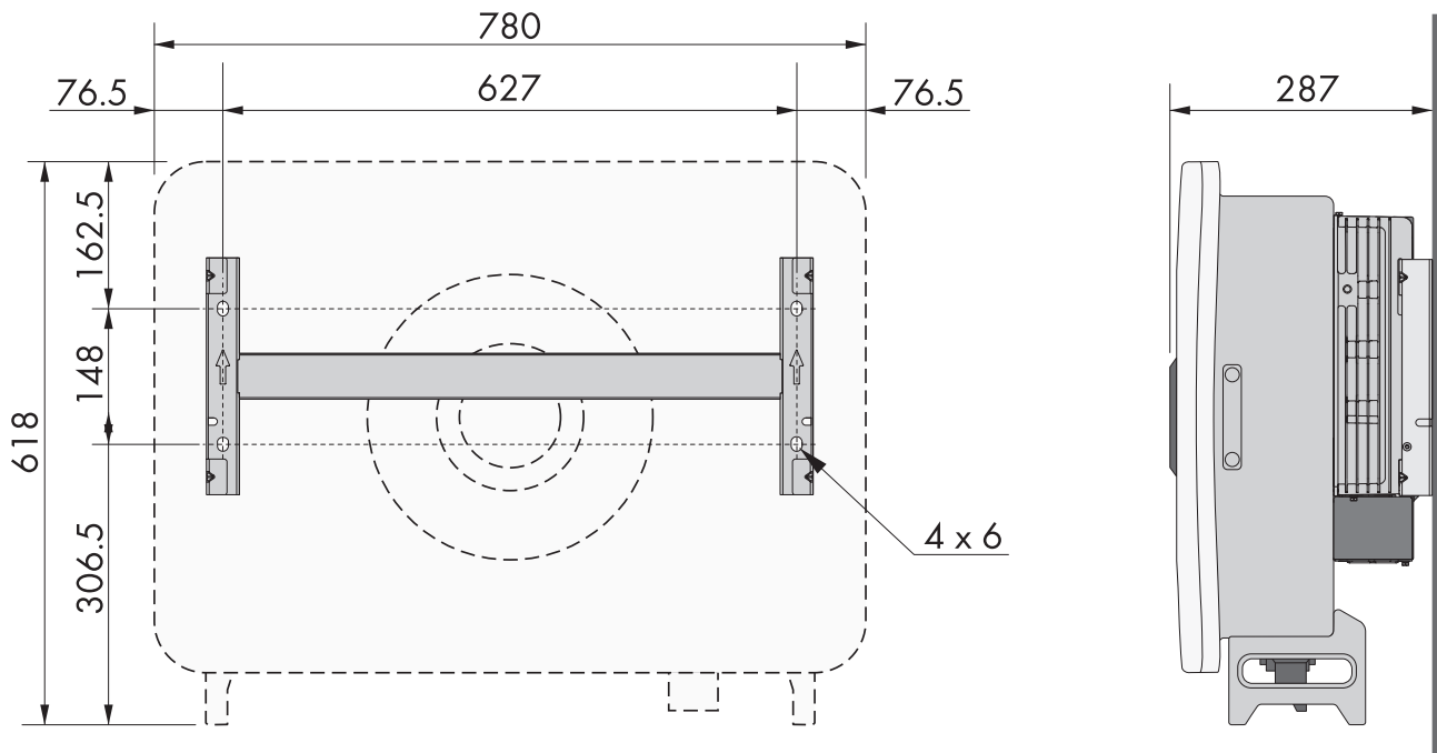
Abbildung 4: Position der Befestigungspunkte (Maßangaben in mm)
