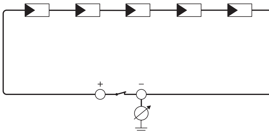
Abbildung 11: Schematische Darstellung der Messung
