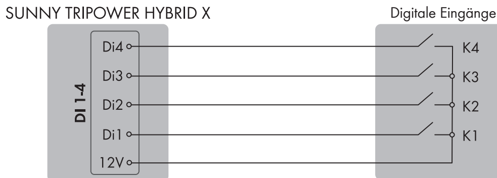
Abbildung 8: Anschluss eines Fernwirkgeräts am digitalen Eingang DI D1-D4, Vcc des Sunny Tripower Hybrid
