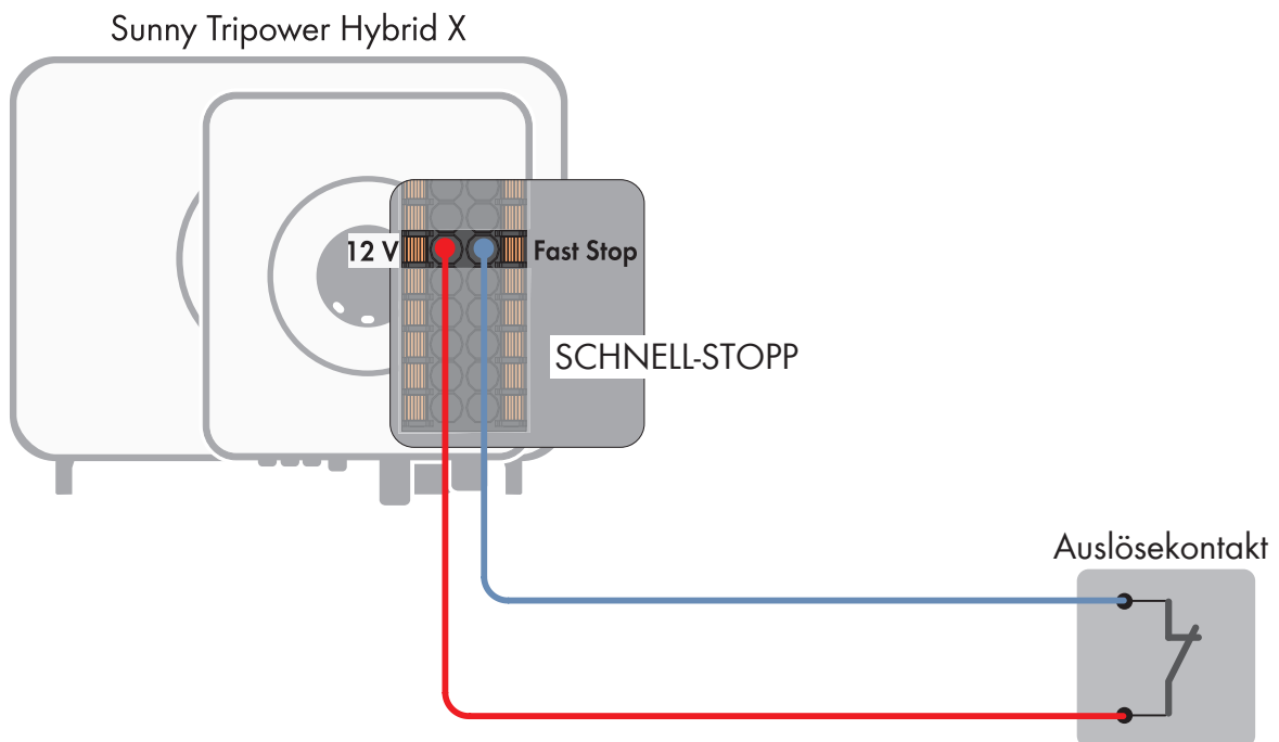
Abbildung 9: Beispiel der Verschaltung für den Anschluss eines Auslösekontakts für den Schnell-Stopp.
