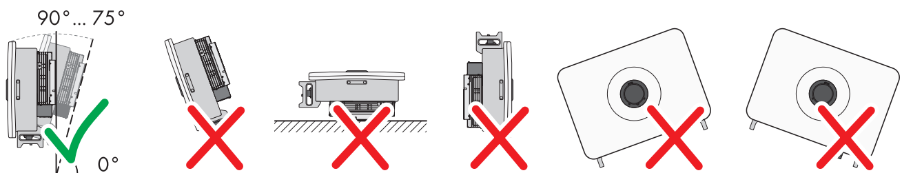
Abbildung 3: Zulässige und unzulässige Montagepositionen
