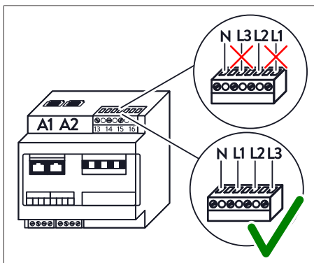
Abb. 8: Anschluss Spannungsmessung
