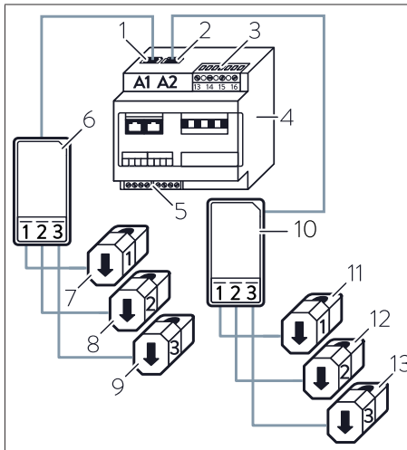
Abb. 7: Komponenten des Leistungsmessgeräts WM271
