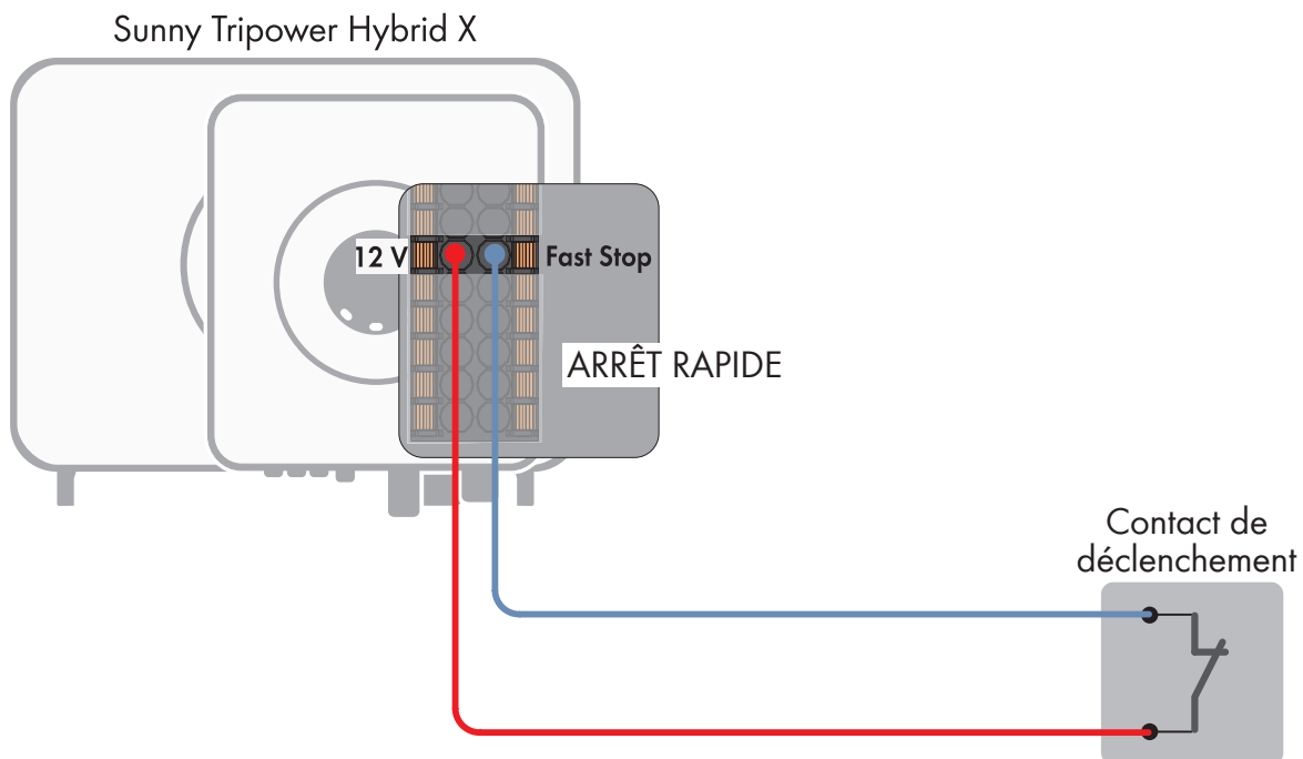
Figure 11 : Exemple de câblage pour le raccordement d'un contact de déclenchement pour l'arrêt rapide.
