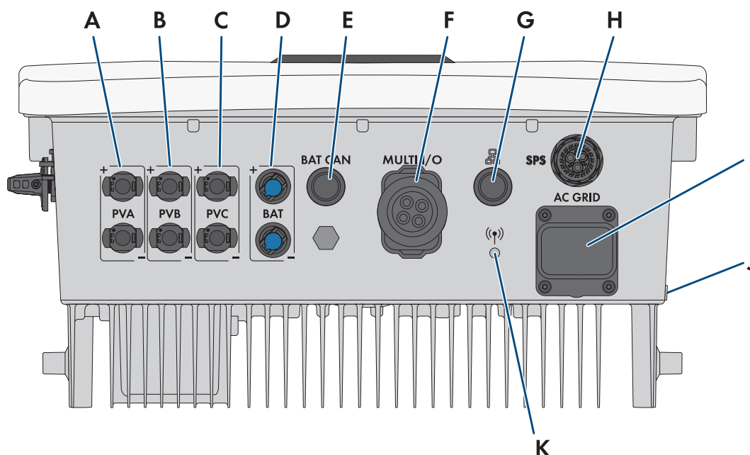
Figure 7 : Vue de dessous de l'onduleur
