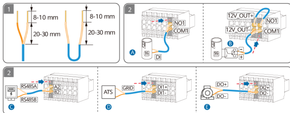
Figure 5-30 Connexion du câble de signal à la borne à 14 broches
