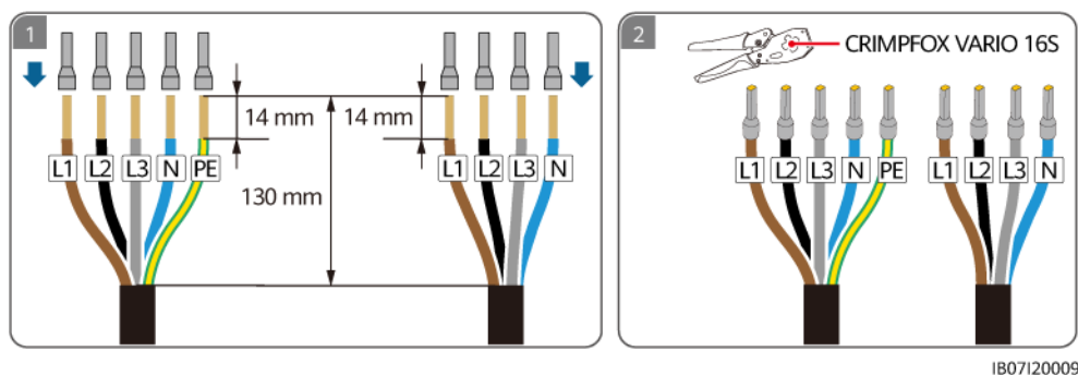
Figure 5-21 Sertissage des bornes d'extrémité du cordon CA
