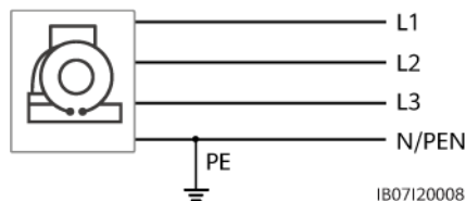
Figure 5-7 Mise à la terre des fils neutres du générateur
