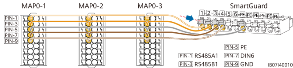
Figure 5-26 Connexion parallèle de câbles de signaux (en utilisant trois onduleurs connectés en parallèle à titre d'exemple)
