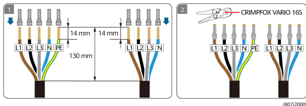
Figure 5-13 Sertissage des bornes d'extrémité du cordon CA
