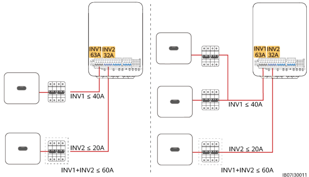
Figure 5-12 Onduleurs connectés en parallèle (les cases pointillées indiquent les composants facultatifs)
