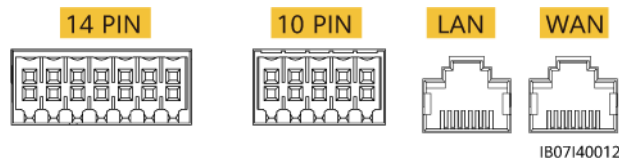
Figure 5-28 Définitions des ports
