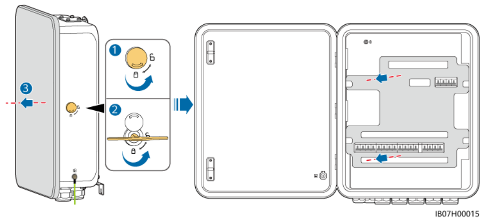
Figure 5-5 Ouverture de la porte du compartiment de maintenance
