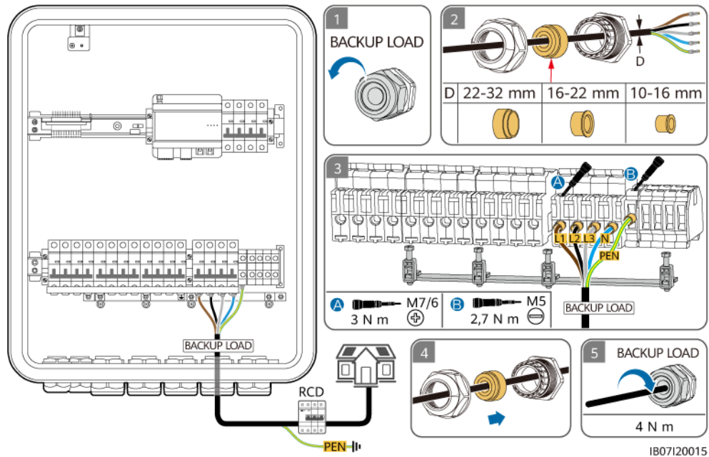
Figure 5-18 Connexion du câble d'alimentation de sortie de la charge de secours du SmartGuard-63A-T0 (système TN-S/TN-C-S/TT)
