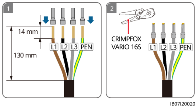
Figure 5-9 Sertissage des bornes d'extrémité du cordon CA (système TN-C)
