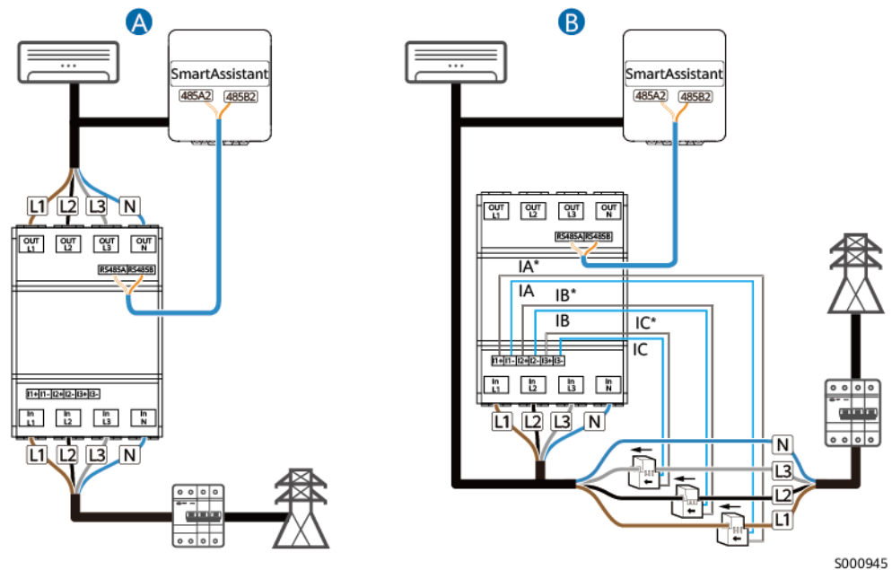
Figure 5-31 Connexion du câble de communication du compteur électrique
