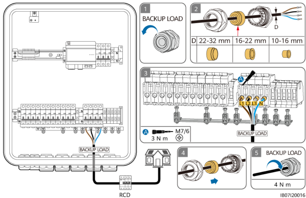
Figure 5-19 Connexion du câble d'alimentation de sortie de la charge de secours du SmartGuard-63A-AUTO (système TN-S/TN-C-S/TT)
