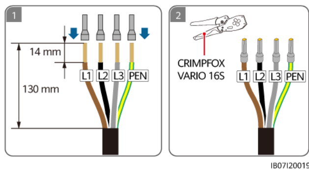
Figure 5-17 Sertissage des bornes d'extrémité du cordon CA (système TN-C)
