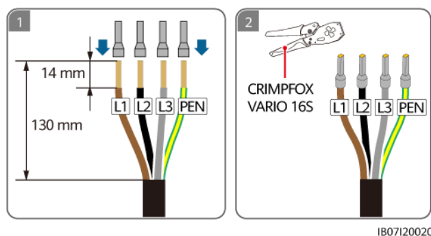
Figure 5-22 Sertissage des bornes d'extrémité du cordon CA (système TN-C)
