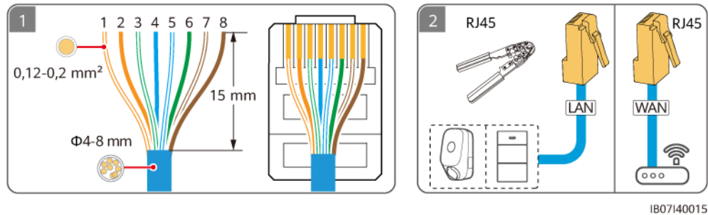
Figure 5-32 Câble de communication FE (les cases en pointillés indiquent les composants en option)
