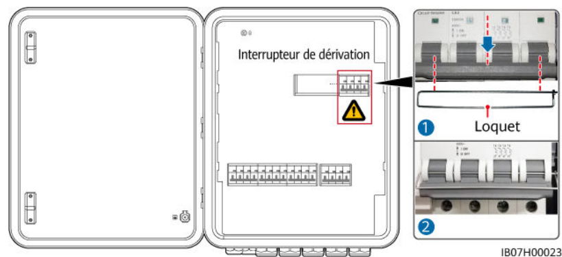
Figure 6-5 Désactivation du commutateur de dérivation
