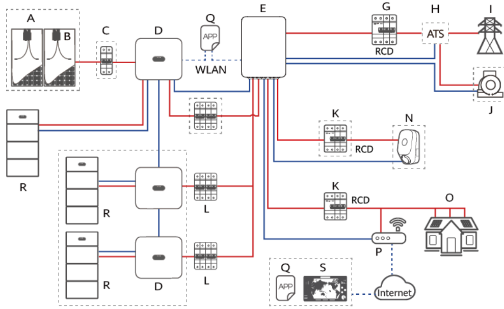
Figure 2-5 Mise en réseau avec toutes les charges connectées au SmartGuard (composants optionnels indiqués par des cadres en pointillés)
