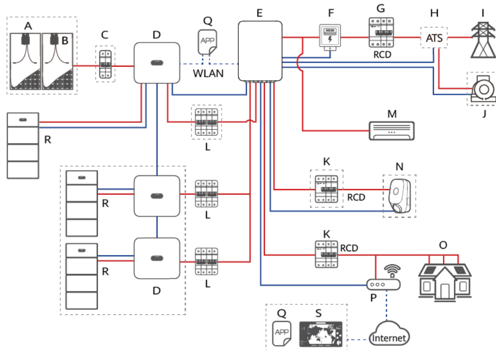
Figure 2-6 Mise en réseau avec certaines charges connectées au SmartGuard (composants optionnels indiqués par des cadres en pointillés)
