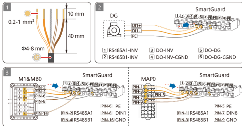
Figure 5-25 Sertissage des bornes d'extrémité de cordon pour le câble de signal (la case en pointillée indique un composant facultatif)
