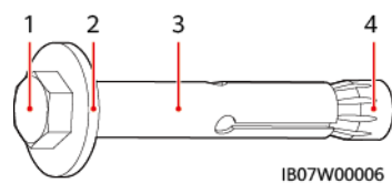
Figure 4-4 Composition d'un boulon à expansion
