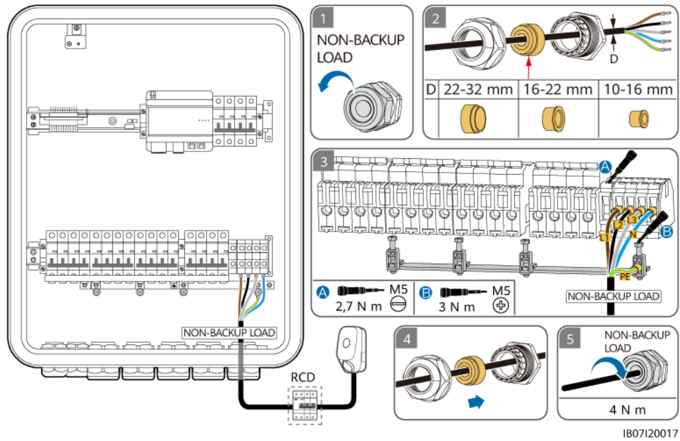
Figure 5-23 Connexion du câble d'alimentation de sortie de charge non de secours (système TN-S/TN-C-S/TT)
