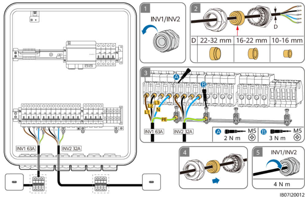
Figure 5-14 Branchement des câbles d'alimentation d'entrée CA de l'onduleur (cases en pointillés indiquant les composants facultatifs)
