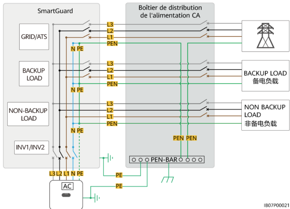
Figure 2-4 Schéma de câblage résidentiel pour le système TN-C (les lignes pointillées indiquent les connexions de câble facultatives)
