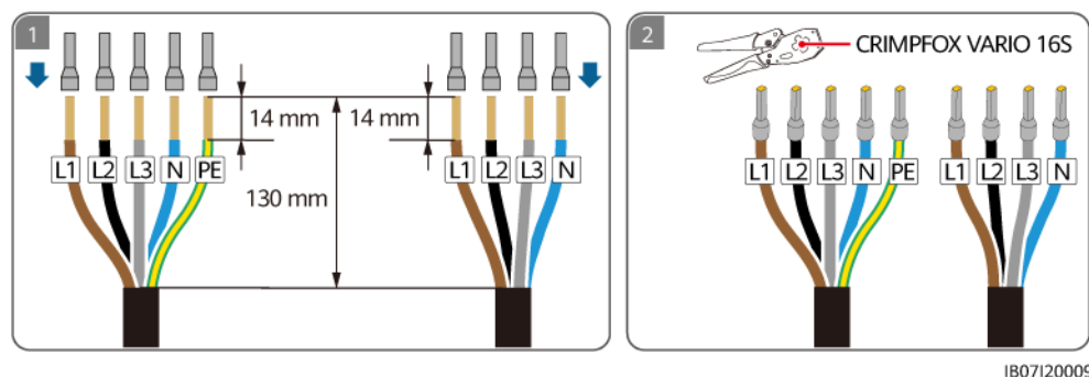
Figure 5-8 Sertissage des bornes d'extrémité du cordon CA (système TN-S/TN-C-S/TT)
