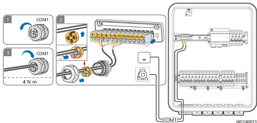
Figure 5-27 Connexion des câbles de signaux du SmartGuard (la case en pointillée indique un composant facultatif)
