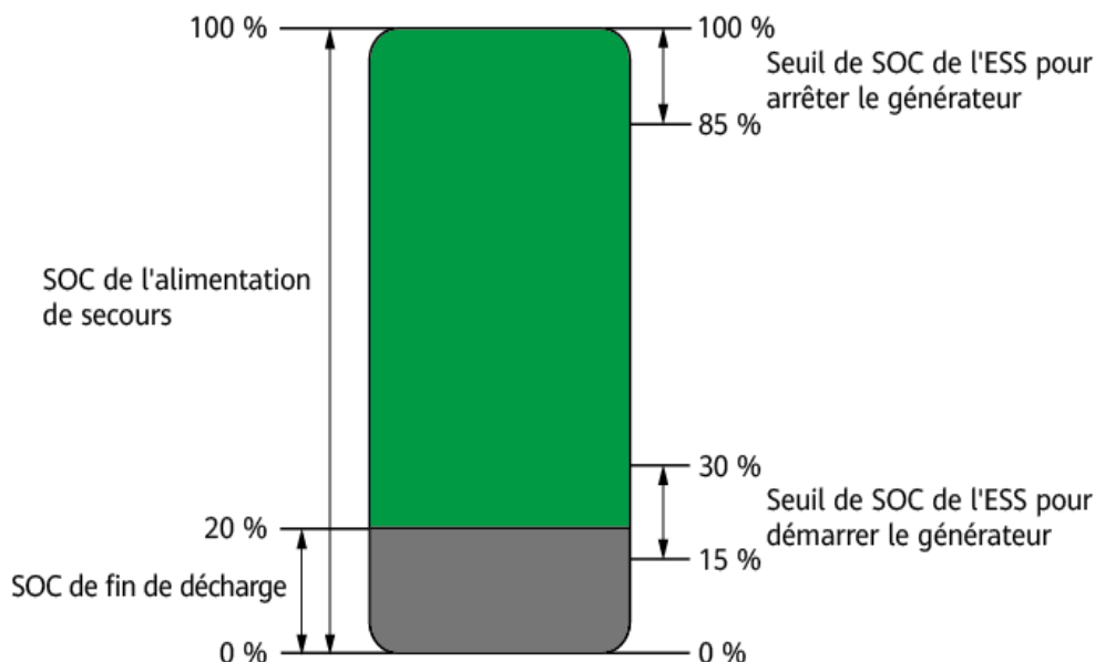
Figure 6-15 SOC Batterie
