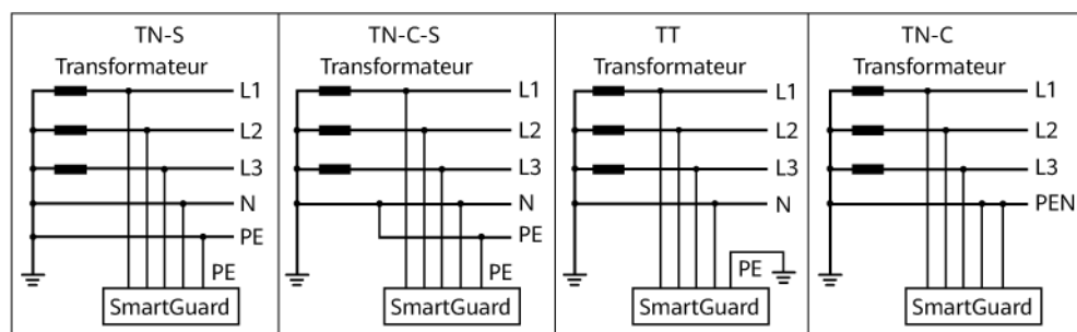
Figure 2-8 Systèmes de mise à la terre
