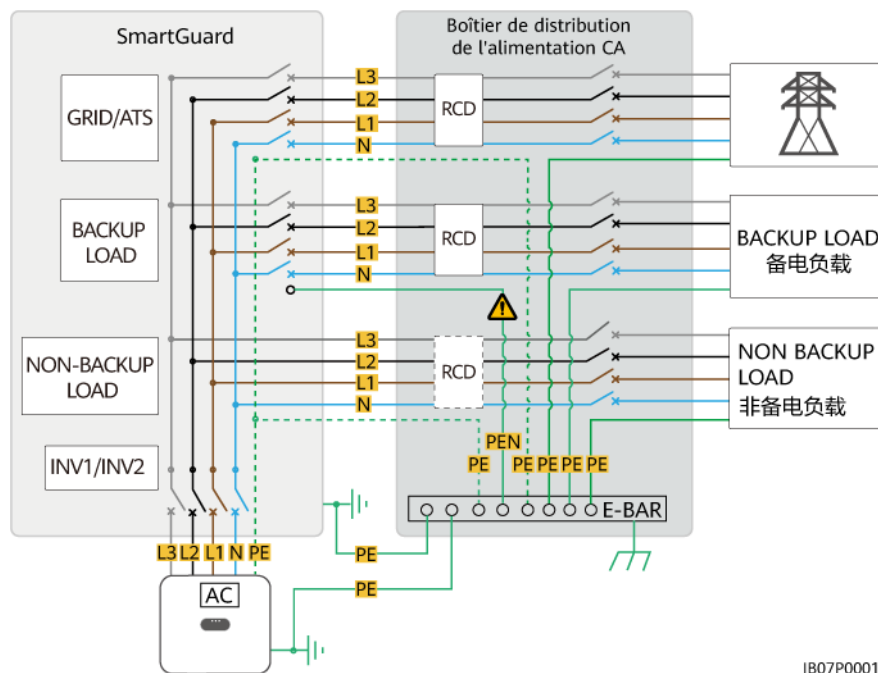
Figure 2-2 Schéma de câblage résidentiel du SmartGuard-63A-T0 (les lignes en pointillé indiquent les connexions de câbles en option)
