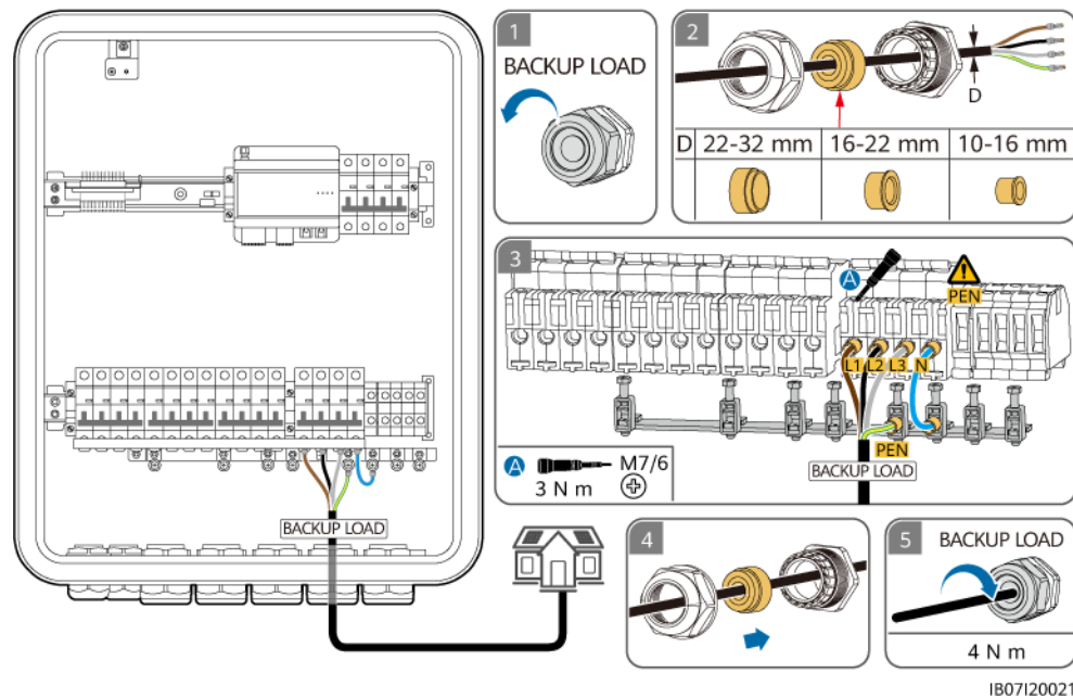
Figure 5-20 Connexion du câble d'alimentation de sortie de la charge de secours (système TN-C)
