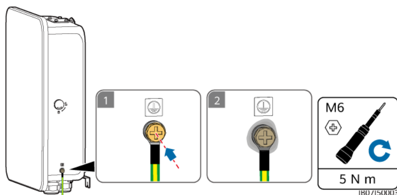
Figure 5-4 Connexion du câble PE
