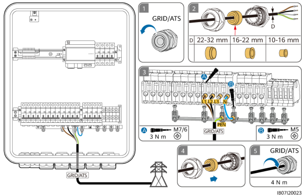
Figure 5-11 Connexion du câble d'alimentation de sortie CA du réseau (système TN-C)
