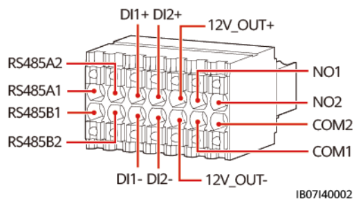
Figure 5-29 Définitions des broches
