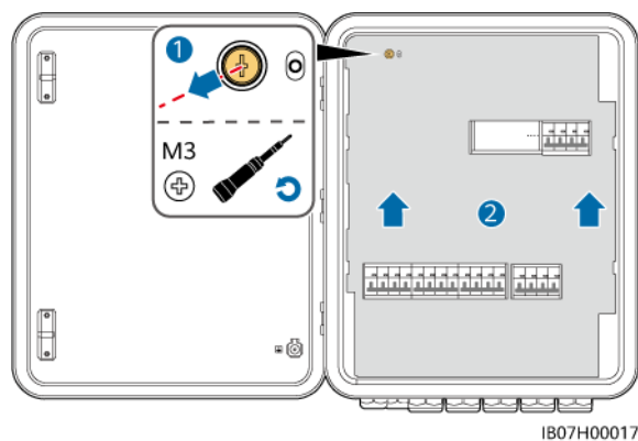
Figure 5-6 Ouverture du couvercle du compartiment de maintenance
