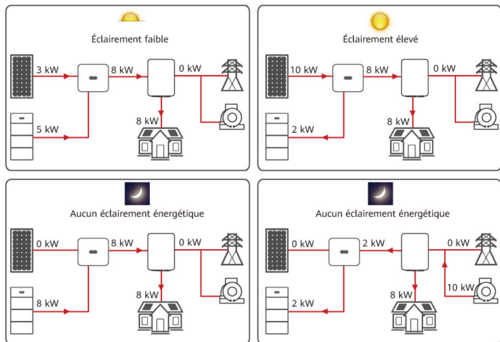
Figure 2-7 Illustration de la puissance maximale en mode hors réseau
