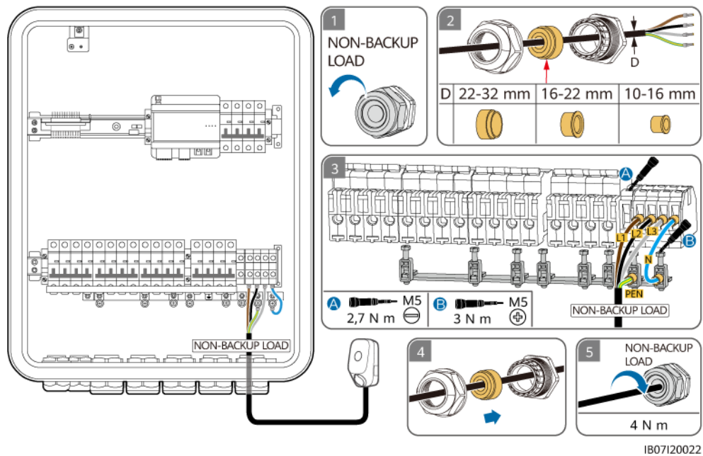
Figure 5-24 Connexion du câble d'alimentation de sortie de charge non de secours (système TN-C)
