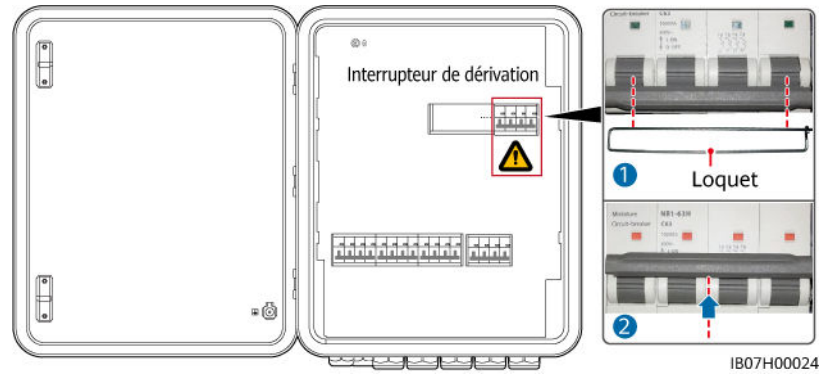
Figure 6-2 Activation du commutateur de dérivation
