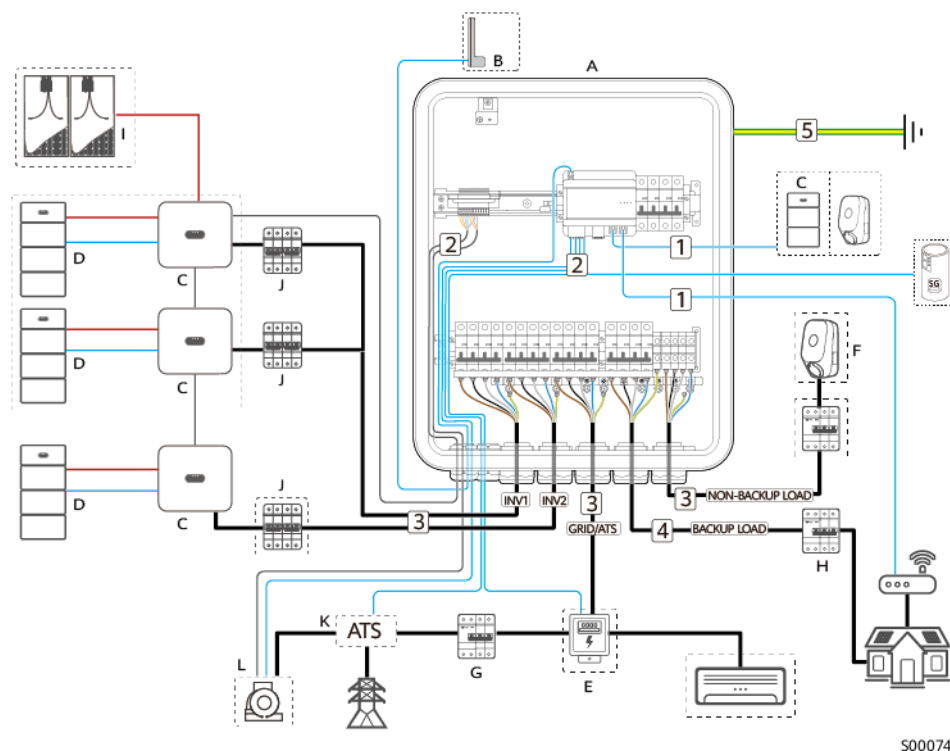
Figure 5-1 Connexions des câbles (les cases en pointillés indiquent des configurations facultatives)
