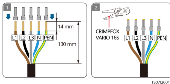
Figure 5-15 Sertissage des bornes d'extrémité du cordon CA pour le SmartGuard-63A-T0 (système TN-S/TN-C-S/TT)
