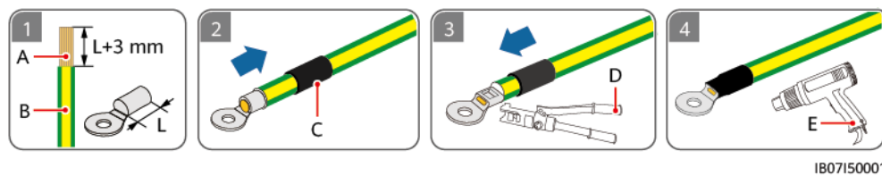
Figure 5-3 Sertissage d'une borne OT
