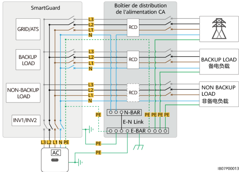
Figure 2-3 Schéma de câblage résidentiel du SmartGuard-63A-AUT0 (les lignes en pointillé indiquent les connexions de câbles en option)
