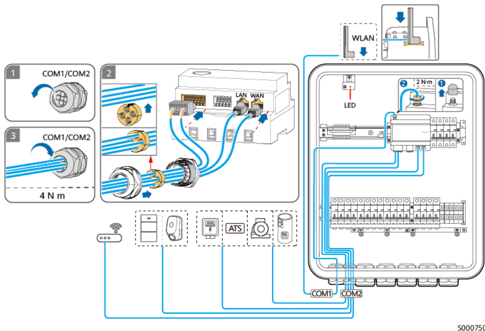
Figure 5-33 Connexion des câbles de signal SmartAssistant (les cases en pointillés indiquent les composants facultatifs)
