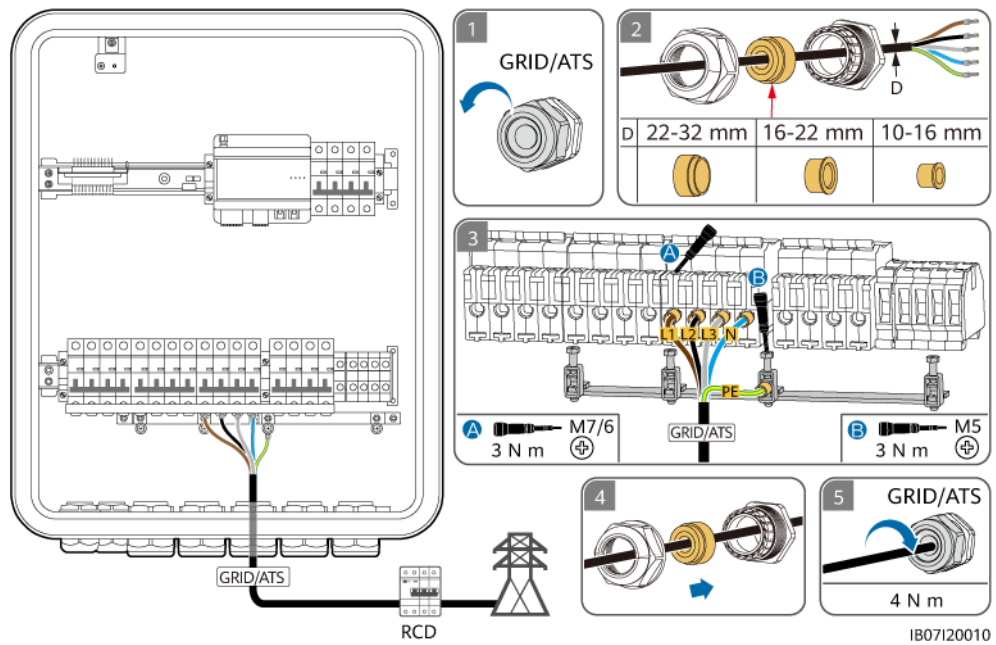
Figure 5-10 Connexion du câble d'alimentation de sortie CA du réseau (système TN-S/TN-C-S/TT)
