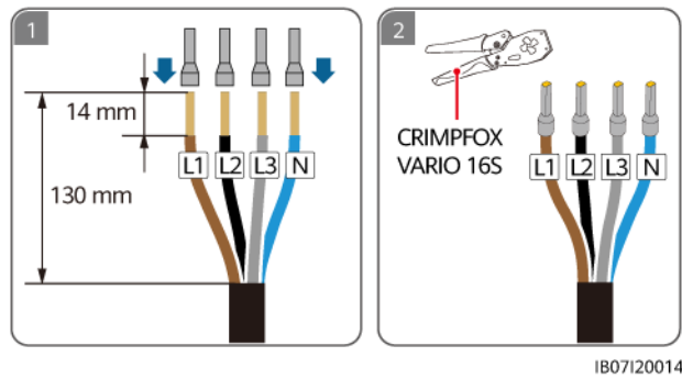
Figure 5-16 Sertissage des bornes d'extrémité du cordon CA pour le SmartGuard-63A-AUTO (système TN-S/TN-C-S/TT)
