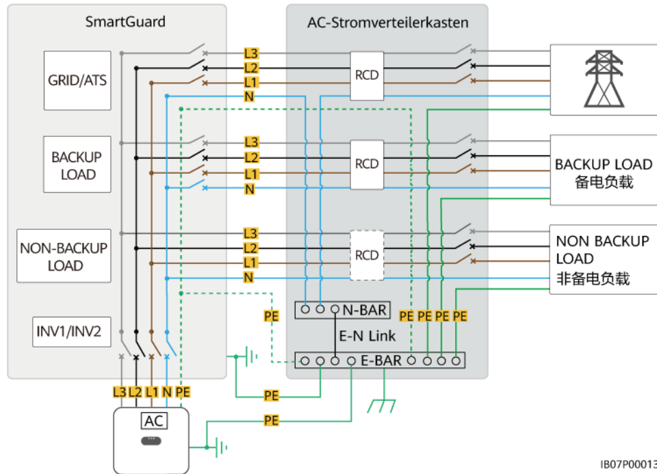
Abbildung 2-3 SmartGuard-63A-AUT0-Schaltplan für Eigenheime (gestrichelte Linien zeigen optionale Kabelverbindungen an)
