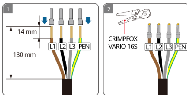
Abbildung 5-9 Crimpen der AC-Kabelndklemmen (TN-C-System)
