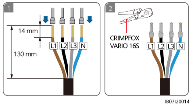
Abbildung 5-16 Crimpen der AC-Kabelendklemmen für den SmartGuard-63A-AUT0 (TN-S/TN-C-S/TT-System)
