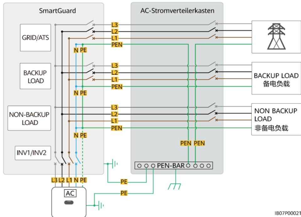
Abbildung 2-4 Schaltpläne für Eigenheime für das TN-C-System (gestrichelte Linien zeigen optionale Kabelverbindungen an)
