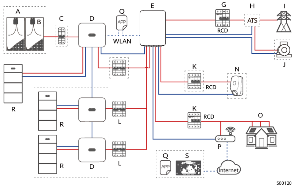
Abbildung 2-5 Vernetzung aller Lasten, die an die SmartGuard angeschlossen sind (gestrichelte Kästchen weisen auf optionale Komponenten hin)
