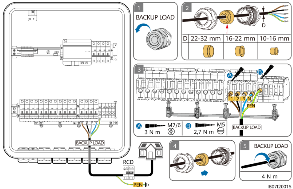
Abbildung 5-18 Anschließen des Ausgangstromkabels der Backup-Last vom SmartGuard-63A-T0 (TN-S/TN-C-S/TT-System)
