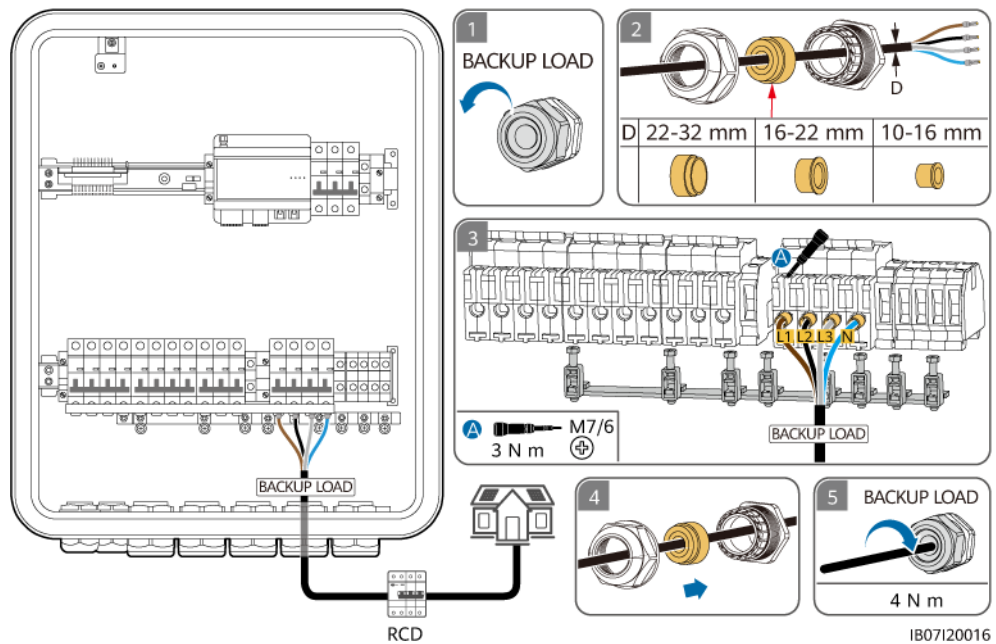
Abbildung 5-19 Anschließen des Ausgangstromkabels der Backup-Last vom SmartGuard-63A-AUTO (TN-S/TN-C-S/TT-System)
