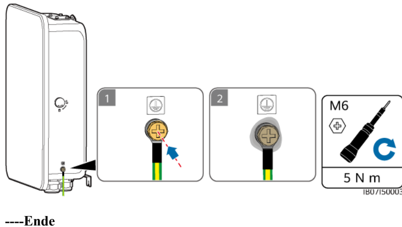
Abbildung 5-4 Anschließen des PE-Kabels
