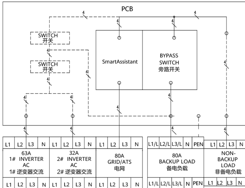
Abbildung 2-11 Elektrischer Schaltplan der SmartGuard
