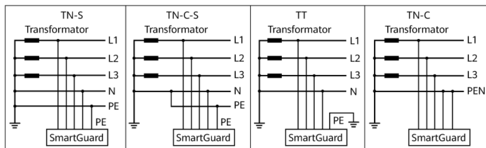
Abbildung 2-8 Erdungssysteme
