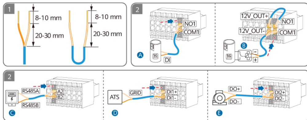
Abbildung 5-30 Anschluss des Signalkabels an die 14-polige Klemme
