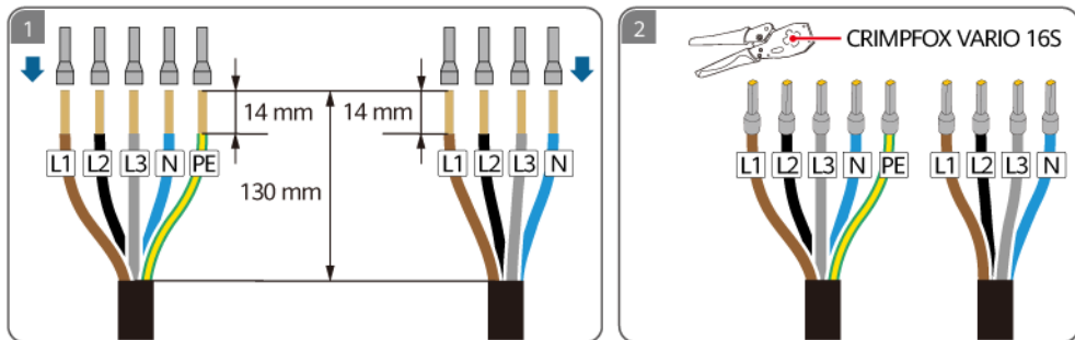
Abbildung 5-8 Crimpen der AC-Kabelndklemmen (TN-S/TN-C-S/TT-System)
