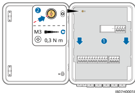
Abbildung 6-1 Abdeckungen schließen
