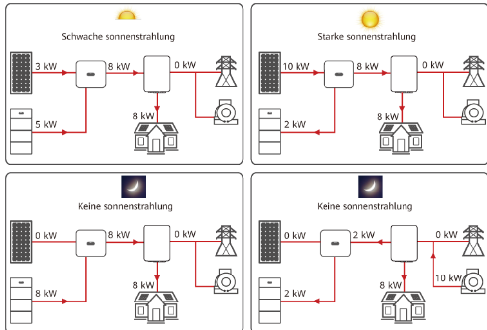
Abbildung 2-7 Darstellung der maximalen Leistung im netzentkoppelten Modus
