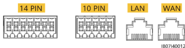
Abbildung 5-28 Anschlussdefinitionen
