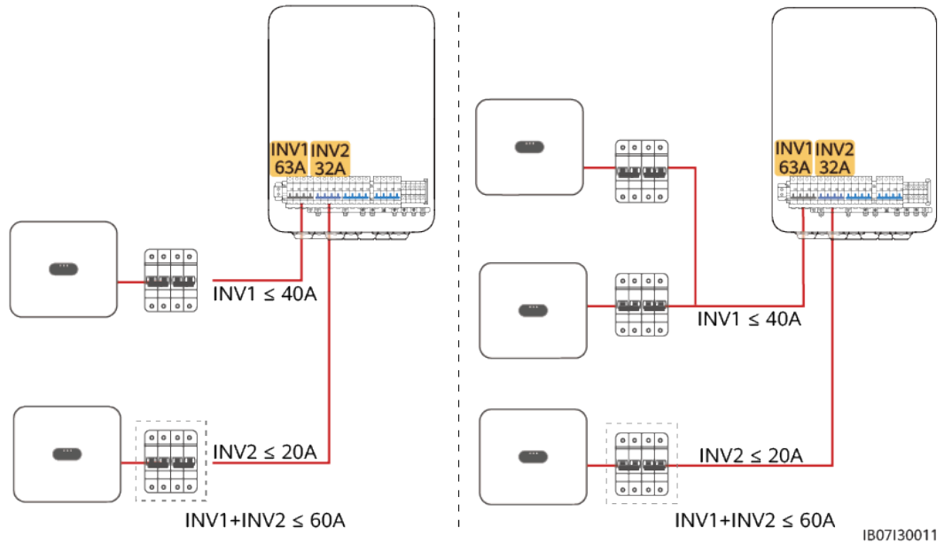
Abbildung 5-12 Parallel geschaltete Wechselrichter (gestrichelte Kästchen weisen auf optionale Komponenten hin)
