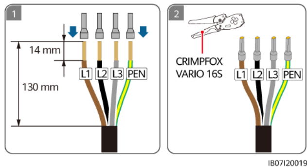
Abbildung 5-17 Crimpen der AC-Kabelendklemmen (TN-C-System)
