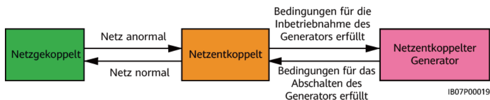
Abbildung 2-12 Arbeitsmodi
